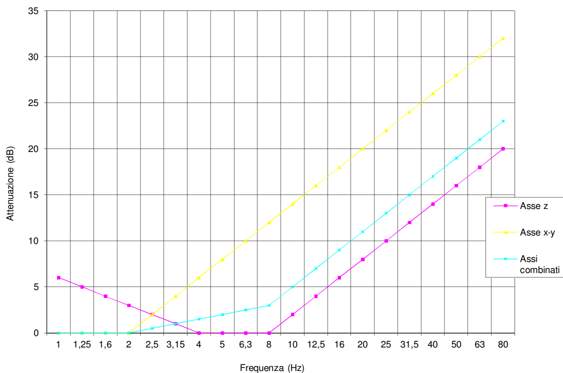
Figura 3-2 Filtri di ponderazione (UNI 9614)
