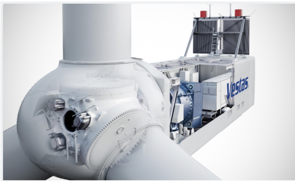
Figura 7 - Spaccato aerogeneratore tipo, modello V162
