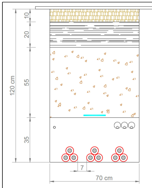
Figura 12 – Sezione tipo del cavidotto interrato MT composto da n.3 terne di cavi su strada asfaltata
