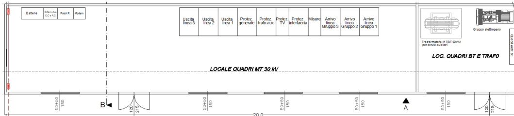
Figura 8 – Pianta della cabina di raccolta
