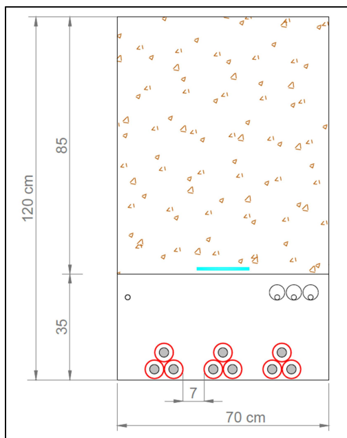
Figura 14 – Sezione tipo del cavidotto interrato MT composto da n.3 terne di cavi su terreno
