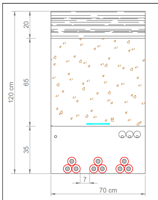
Figura 13 – Sezione tipo del cavidotto interrato MT composto da n.3 terne di cavi su strada sterrata
