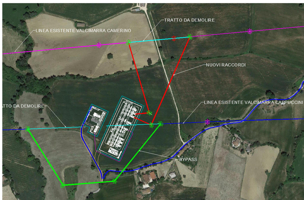
Figura 20 – Stralcio su ortofoto della posizione della SEU, del cavidotto in AT (in ciano), della Stazione SE e di raccordi (in rosso)
