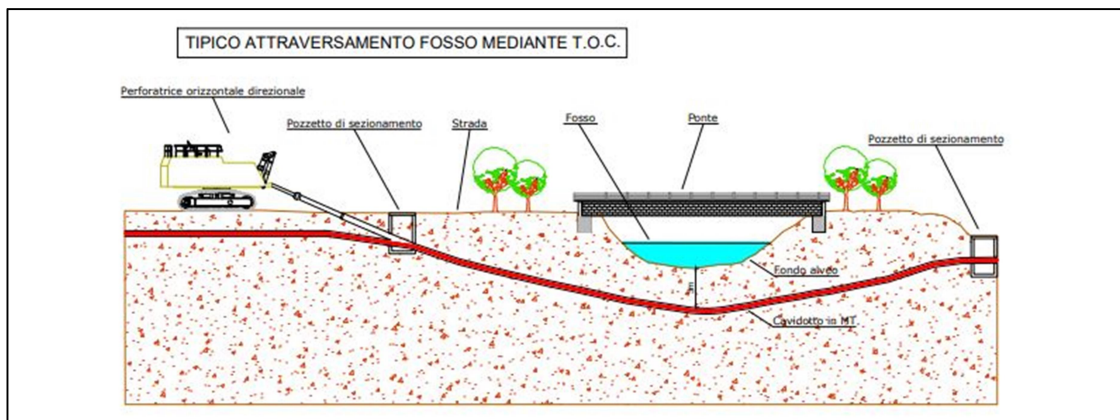
Figura 15 - Attraversamento tipo mediante tecnica TOC dei fossi
