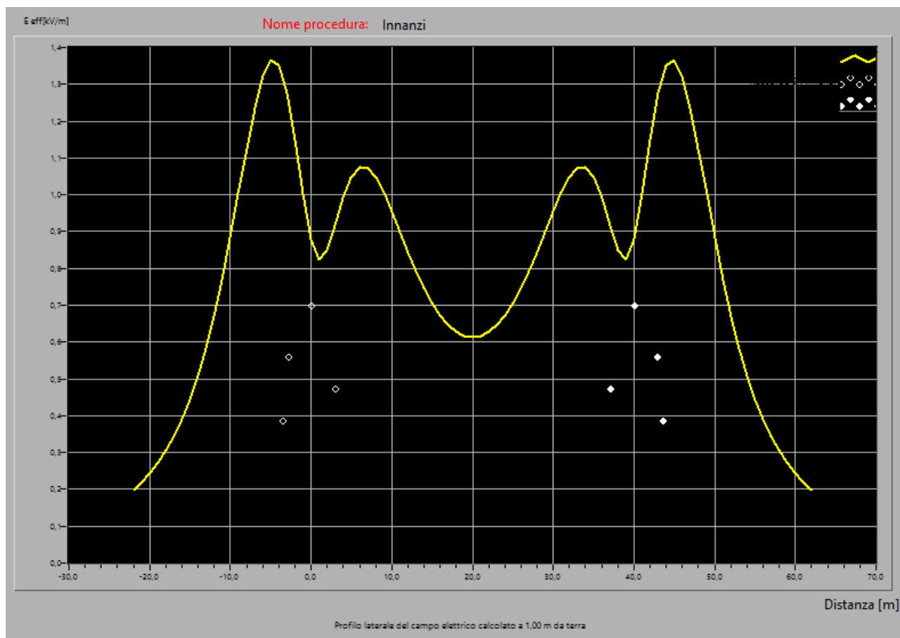
Profilo laterale del campo elettrico a 1 m dal suolo generato dai 2 elettrodoti paralleli
