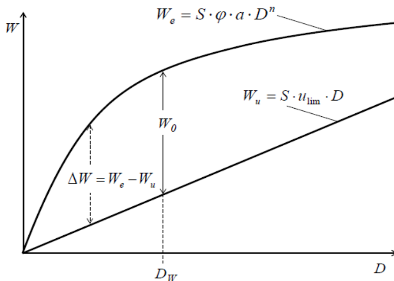
Figura 5 Individuazione con il metodo delle sole piogge dell'evento critico D_w e del corrispondente volume critico W_0 di laminazione, ovvero quello che massimizza il volume invasato.
