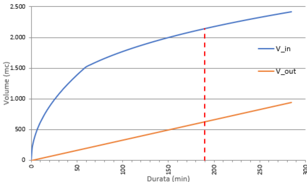
Figura 7 Determinazione dell'evento critico D_w e del corrispondente volume critico W_0 di laminazione – vasca di laminazione V2
