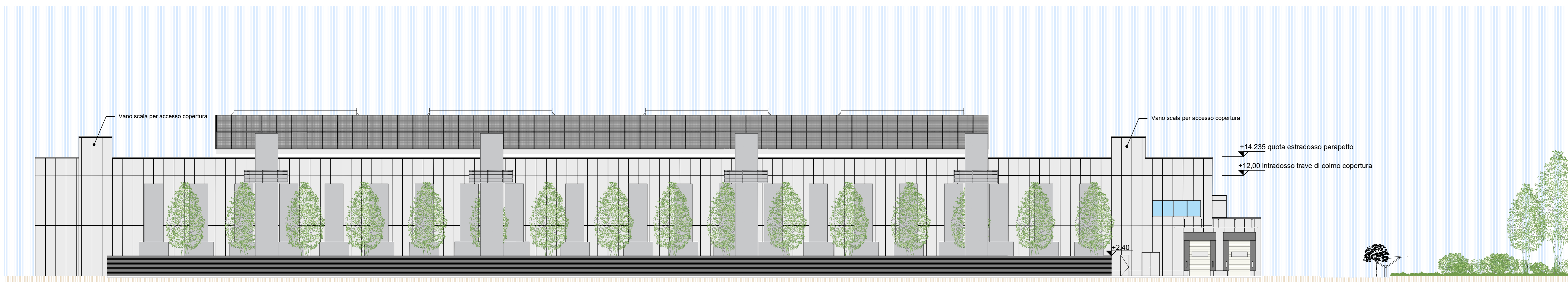
PROSPETTO 6-6'
