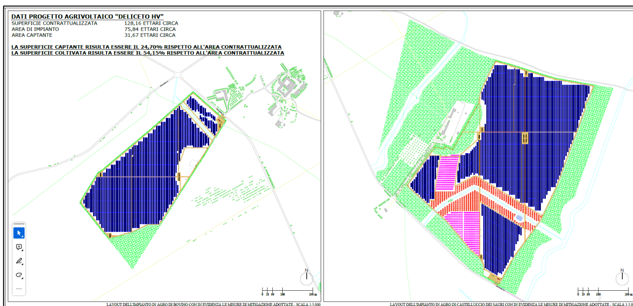
Fig. 3 - Estratto dall'elaborato grafico 23: layout impianto, opere di mitigazione, superfici
