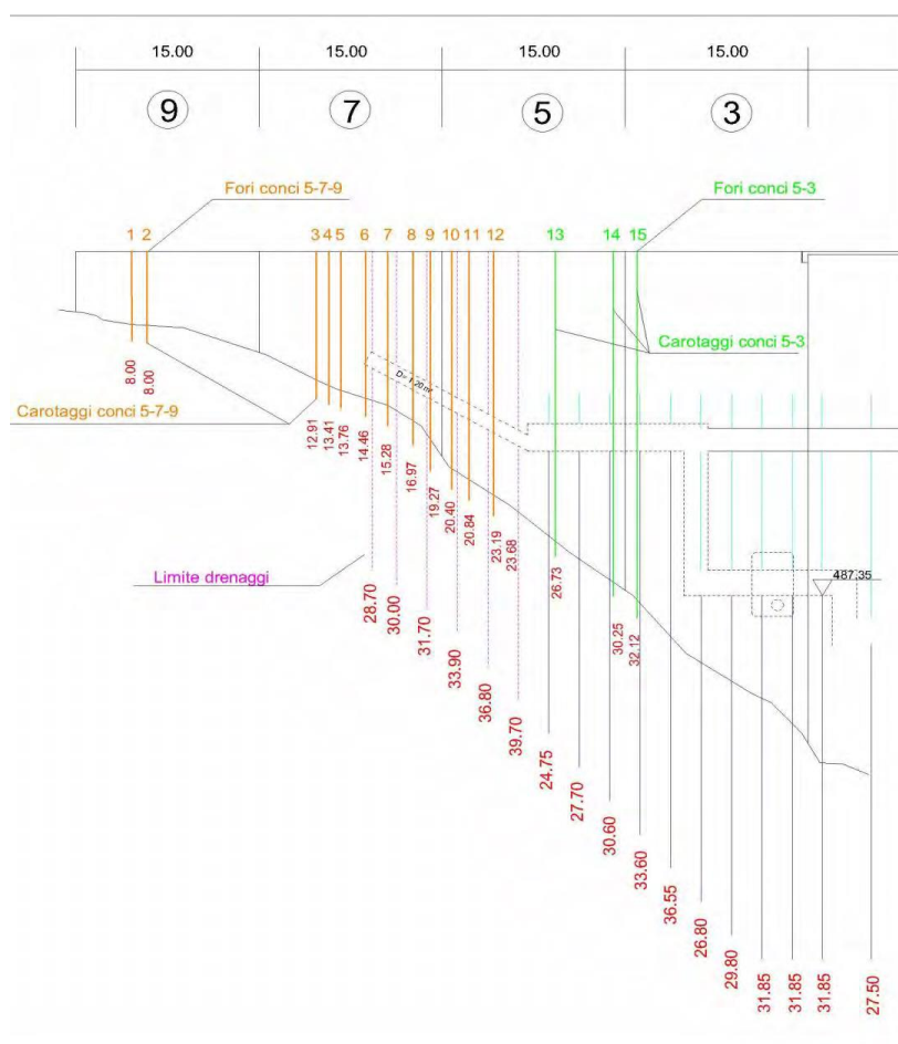
Figura 9 Posizionamento perforazioni a carotaggio nei concii 5-3 indagini Ottobre 2010
