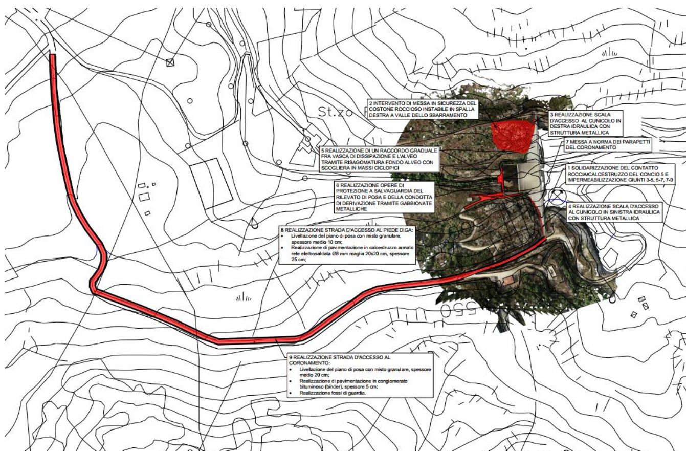
Figura 21 Planimetria riassuntiva degli interventi
