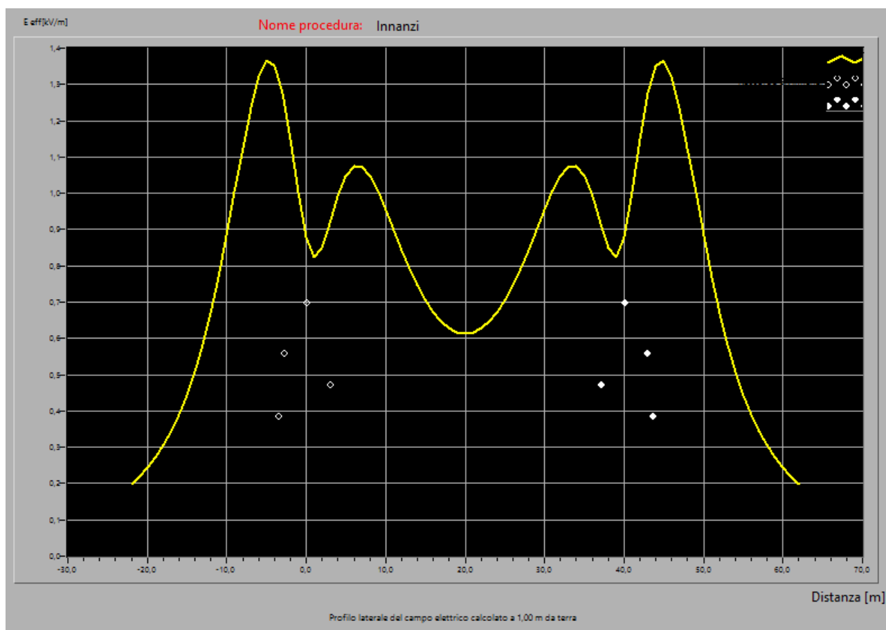
Profilo laterale del campo elettrico a 1 m dal suolo generato dai 2 elettrodotto paralleli
