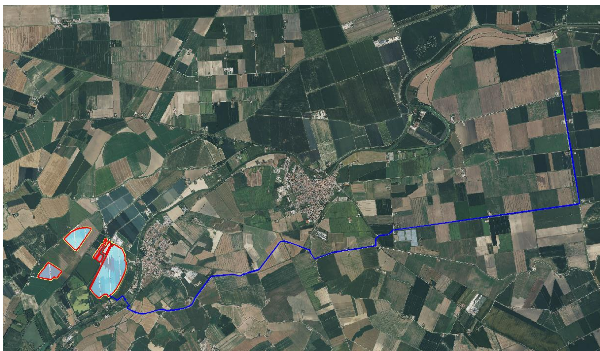
Figura 1 Ubicazione di impianto con connessione alla SSE.
