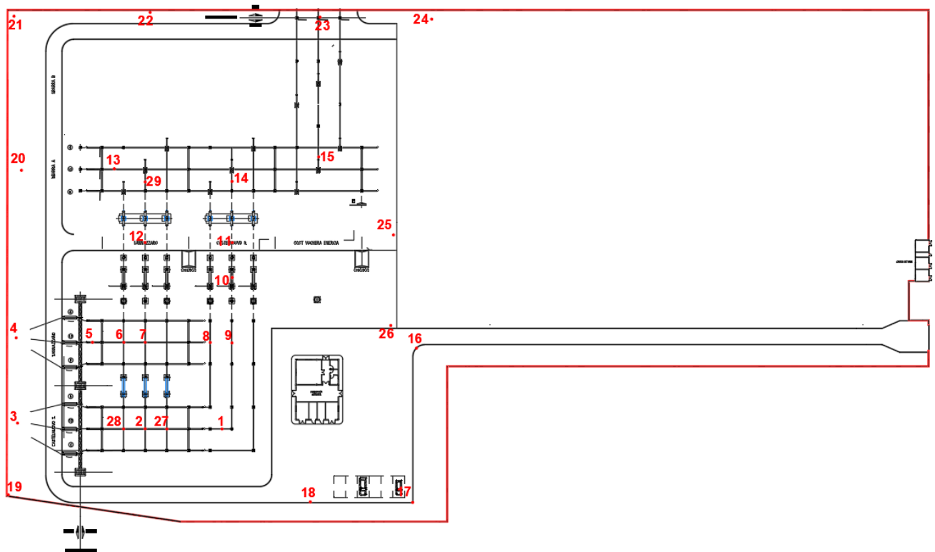
Figura 3 – Planimetrica della stazione 380 kV Voghera esistente
