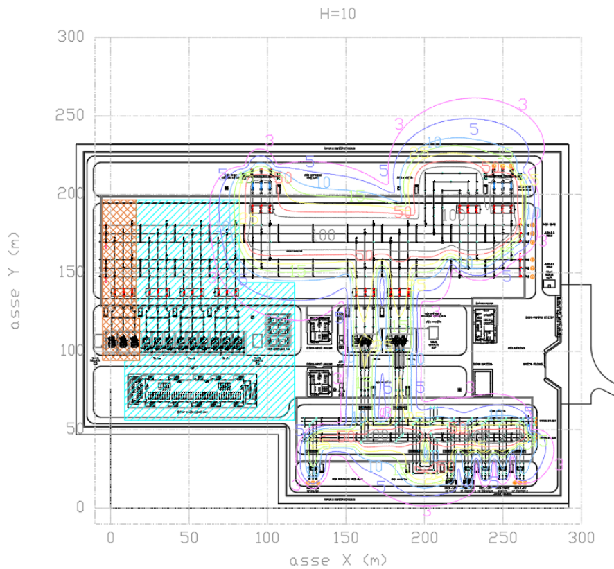
Figura 8 – Livelli di campo magnetico a 10 m dal piano della stazione
