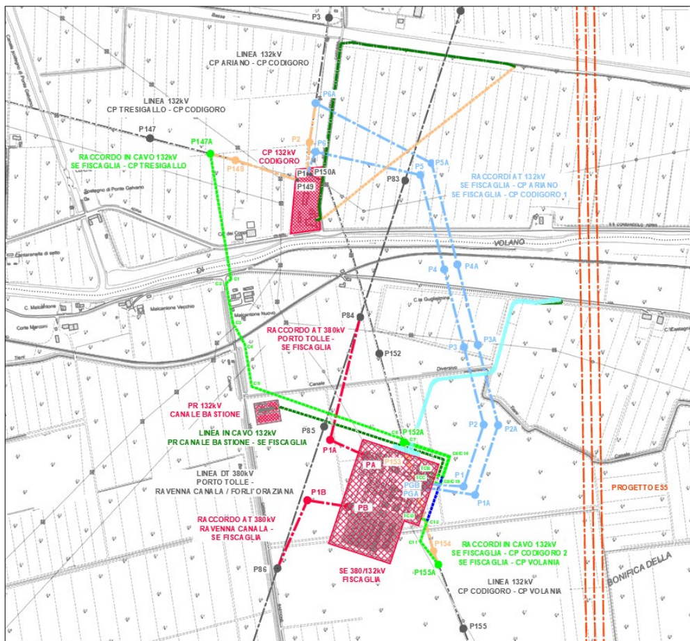
Figura 1: Planimetria delle opere in progetto
