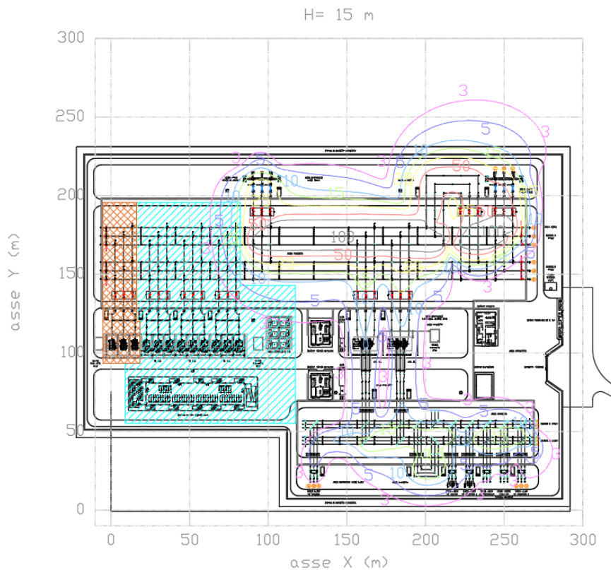
Figura 9 – Livelli di campo magnetico a 15 m dal piano della stazione
