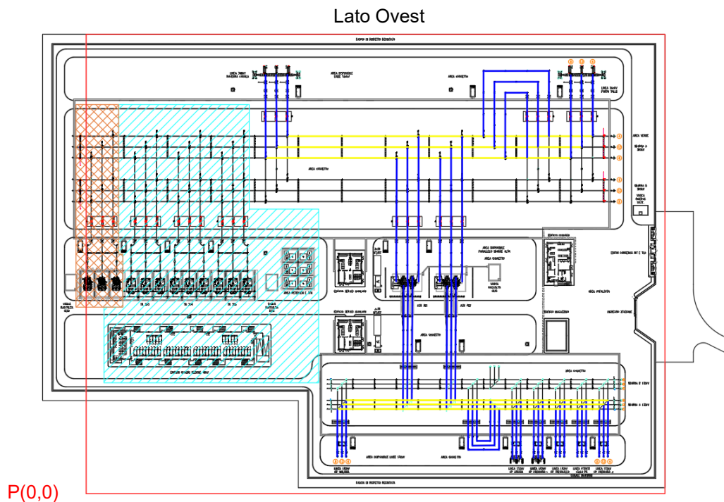
Figura 5 – Schematizzazione degli elementi attivi all'interno della planimetria
