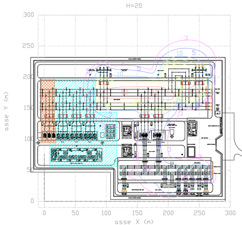
Calculations performed by software BE SHIELDING MAGIC Figura 10 – Livelli di campo magnetico a 20 m dal piano della stazione
