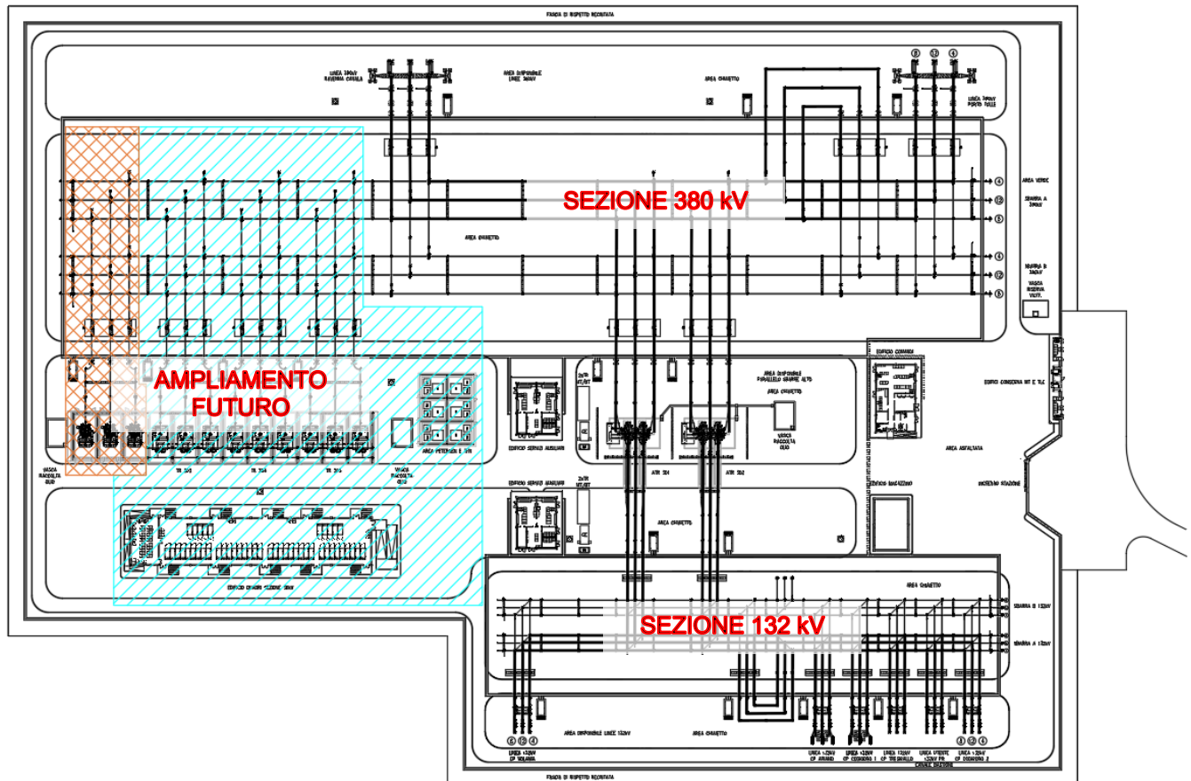
Figura 2: planimetria della stazione
