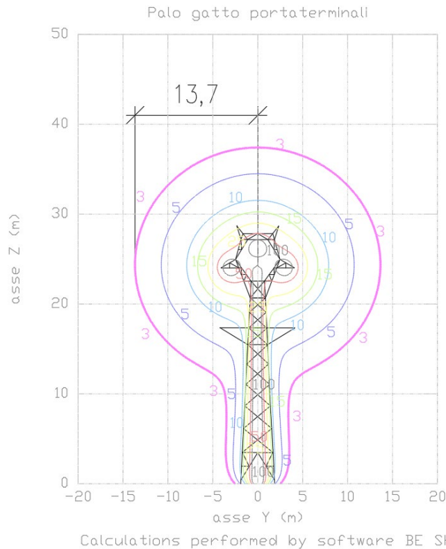
Figura 3 – Livelli di campo magnetico generato dai conduttori aerei e dal cavo come disposti sul palo gatto di transizione
