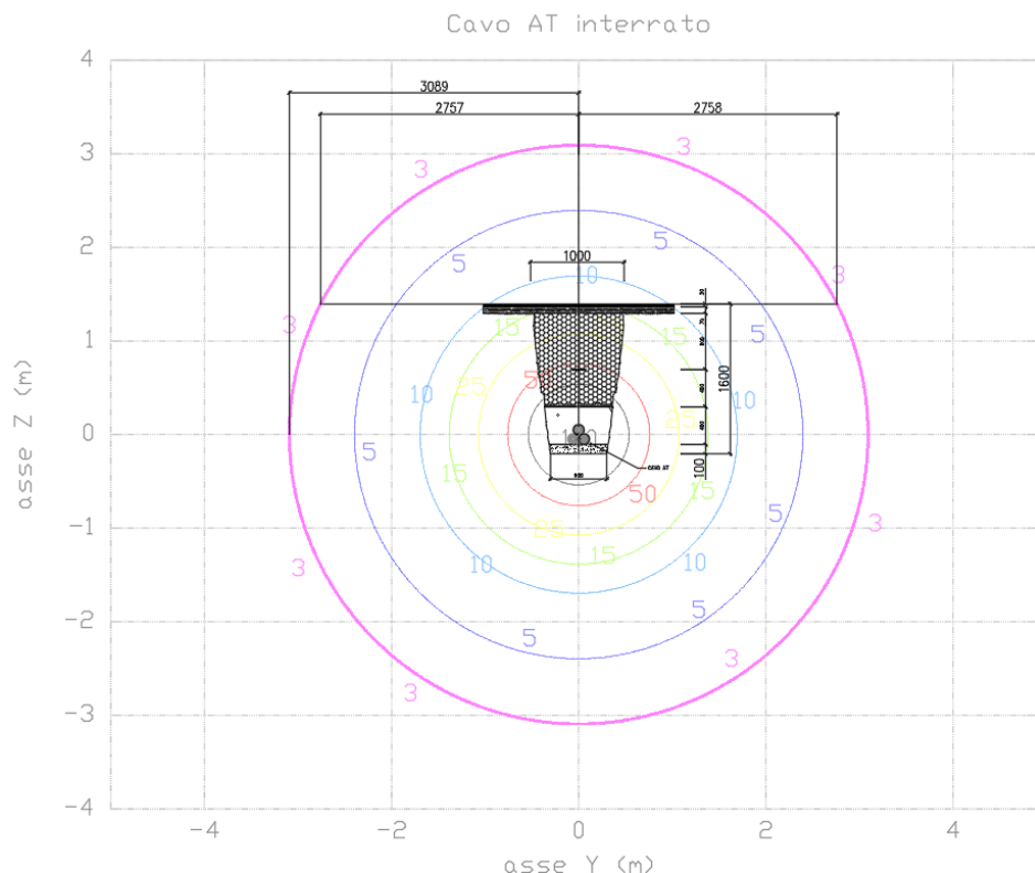
Figura 2 – Livelli di campo magnetico generati dal cavo AT interrato posato a trifoglio
