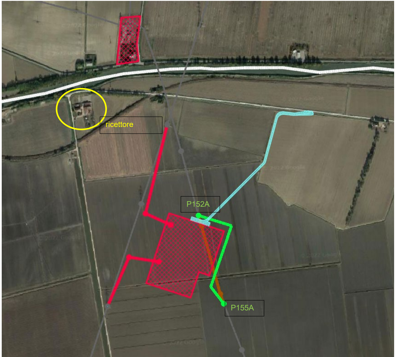
Figura 4 – Foto aerea con individuazione del ricettore sensibile e progetto dell'elettrodotto interrato a 132 kV
