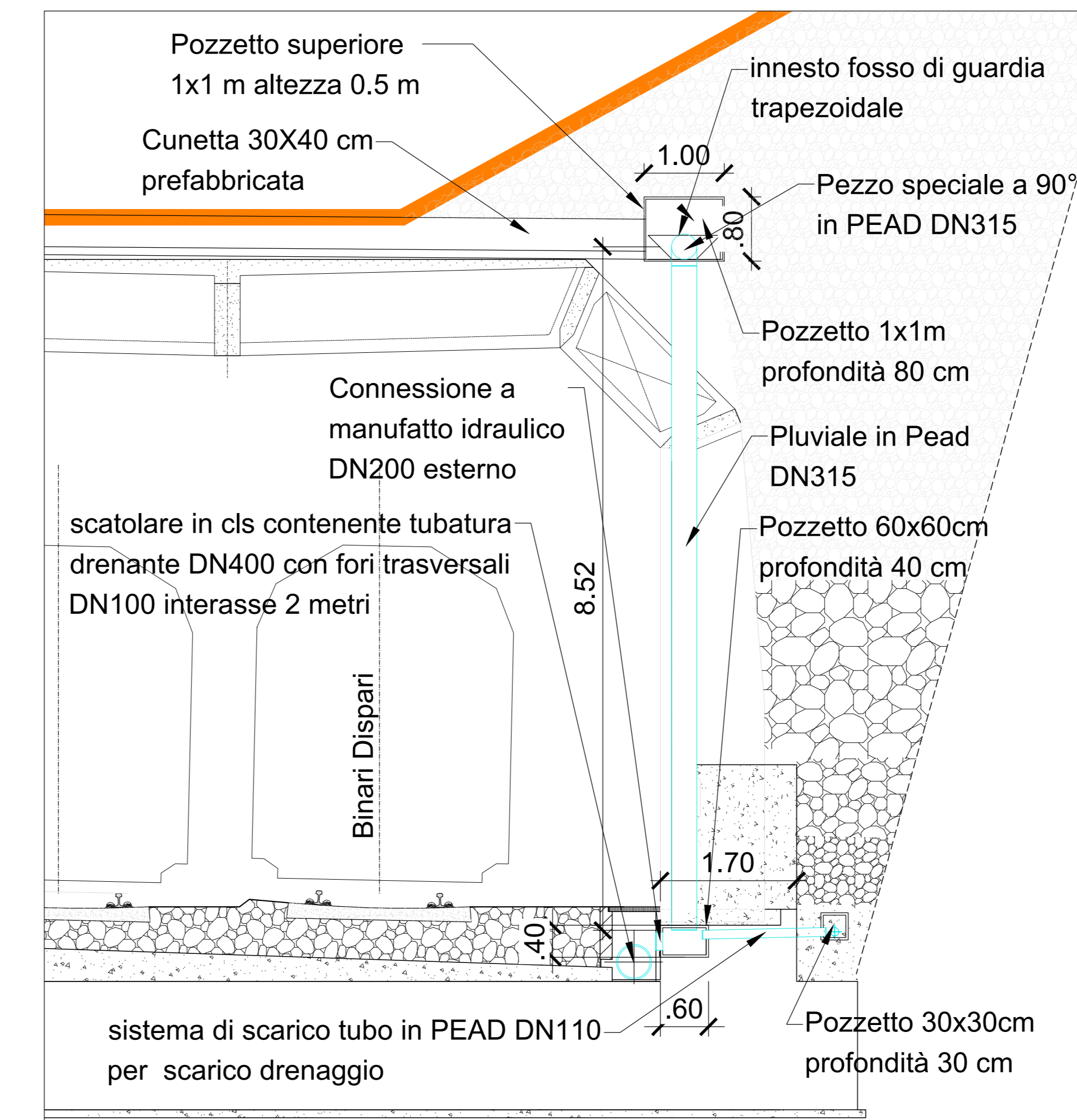
Opera Idraulica 2 1:20 sezione trasversale al tracciato ferroviario
