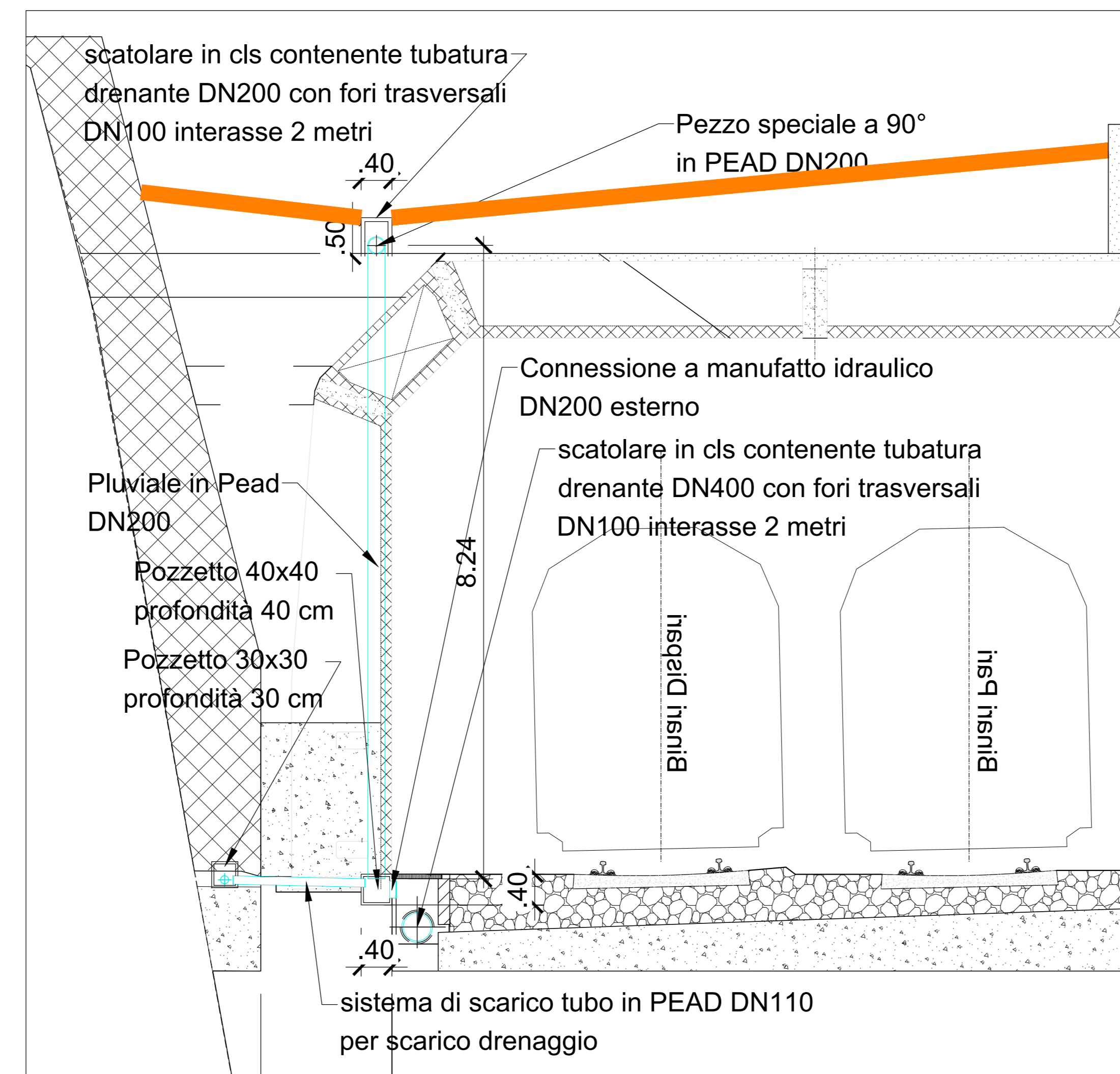
Opera Idraulica 1 1:20 sezione trasversale al tracciato ferroviario
