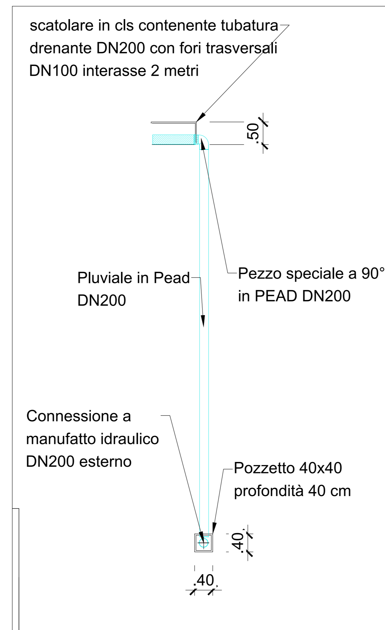
Opera Idraulica 1 1:20 sezione longitudinale al tracciato ferroviario
