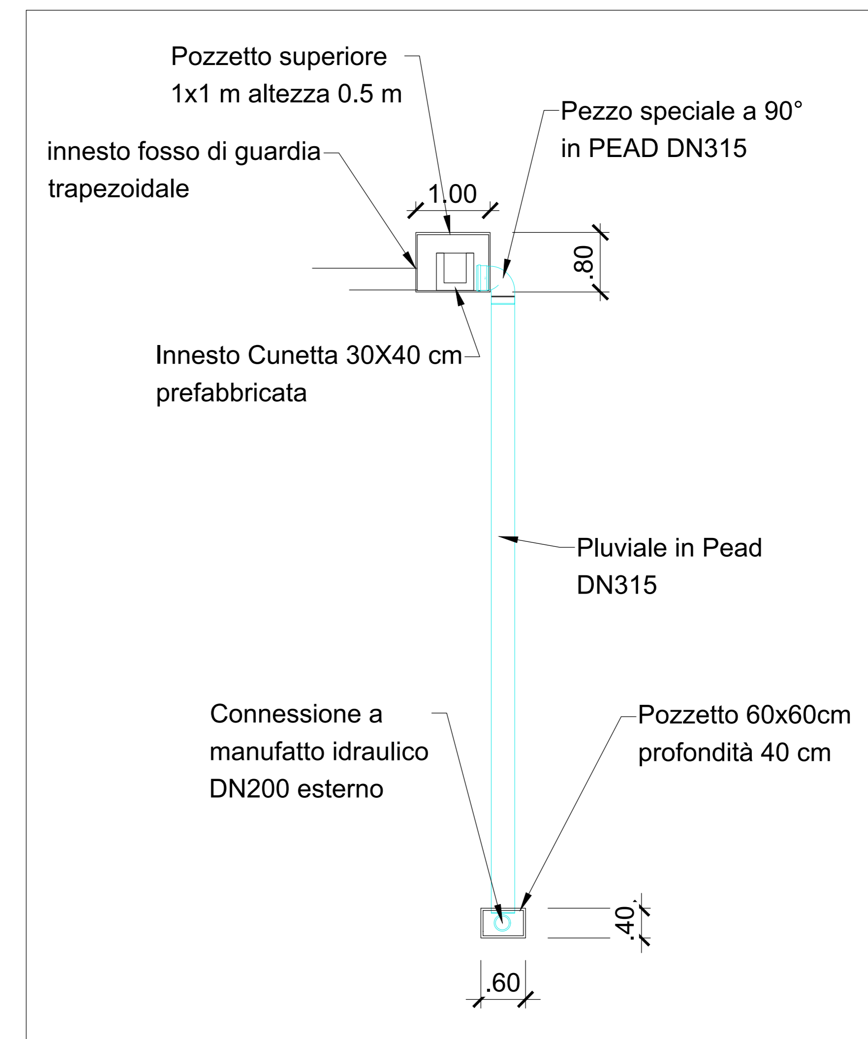
Opera Idraulica 2 1:20 sezione longitudinale al tracciato ferroviario
