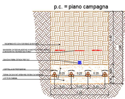
Fig. 26. Schemi della sezione di posa di elettrodotti MT 30 kV interrati con diverso numero di terre
