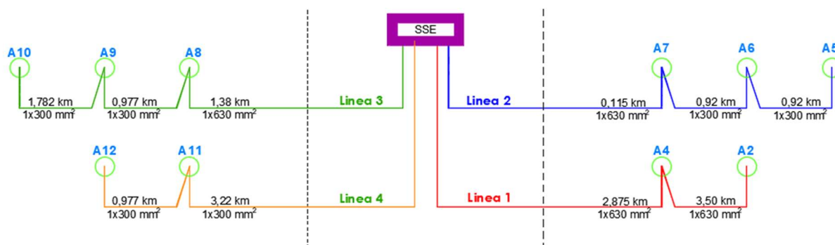
Fig. 27 Grafo a deformata della distribuzione elettrica MT 30kV
