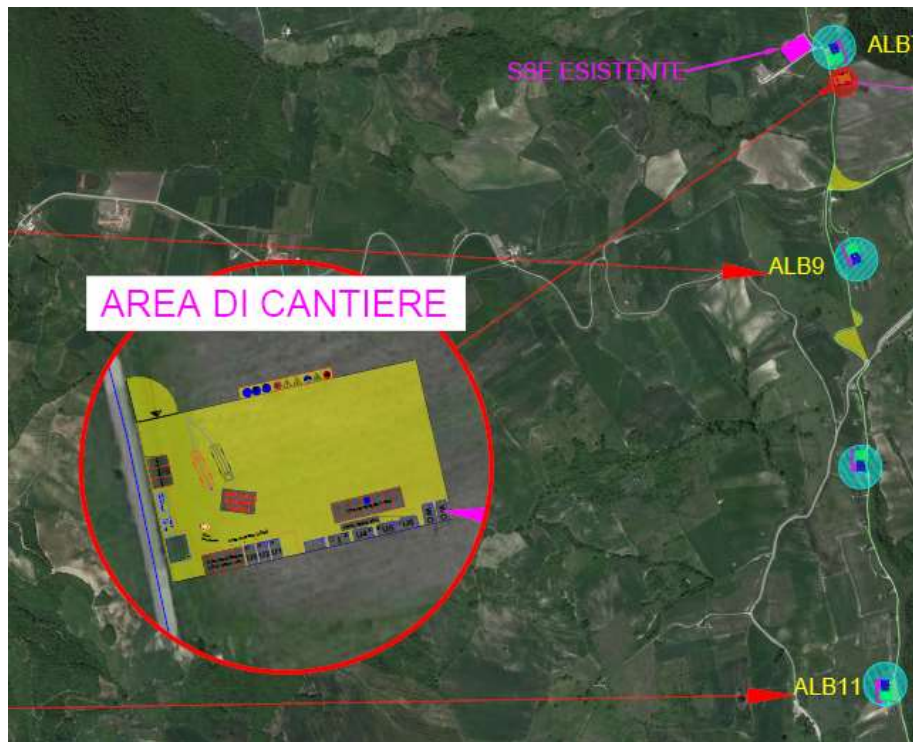
Fig. 19 Punto di ubicazione del Campo Base dell'Area di Cantiere e sua ubicazione rispetto alla sottostazione e agli aerogeneratori del nuovo parco eolico.
