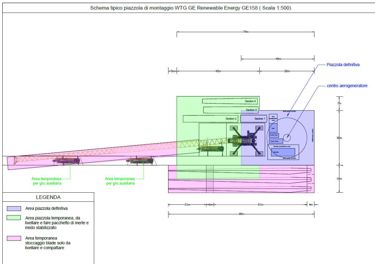
Fig. 10 Schema tipico della piazzola definitiva e di montaggio per il nuovo impianto.
