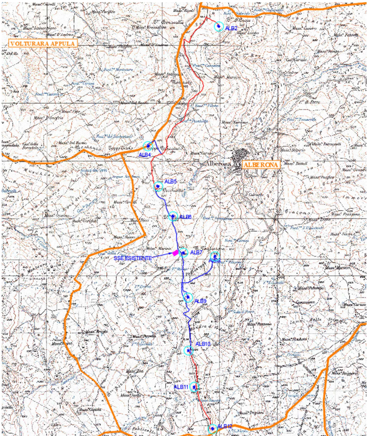
Fig. 5 Tracciato elettrodotti impianto esistente (colore blu) e dell'impianto di progetto (colore magenta)
