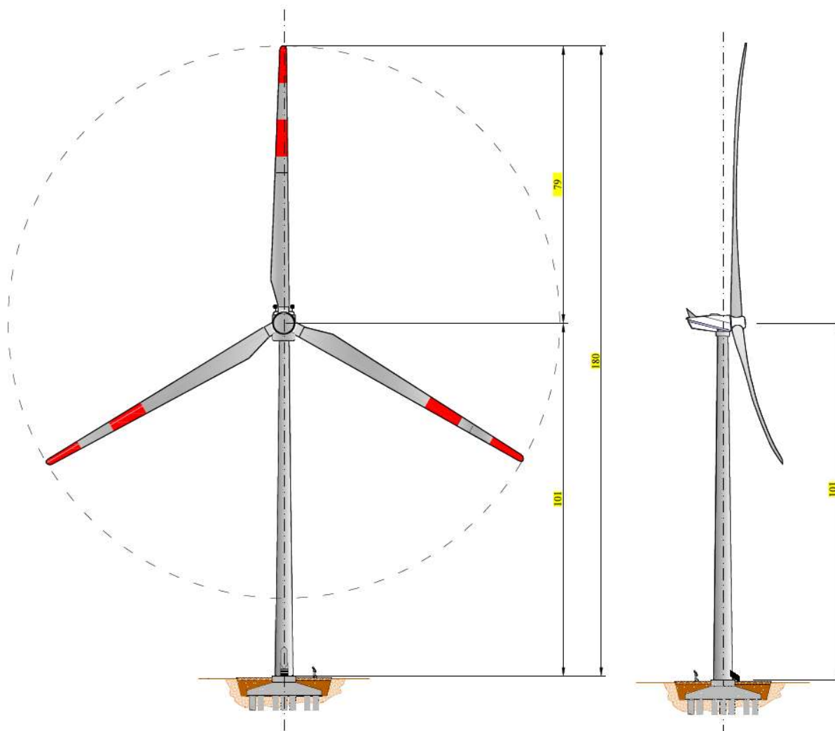
Fig. 11. Caratteristiche dimensionali: Prospetto aerogeneratore GE 158 da 6,1 MW.
