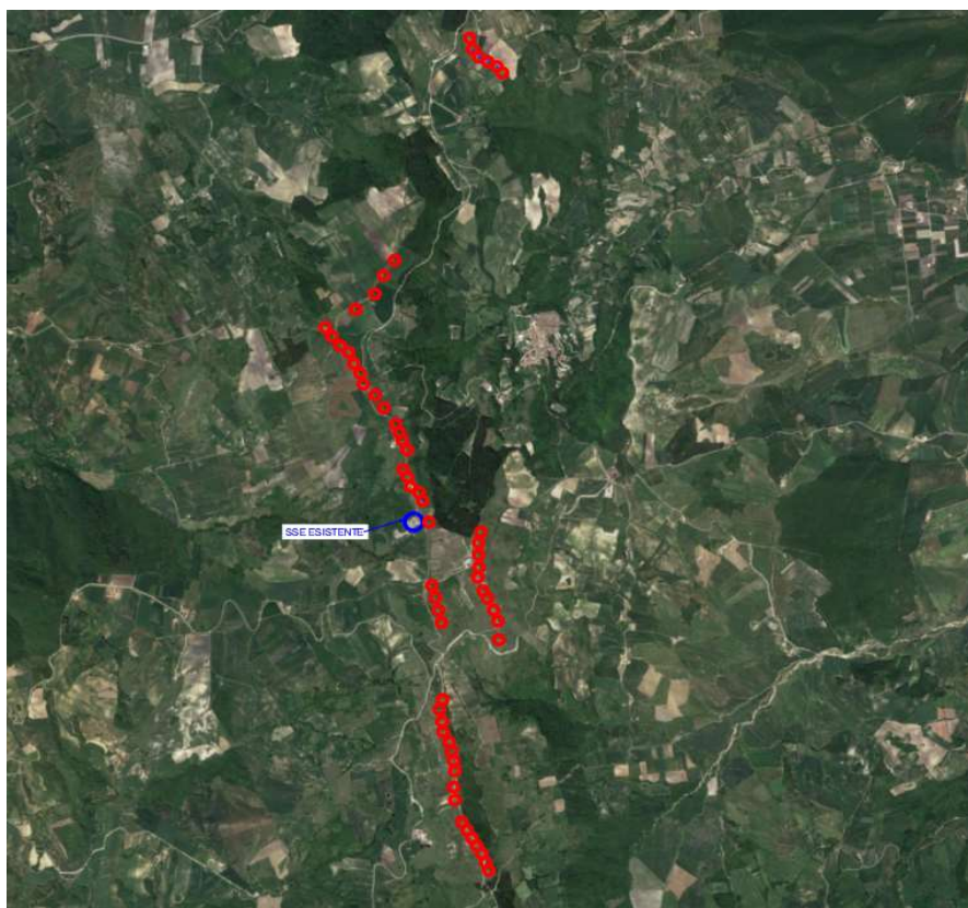
Fig. 2. Layout dell'impianto esistente da dismettere (in rosso i 60 aerogeneratori).
