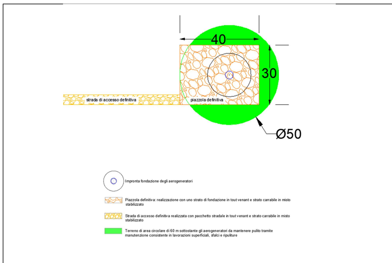
Fig. 16a Schema della piazzola definitiva ai fini della mitigazione del rischio incendio.
