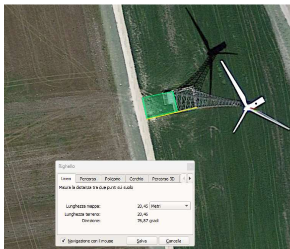
Fig. 3 Esempio di piazzola di aerogeneratore esistente. L'area tra la strada e la cabina (area verde) è la piazzola libera di manovra e sosta per le attività di controllo e manutenzione
