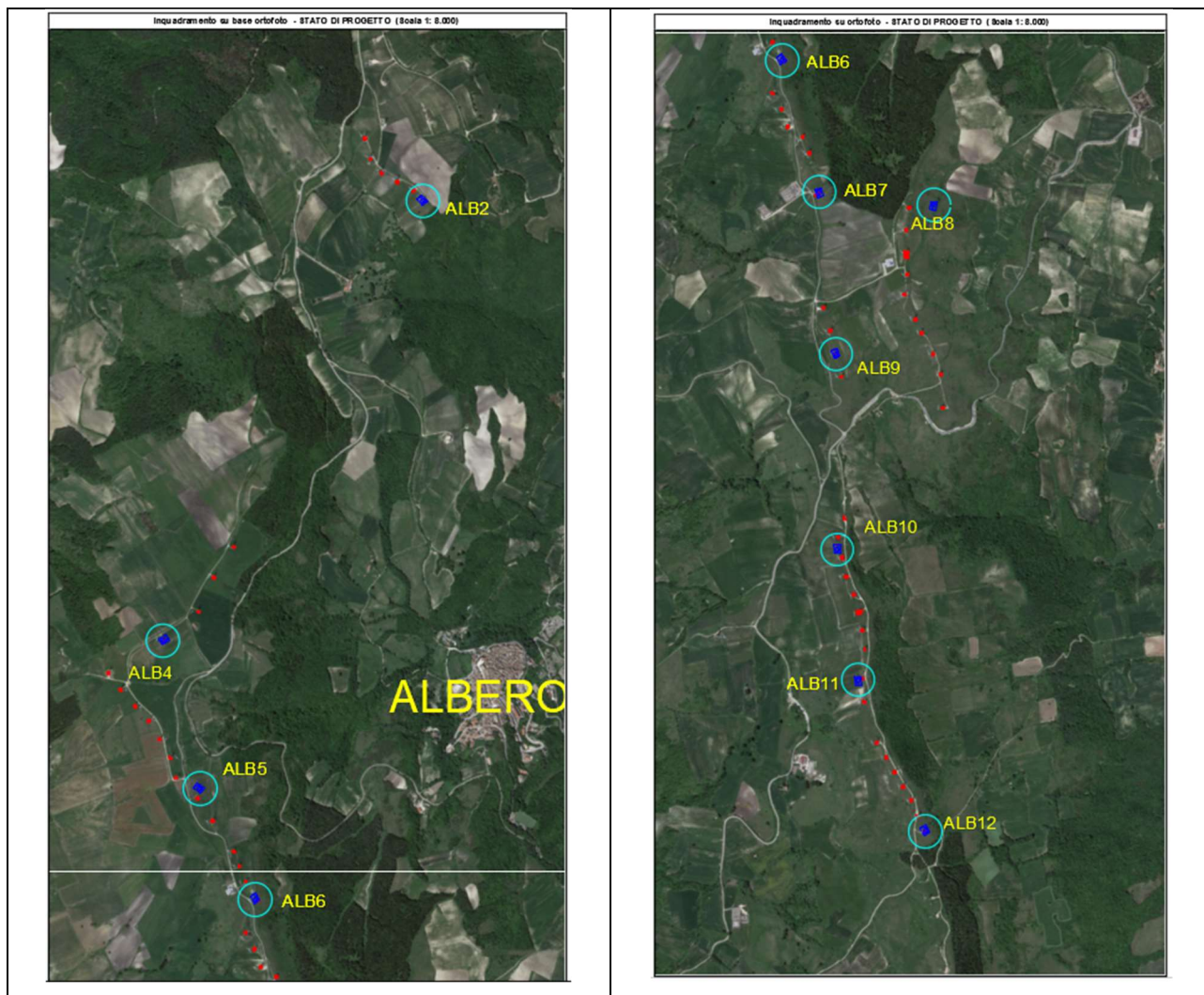
Fig. 7. Sovrapposizione del layout impianto esistente e di quello nuovo (punti in rosso: impianto esistente. Punti in blu e cerchi ciano: impianto nuovo)
