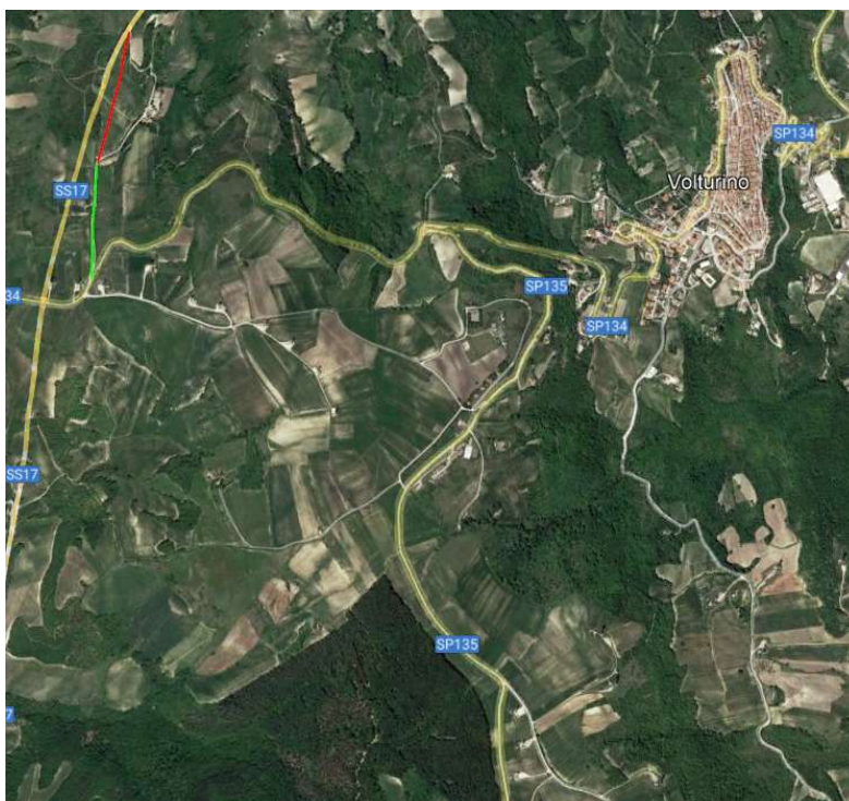
Fig. 18 Viabilità di accesso al parco eolico. In alto a sinistra tratto in rosso corrispondente alla bretella temporanea di collegamento della SS17var alla strada comunale. Tratto in verde strada comunale di collegamento tra la bretella temporanea e la SP135.
