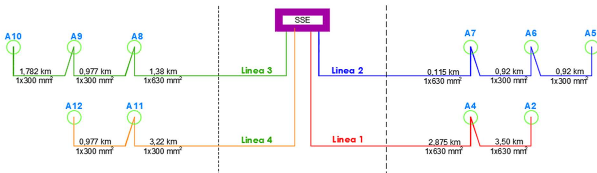
Fig. 15 Schema elettrico a deformata di collegamento degli aerogeneratori alla sottostazione
