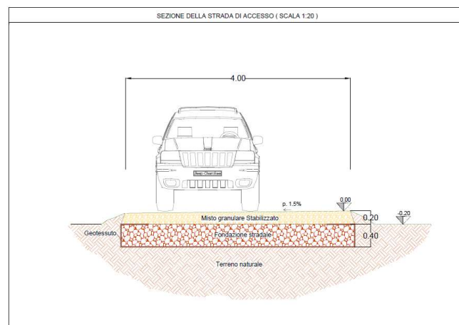
Fig. 17 Schema della sezione stradale per nuova viabilità.
