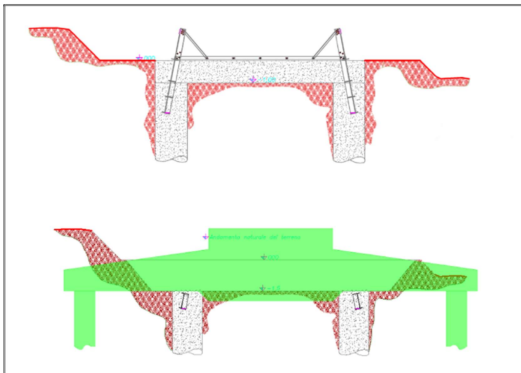
Fig. 21 Schema tipico di alloggiamento della nuova fondazione (colore verde) su fondazione esistente e parzialmente demolita (colore grigio).
