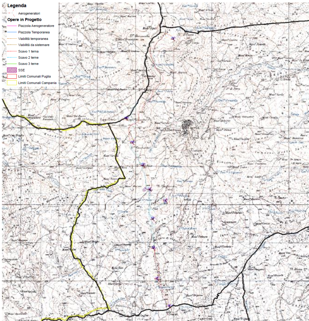
Figura 2.7. – Stralcio Inquadramento Impianto su I.G.M.
