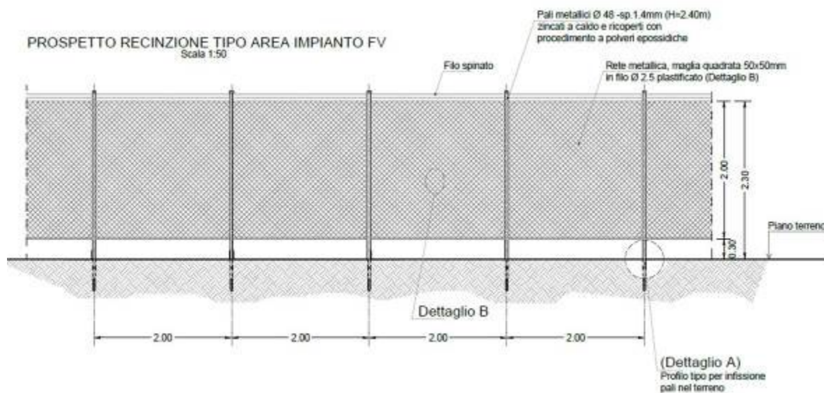
Figura 8 – Prospetto recinzione impianto agrivoltaico
