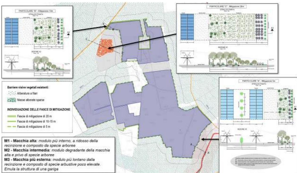
Figura 7 – Fasce di mitigazione campo agrovoltaiico: larghezza 5 m (Particolare “A”), larghezza 10 m (Particolare “B”) e larghezza 20 m (Particolare “C”)
