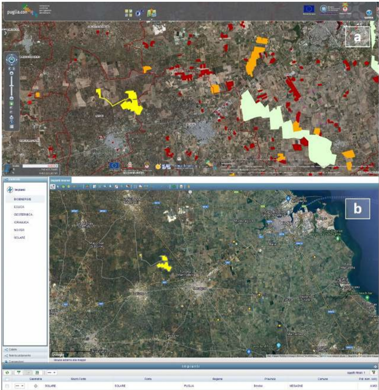
Figura 5 – Stato dei luoghi rispetto all’area di progetto (in giallo) alla presenza di FER: a) presenza di impianti fotovoltaici (Fonte: portale pubblico GSE); b) presenza impianti fotovoltaici (Fonte: portale puglia.con)
