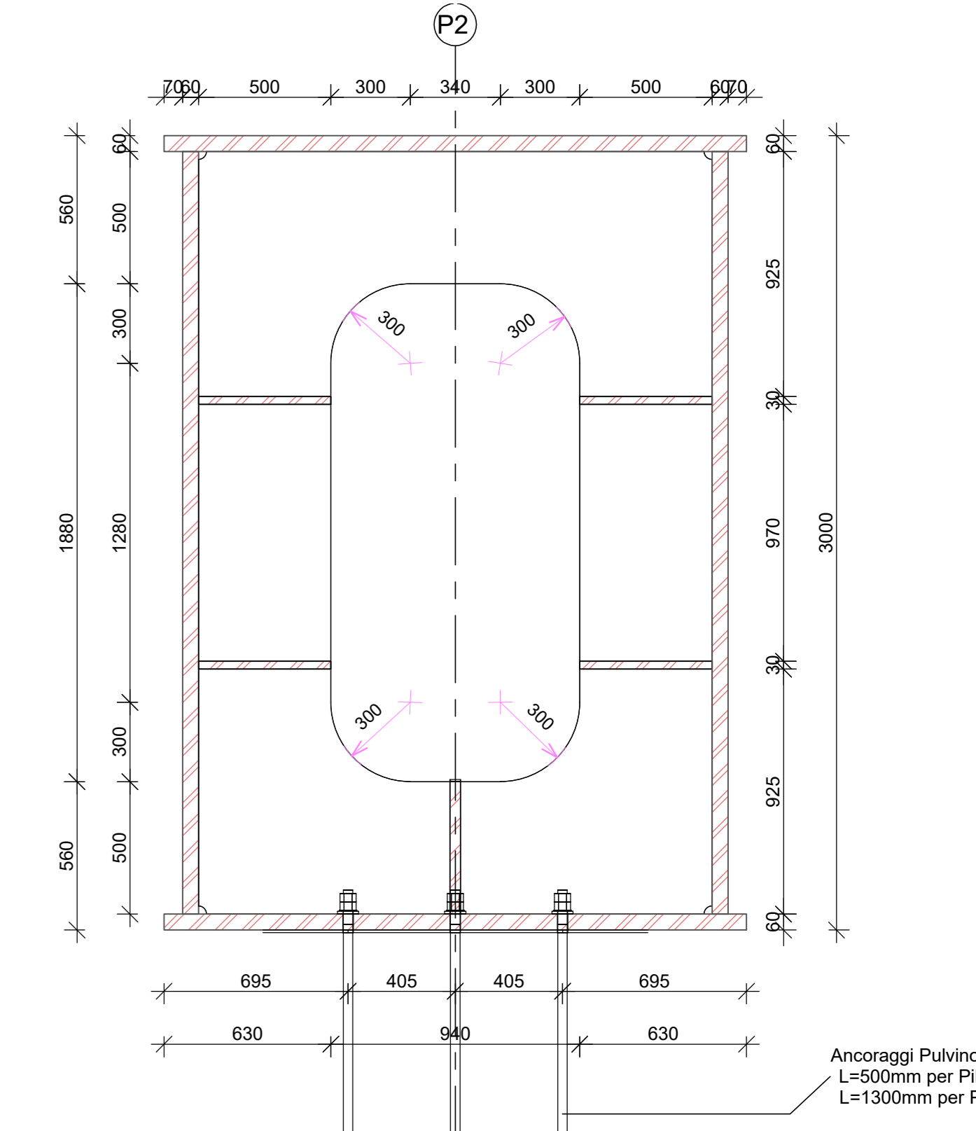
Pulvino - Sezione Longitudinale 2 1 : 20
