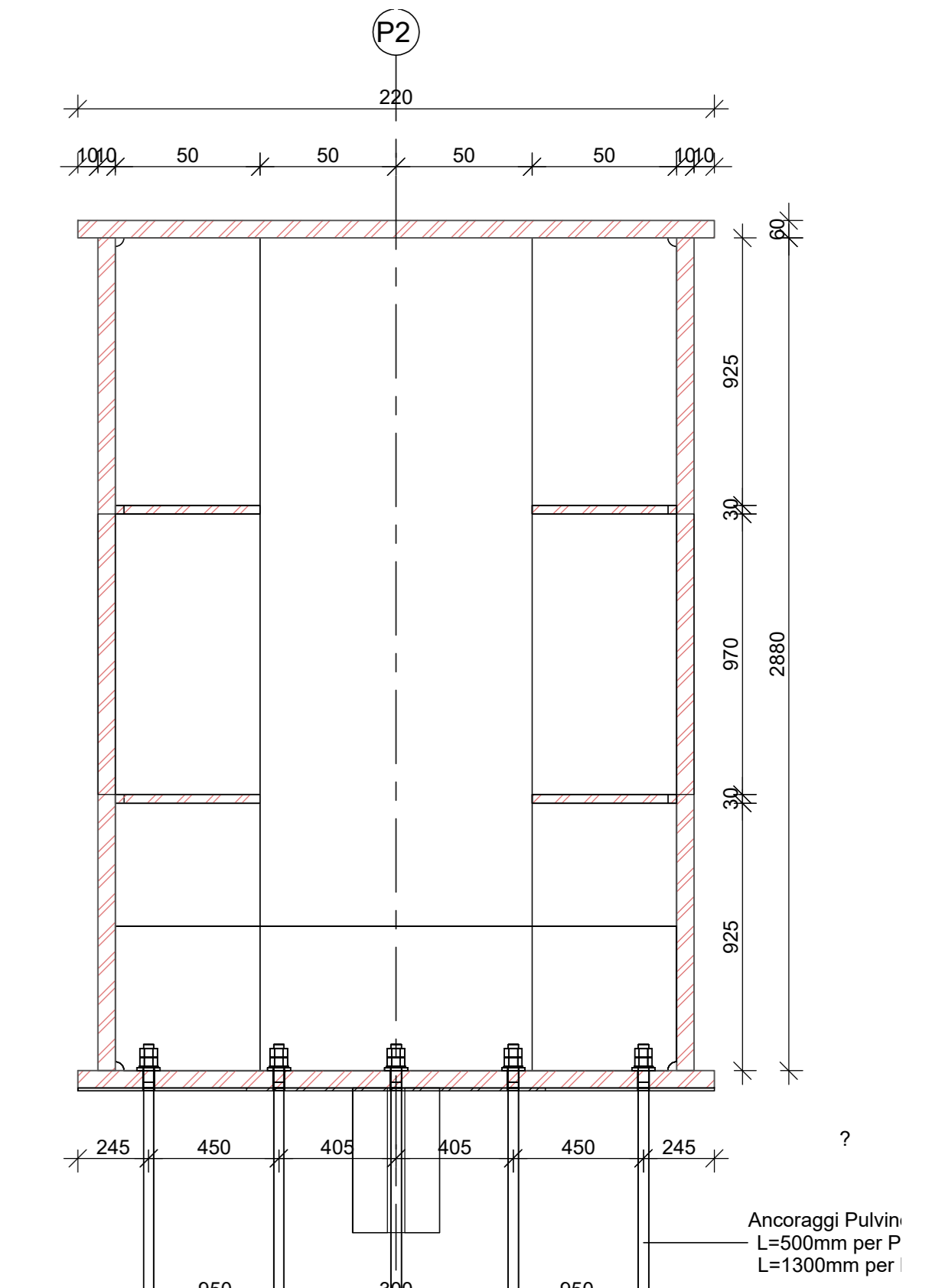
Pulvino - Sezione Longitudinale 2 1 : 20
