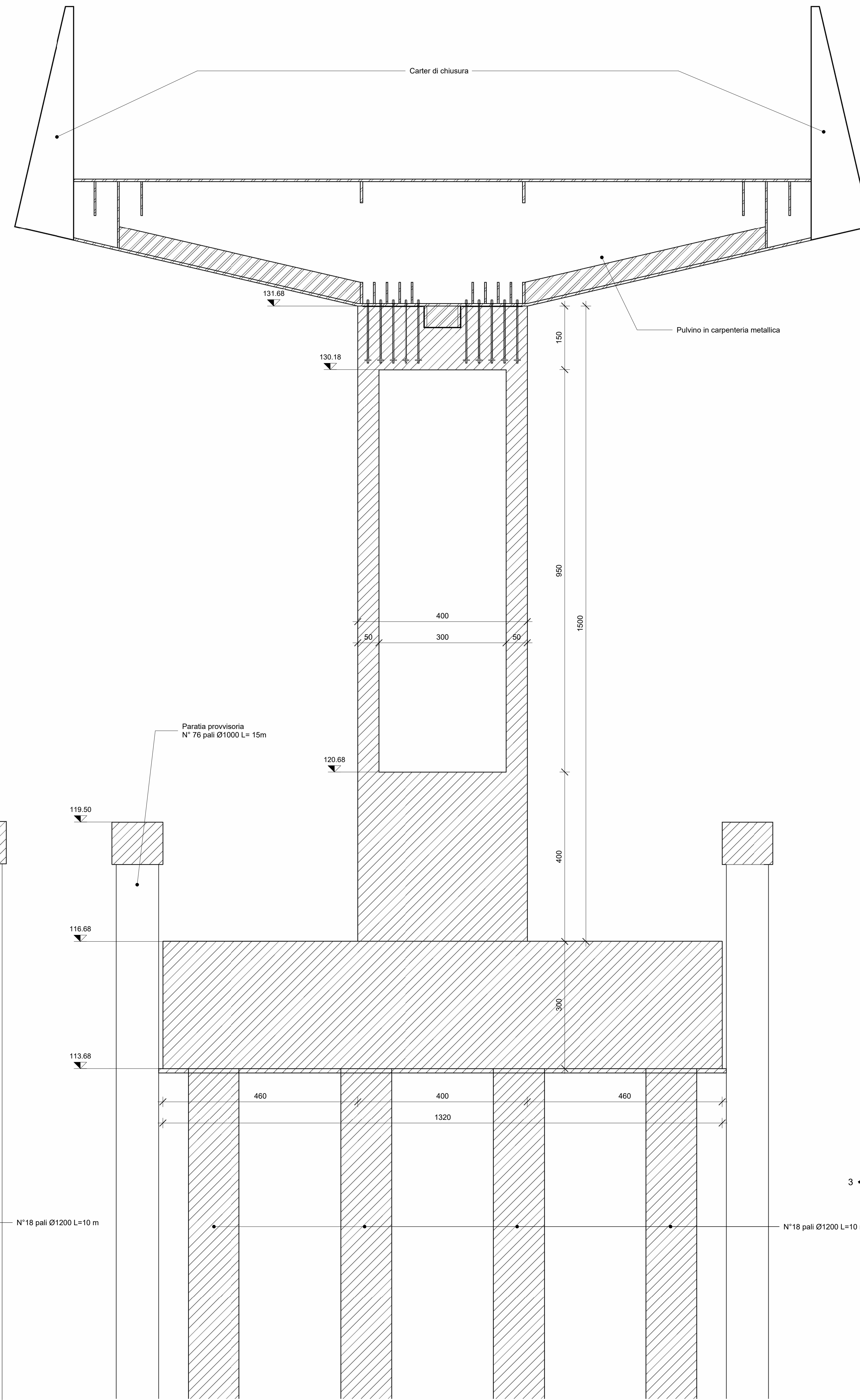
P4 - Sezione Trasversale 1 : 50
