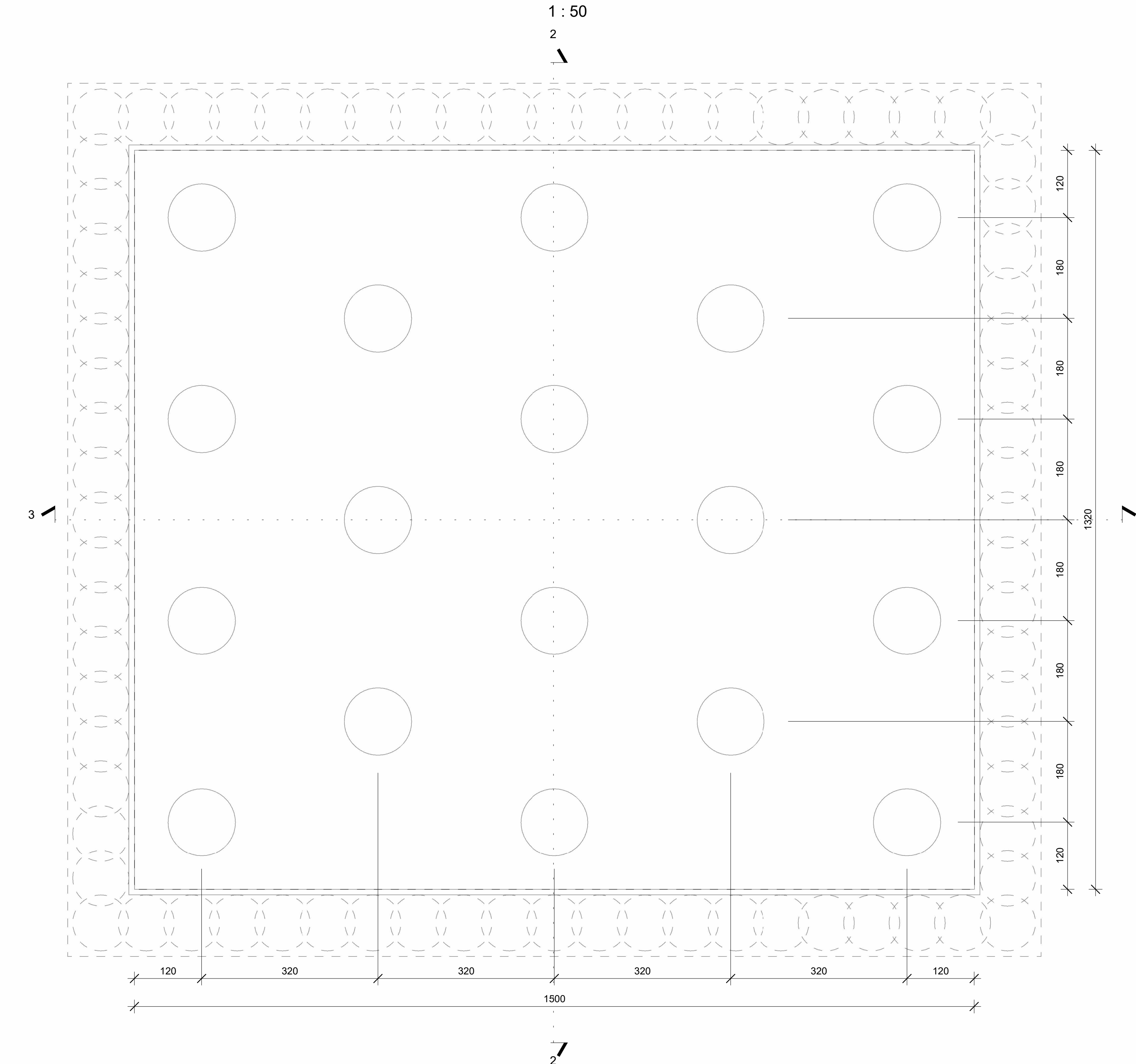
P4 - Sezione Orizzontale Pila 1 : 50
