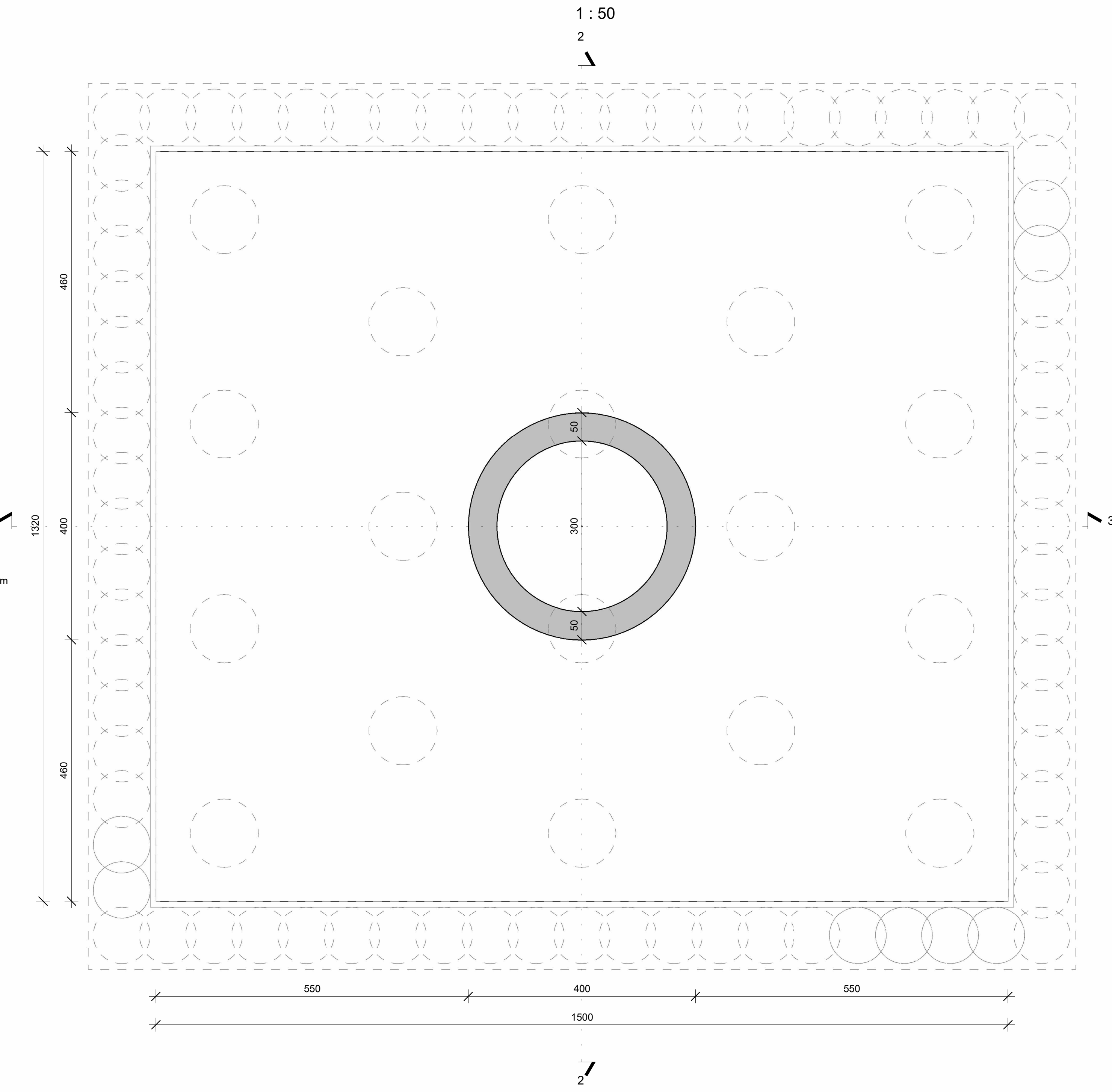
P4 - Sezione Orizzontale Pila 1 : 50
