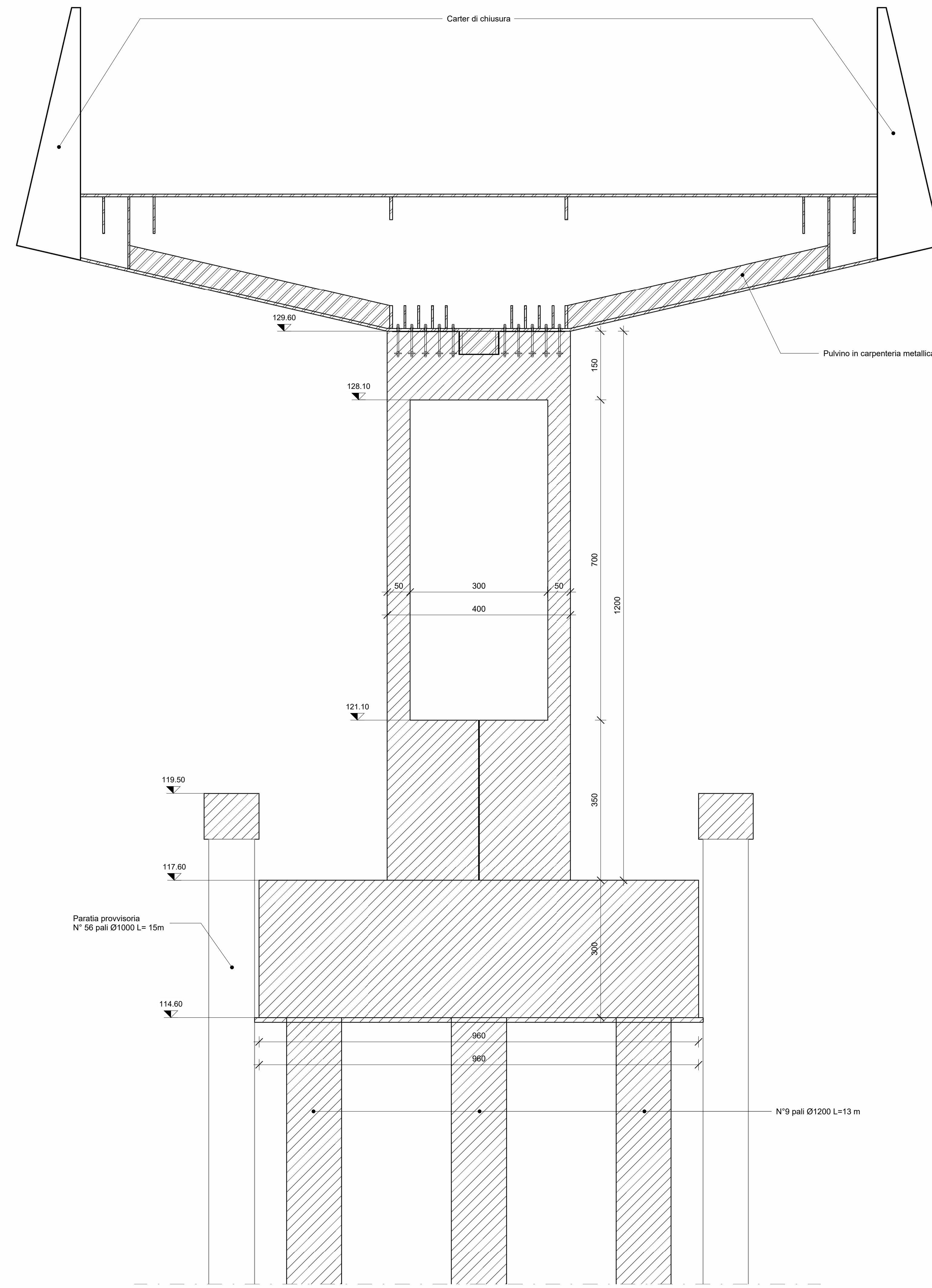
P5 - Sezione Trasversale 1 : 50
