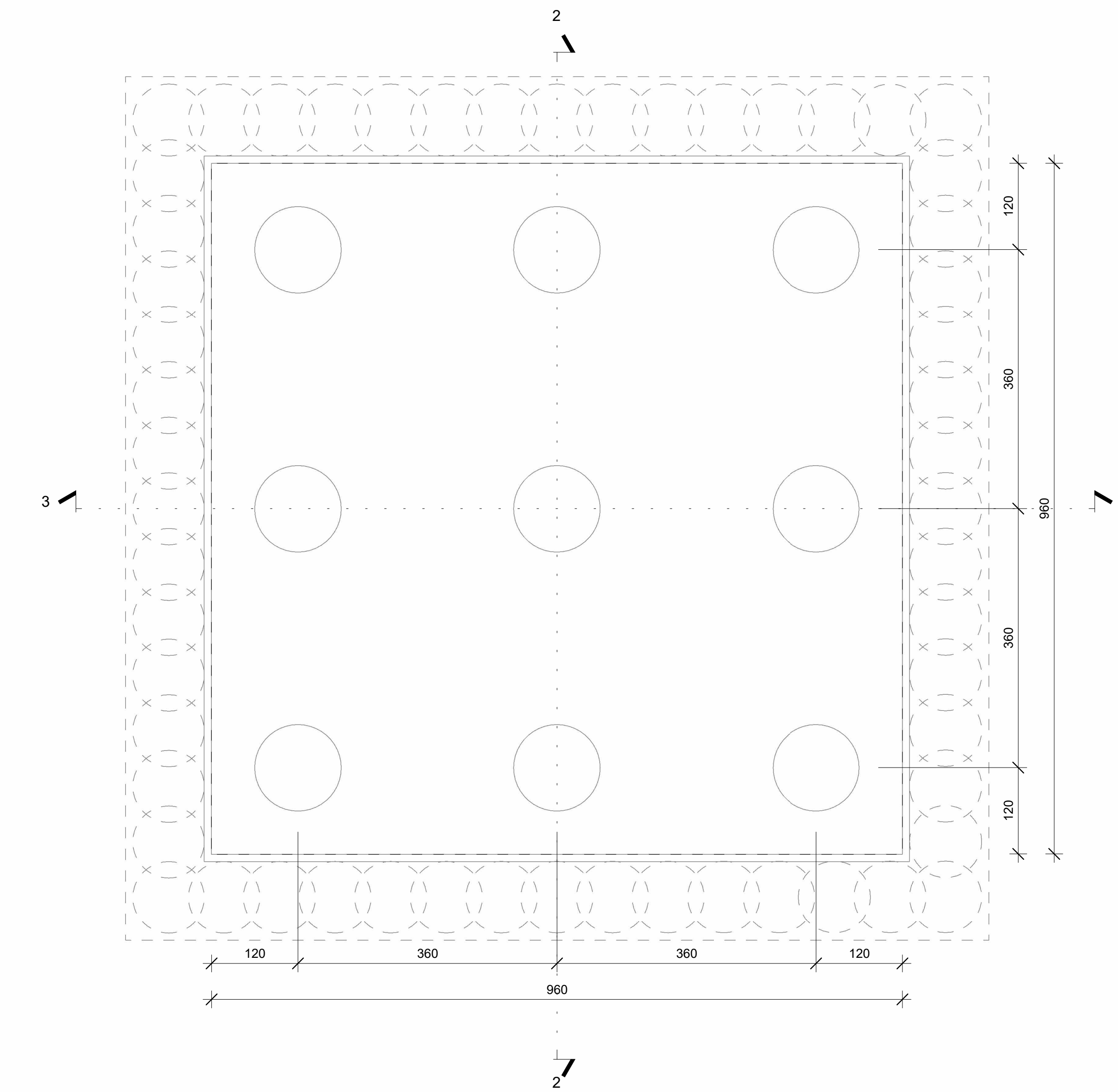
P5 - Pianta Fondazione 1 : 50
