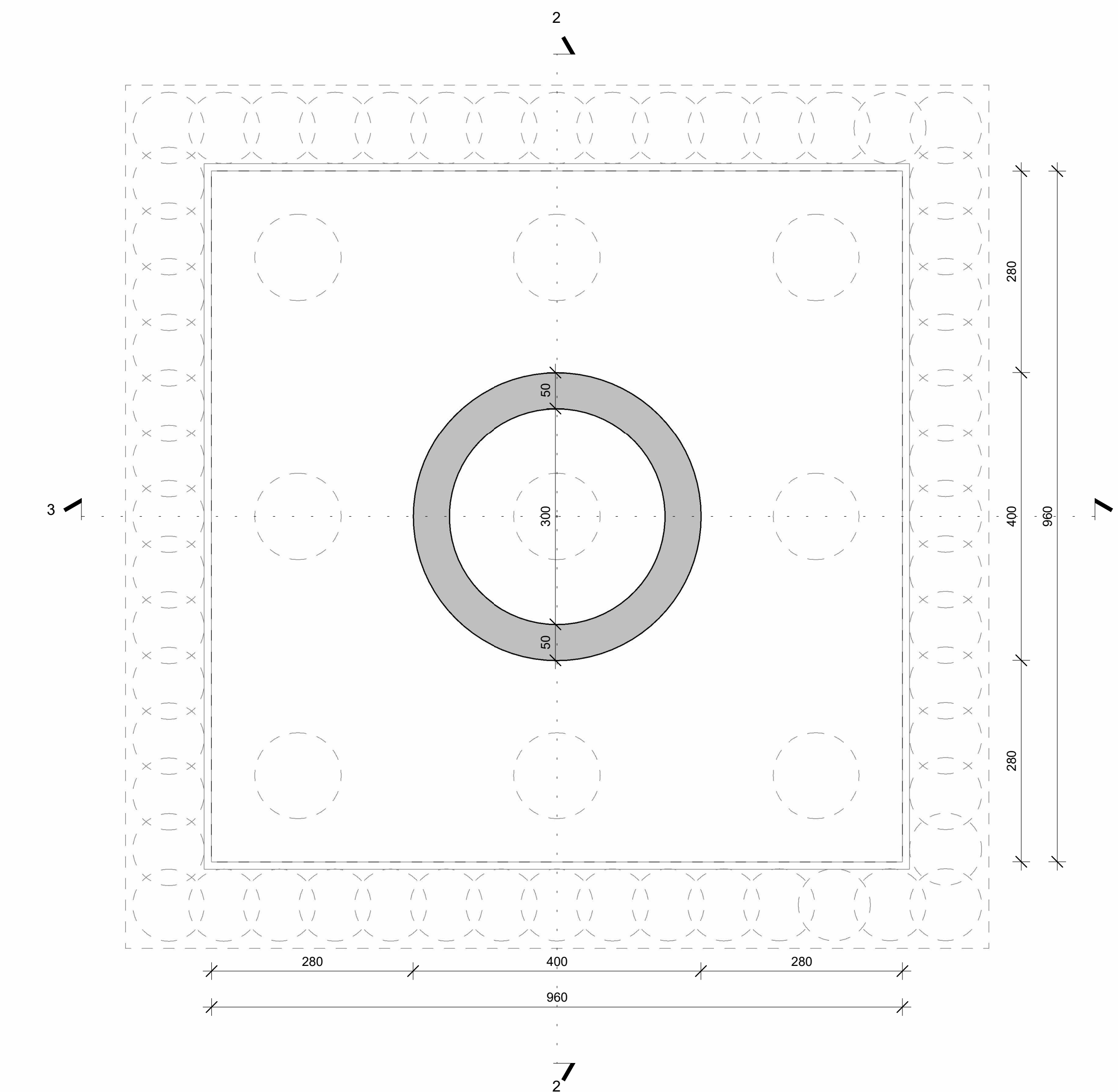
P5 - Sezione Orizzontale Pila 1 : 50
