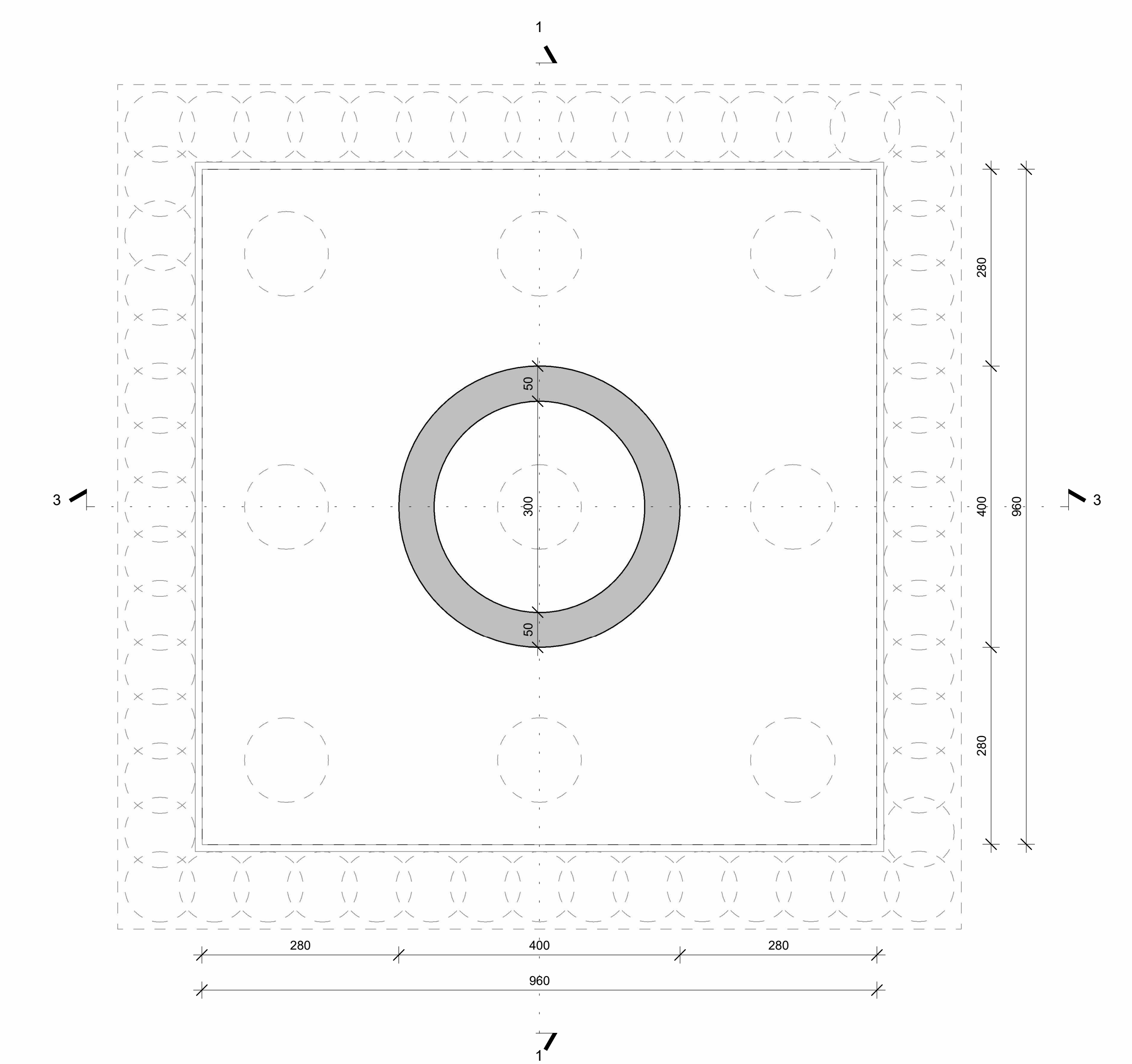
P6 - Sezione Orizzontale Pila 1 : 50
