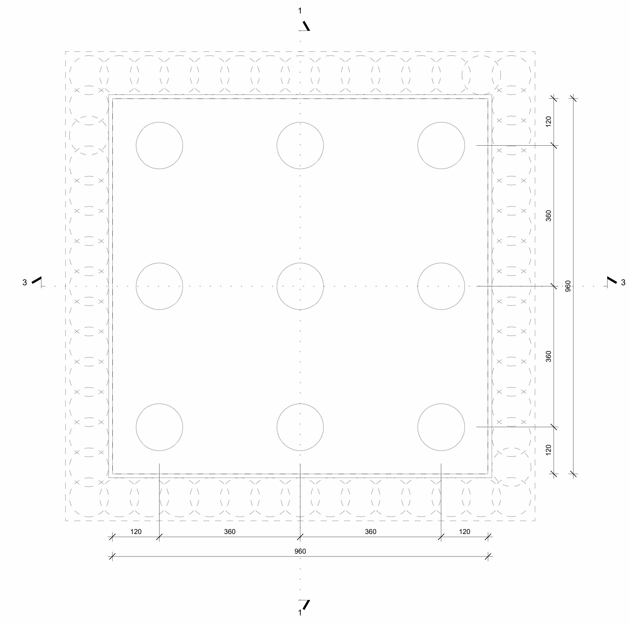
P6 - Sezione Orizzontale Pila 1 : 50
