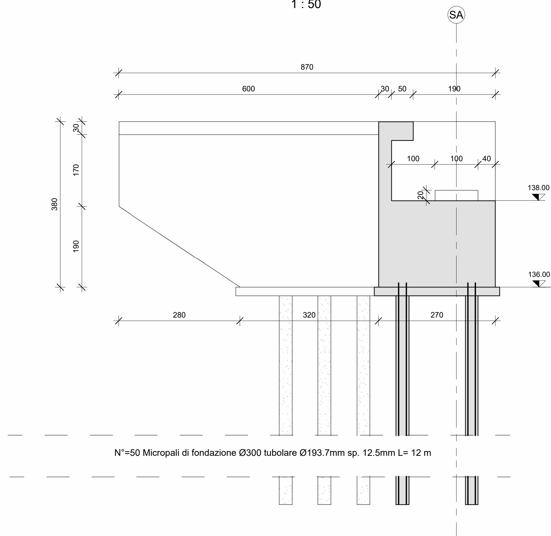
Sezione B - B 1 : 50
