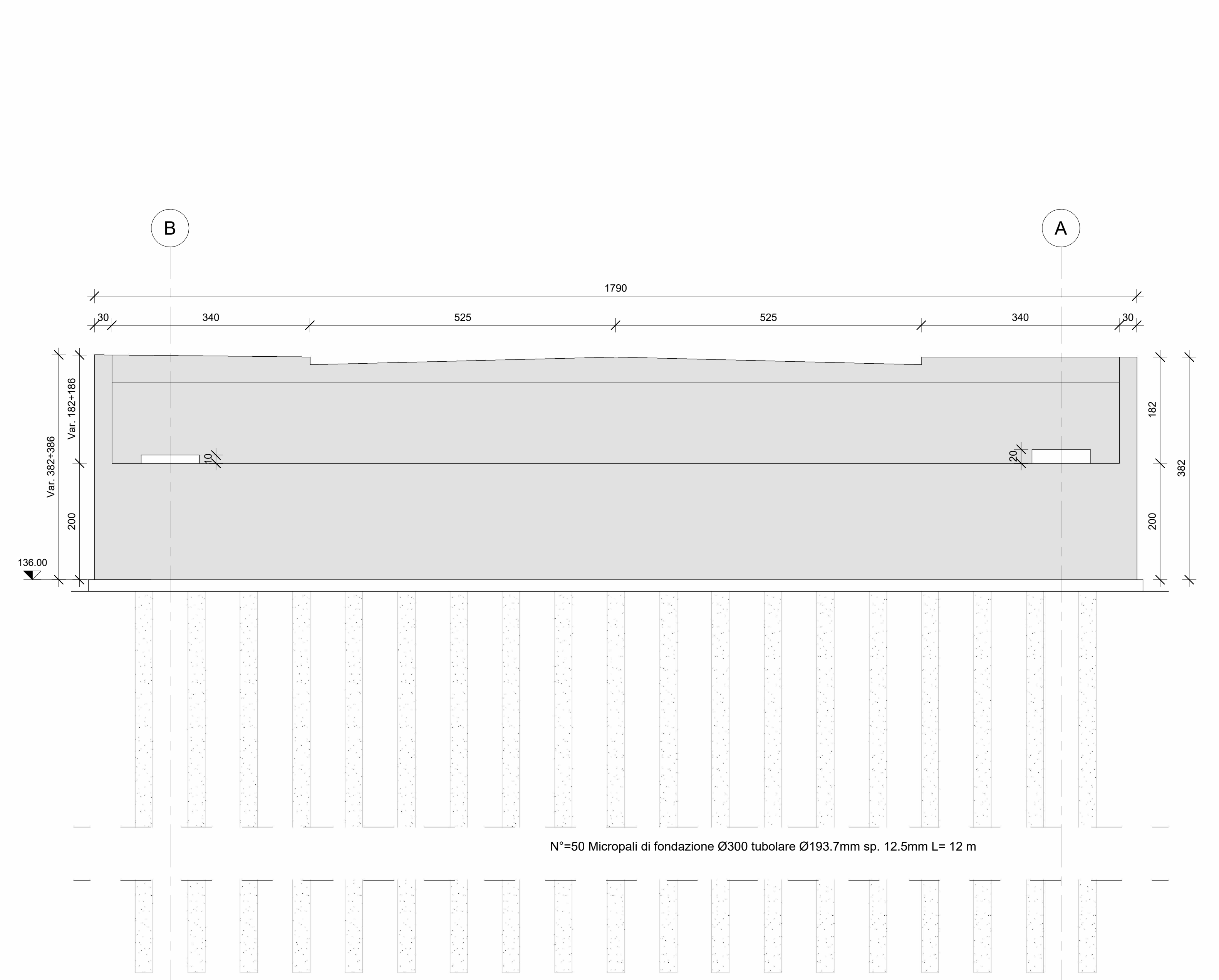
Sezione A - A 1 : 50
