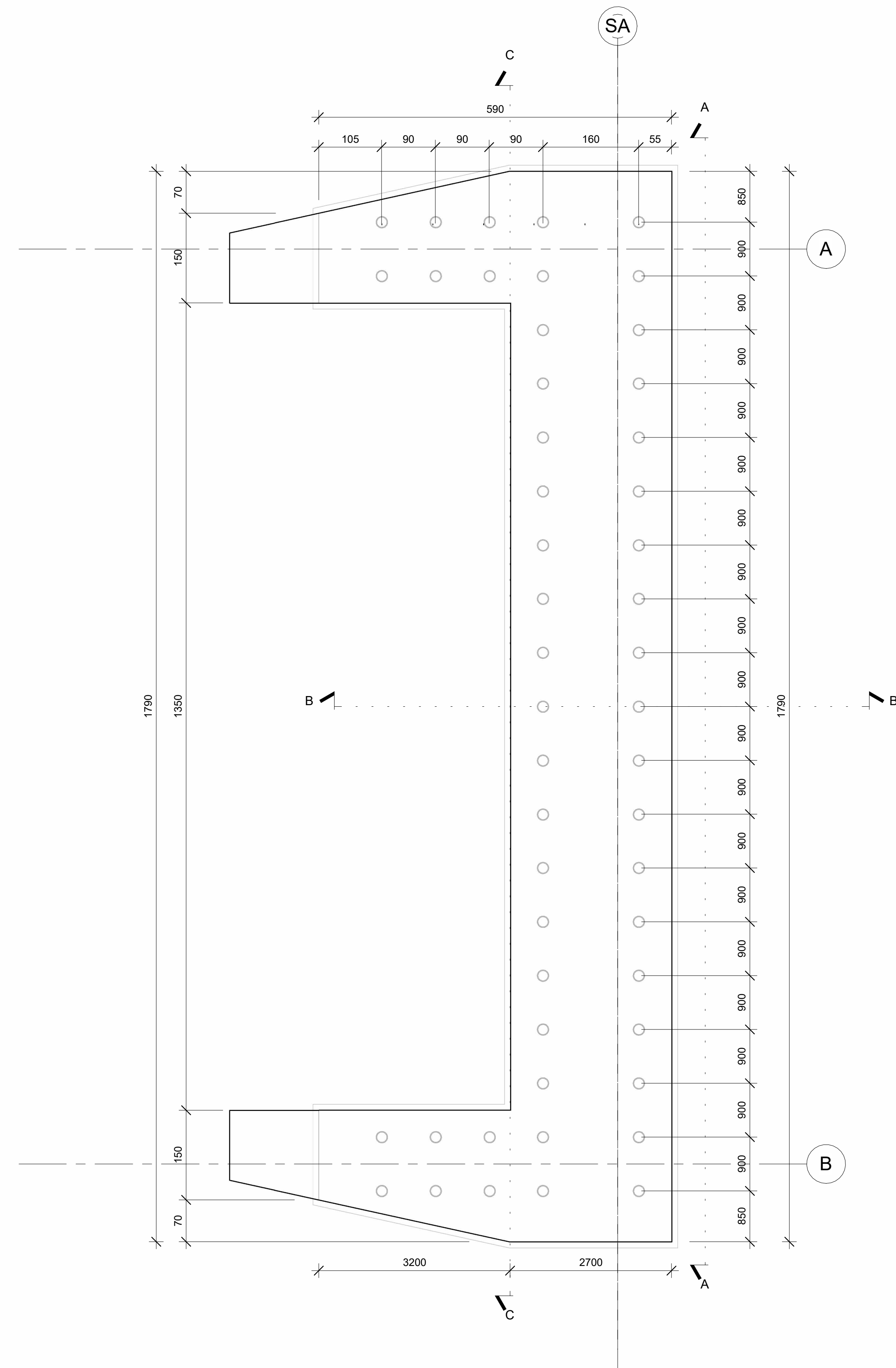
Pianta della Fondazione 1 : 50
