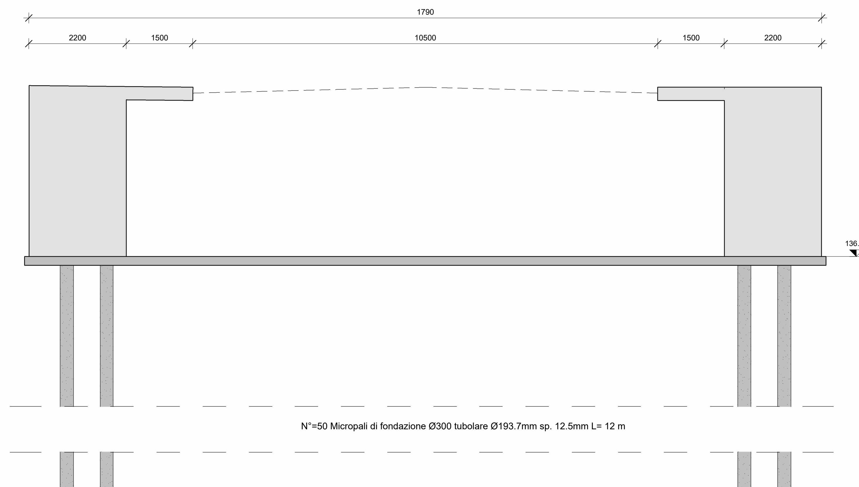
Sezione C - C 1 : 50
