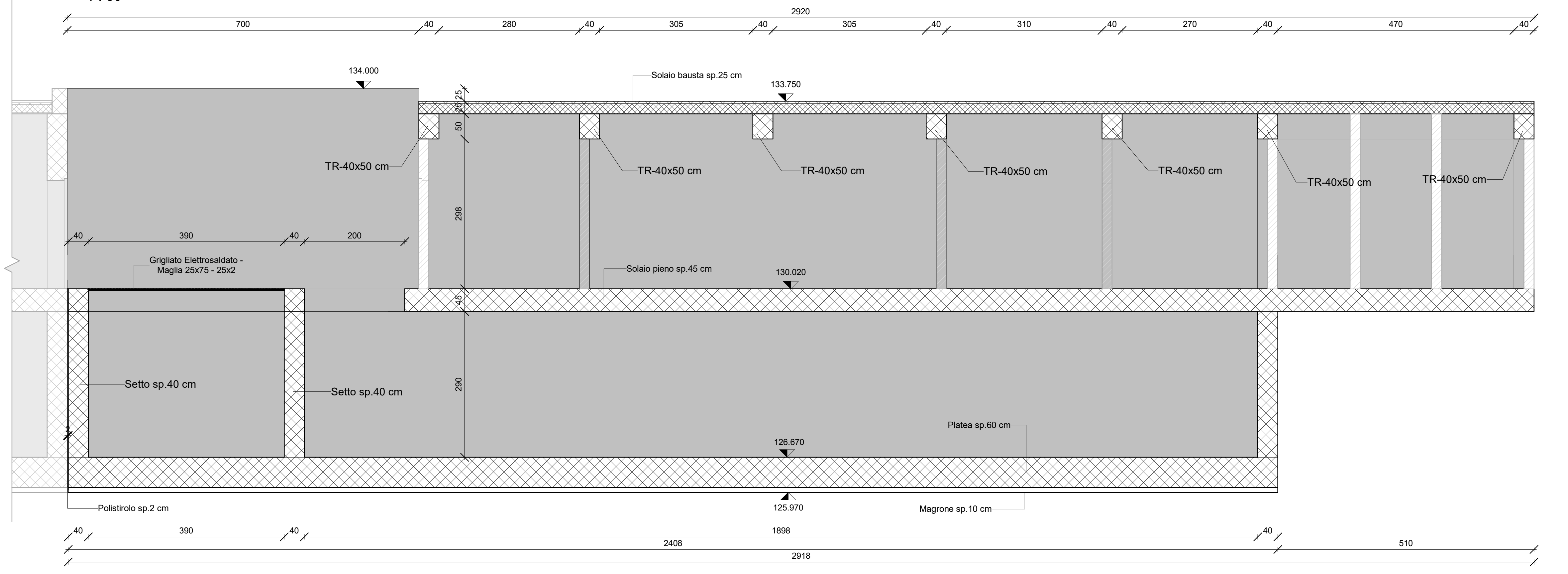
Sezione B-B 1 : 50
