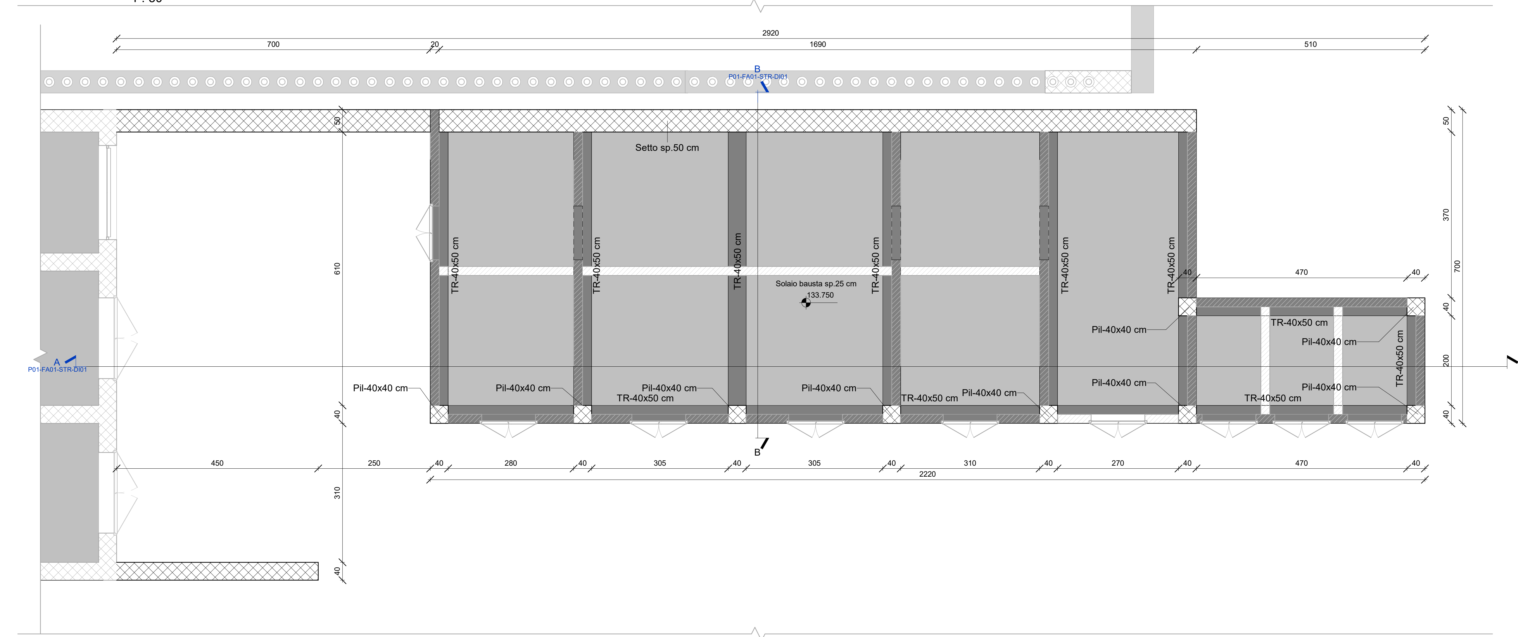
Carpenteria solaio Q.133.77 m 1 : 50
