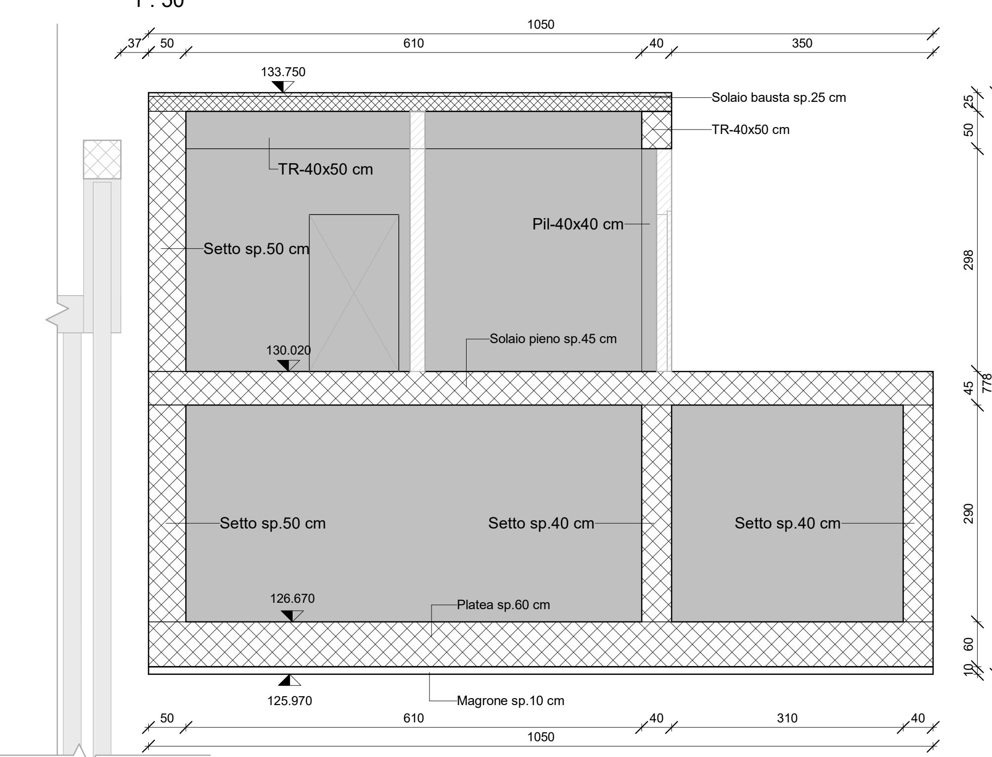
Sezione B-B 1 : 50
