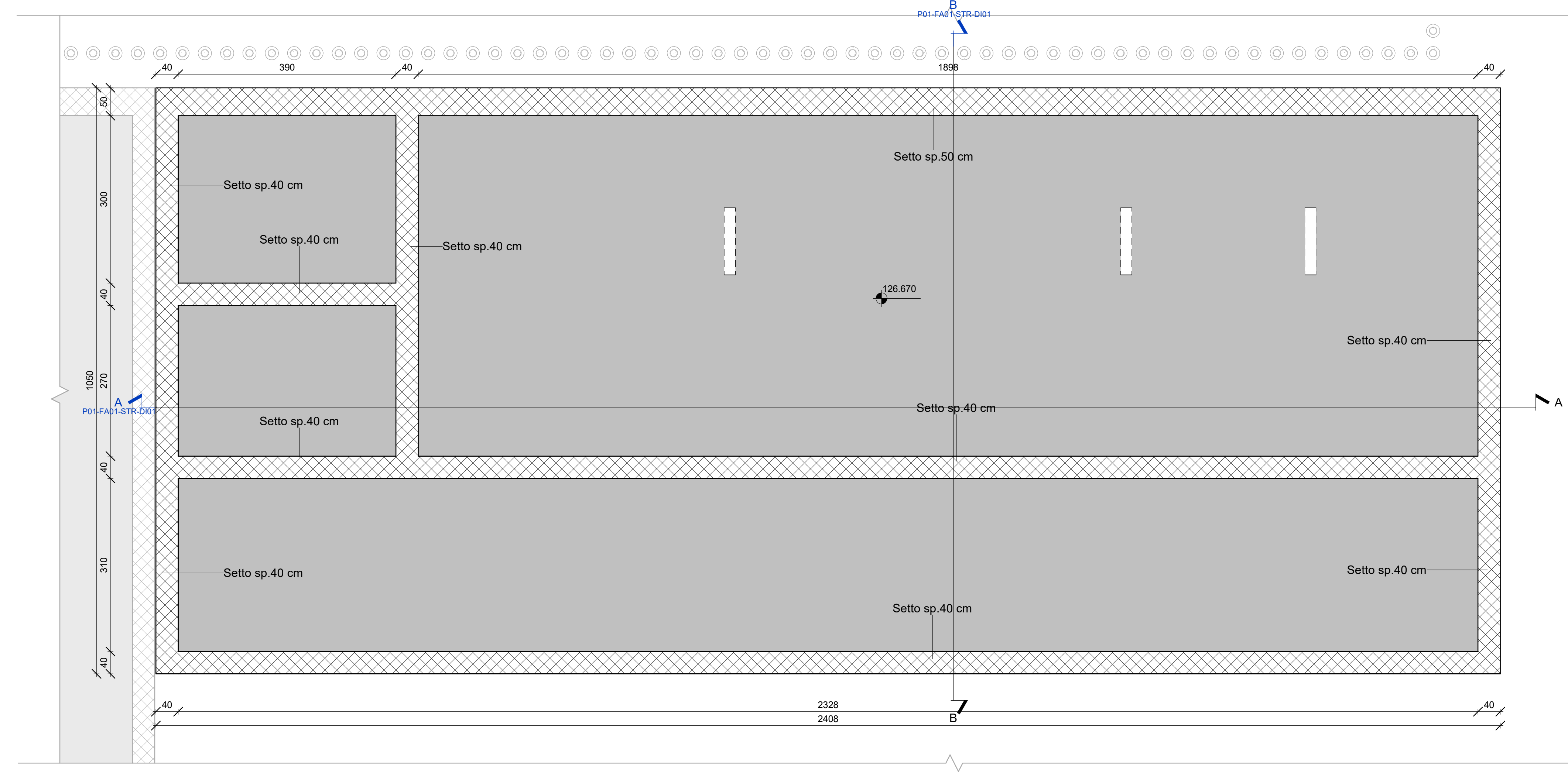
Pianta fondazione 1 : 50
