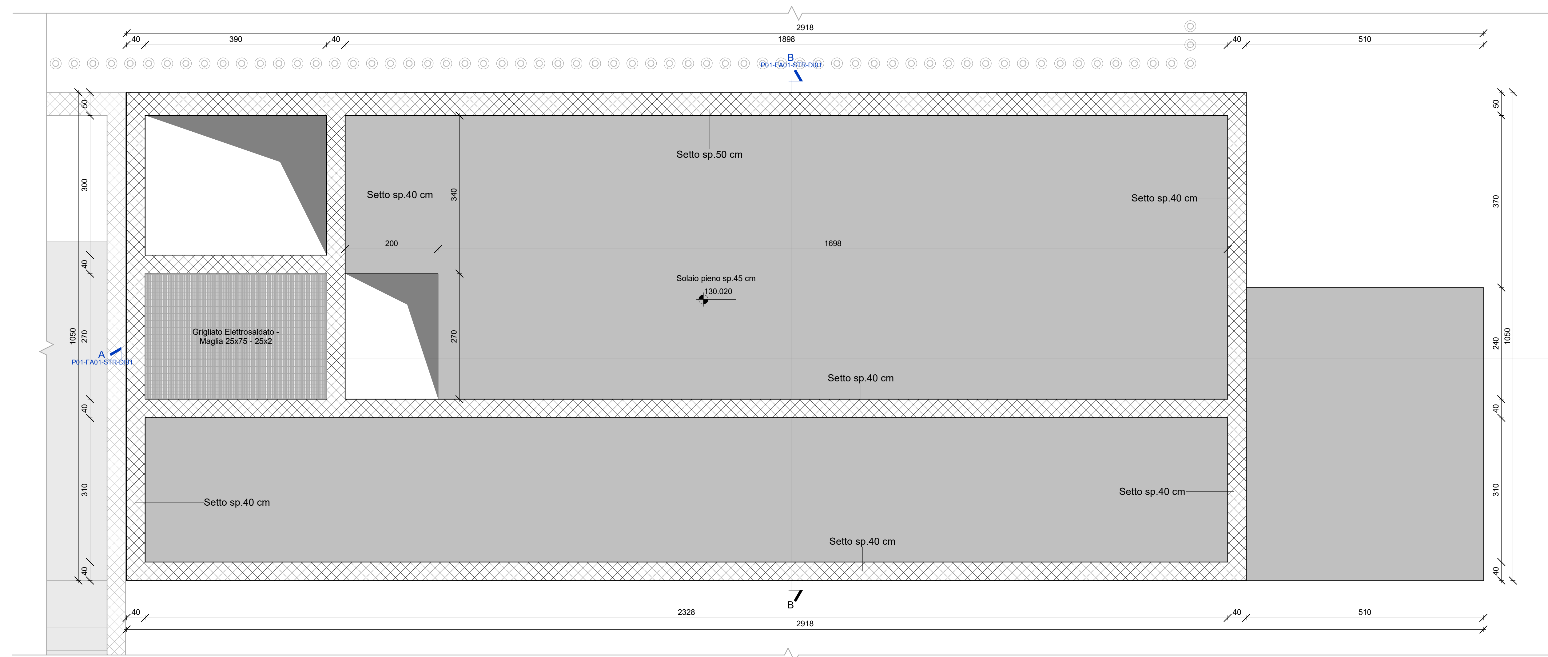
Carpenteria solaio Q.130.02 m 1 : 50
