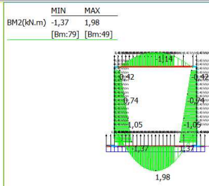
20: SISMICA PSEUDOST.: PP Soletta + piedritti verticale (-1,0,0)
