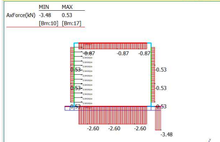
28: SPINTA SISMICA PIEDRITTI: PAVIMENTAZIONE (G2) (0,0,0)
