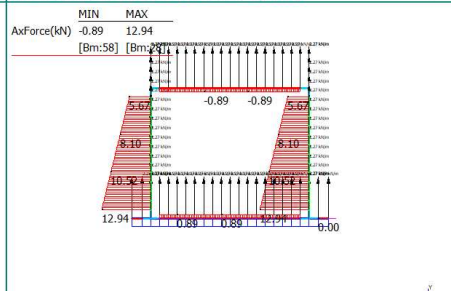
24: SISMICA PSEUDOST.: TANDEM VERTICALE (0,0,0)
