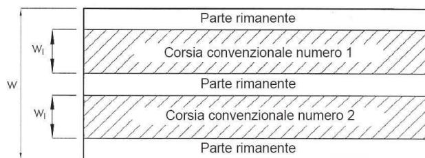
ESEMPIO DI NUMERAZIONE DELLE CORSIE
