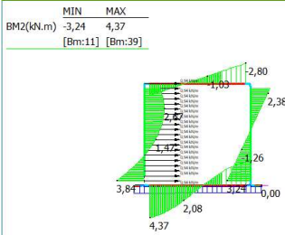
25: SISMICA PSEUDOST.: TRAFFICO DISTRIBUITO ORIZZONTALE (-1,0,0)
