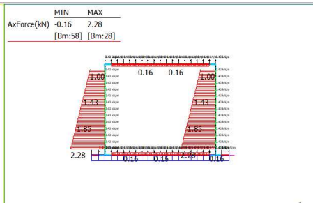
20: SISMICA PSEUDOST.: PP Soletta + piedritti verticale (0,0,0)
