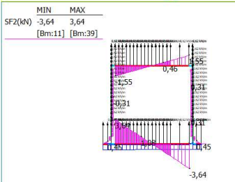
19: SISMICA PSEUDOST.: PP soletta + piedritti orizzontale (-1,0,0)
