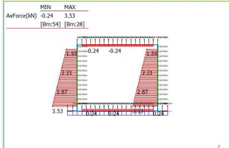
22: SISMICA PSEUDOST.: G2 verticale (0,0,0)
