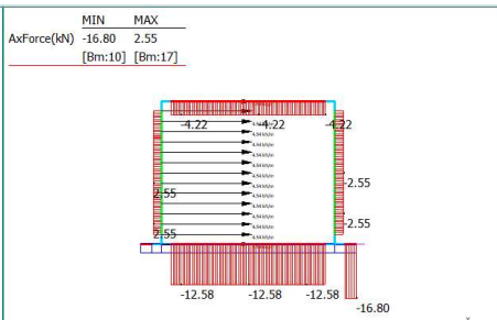
27: SPINTA SISMICA PIEDRITTI: RILEVATO (G2) (0,0,0)
