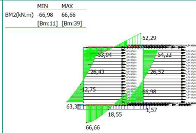
20: SISMICA PSEUDOST.: PP Soletta + piedritti verticale (-1,0,0)
