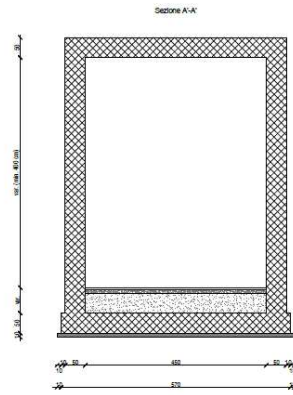
SEZIONE TRASVERSALE A'-A' SOTTOPASSO ST.02 - Scala 1:50
