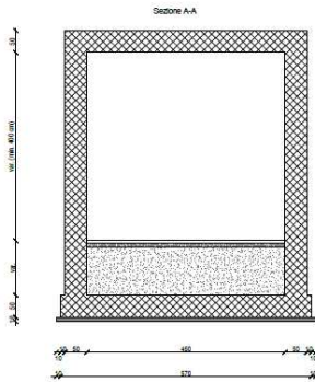
SEZIONE TRASVERSALE A-A SOTTOPASSO ST.02 - Scala 1:50
