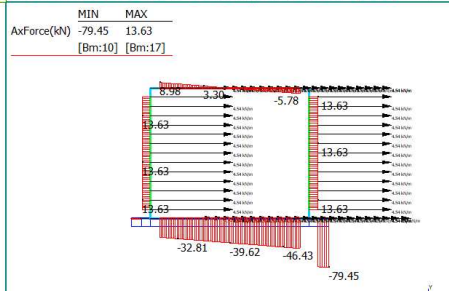
23: SISMICA PSEUDOST.: TANDEM ORIZZONTALE (0,0,0)
