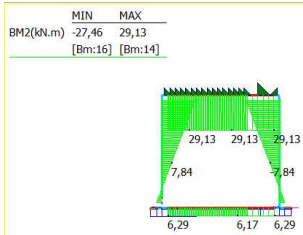
10: temperatura uniforme e3 (contrazione) (-1,0,0)
