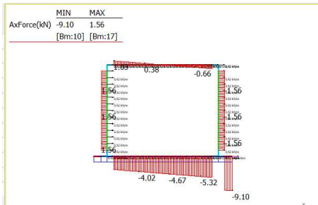
25: SISMICA PSEUDOST.: TRAFFICO DISTRIBUITO ORIZZONTALE (0,0,0)
