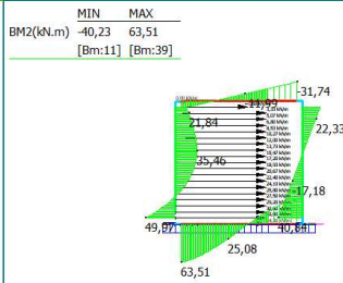
26: SISMICA PSEUDOST.: TRAFFICO DISTRIBUITO VERTICALE (-1,0,0)
