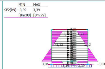
15: Spinta statica: pavimentazione (-1,0,0)
