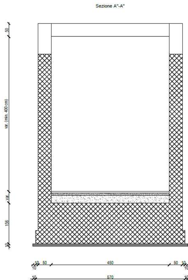
FIGURA 2: CARPENTERIE ELEMENTI DI SBocco/IMBOCCO
