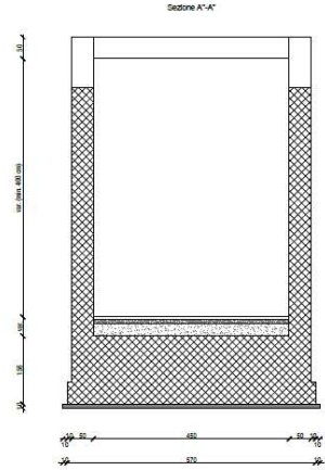
SEZIONE TRASVERSALE A''-A'' SOTTOPASSO ST.02 - Scala 1:50
