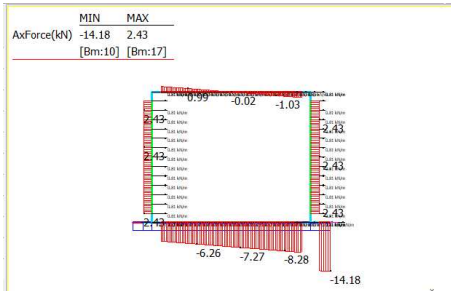
19: SISMICA PSEUDOST.: PP soletta + piedritti orizzontale (0,0,0)
