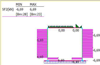
13: gradiente temperatura e3 (intradosso caldo) (-1,0,0)
