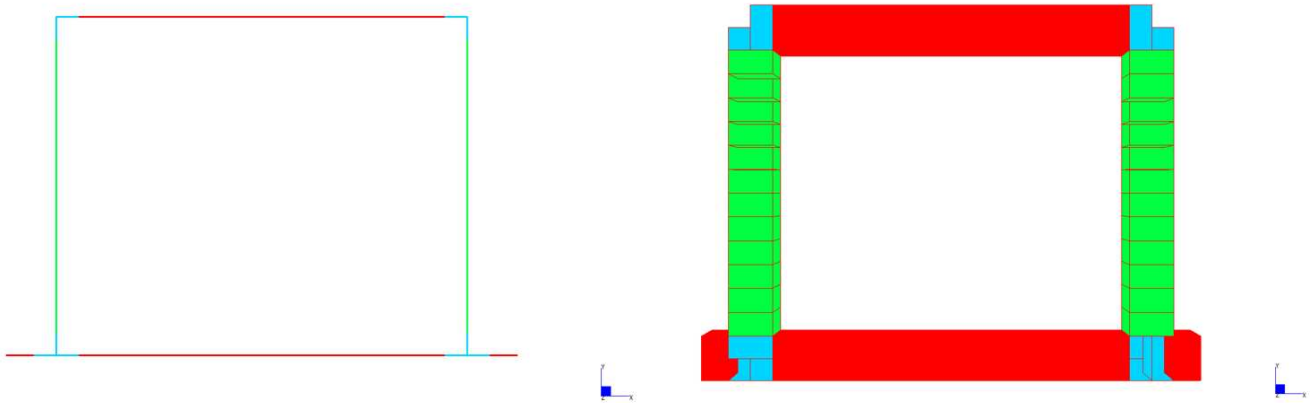
MODELLO DI CALCOLO: VISTA SOLIDA E FILIFORME
