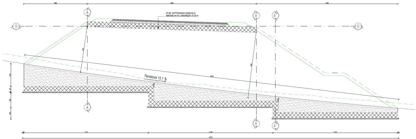
SEZIONE LONGITUDINALE ASSE SOTTOPASSO AGRICOLO ST.02 - Scala 1:50
