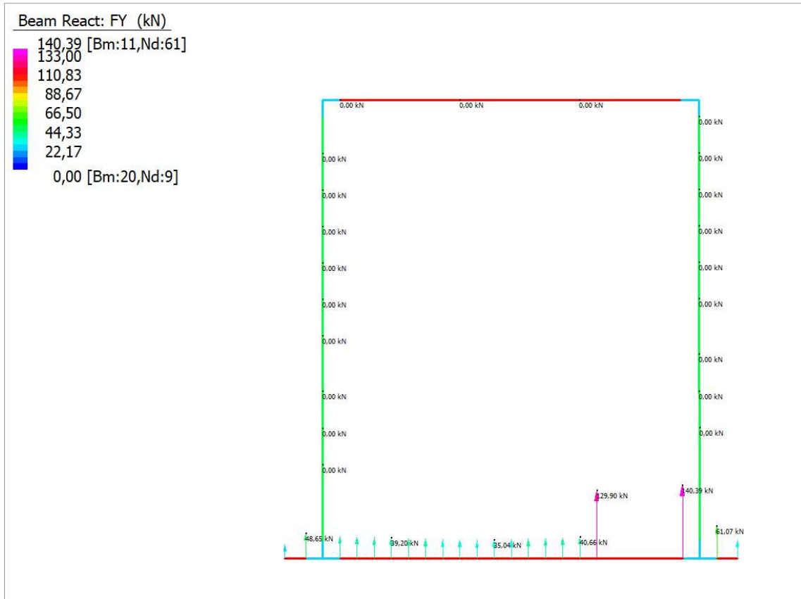
FIGURA 1: REAZIONI VINCOLARI NODALI
