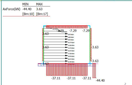
29: SPINTA SISMICA PIEDRITTI; TERRENO (0,0,0)
