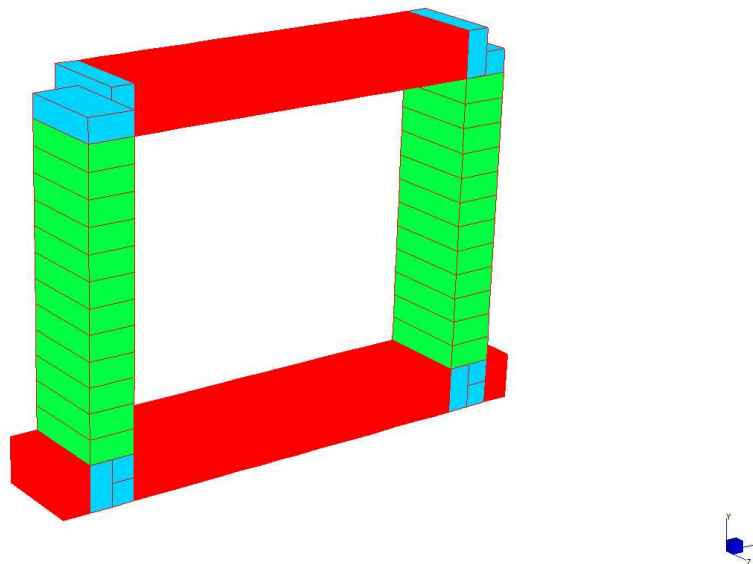
MODELLO DI CALCOLO
