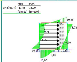
14: Spinta statica: Terreno di riporto (-1,0,0)
