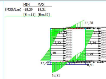
21: SISMICA PSEUDOST.: G2 orizzontale (-1,0,0)
