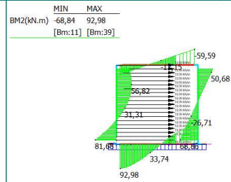
27: SPINTA SISMICA PIEDRITTI: RILEVATO (G2) (-1,0,0)
