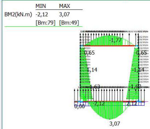
19: SISMICA PSEUDOST.: PP soletta + piedritti orizzontale (-1,0,0)
