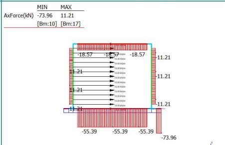
30: SPINTA SISMICA PIEDRITTI: TANDEM (0,0,0)
