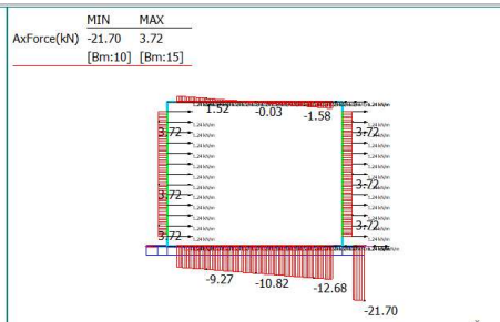
21: SISMICA PSEUDOST.: G2 orizzontale (0,0,0)
