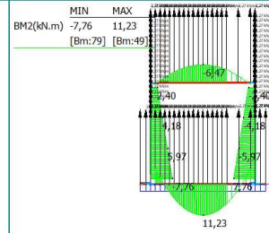
21: SISMICA PSEUDOST.: G2 orizzontale (-1,0,0)
