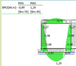
26: SISMICA PSEUDOST.: TRAFFICO DISTRIBUITO VERTICALE (-1,0,0)
