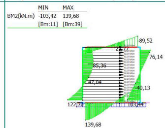
15: Spinta statica: pavimentazione (-1,0,0)
