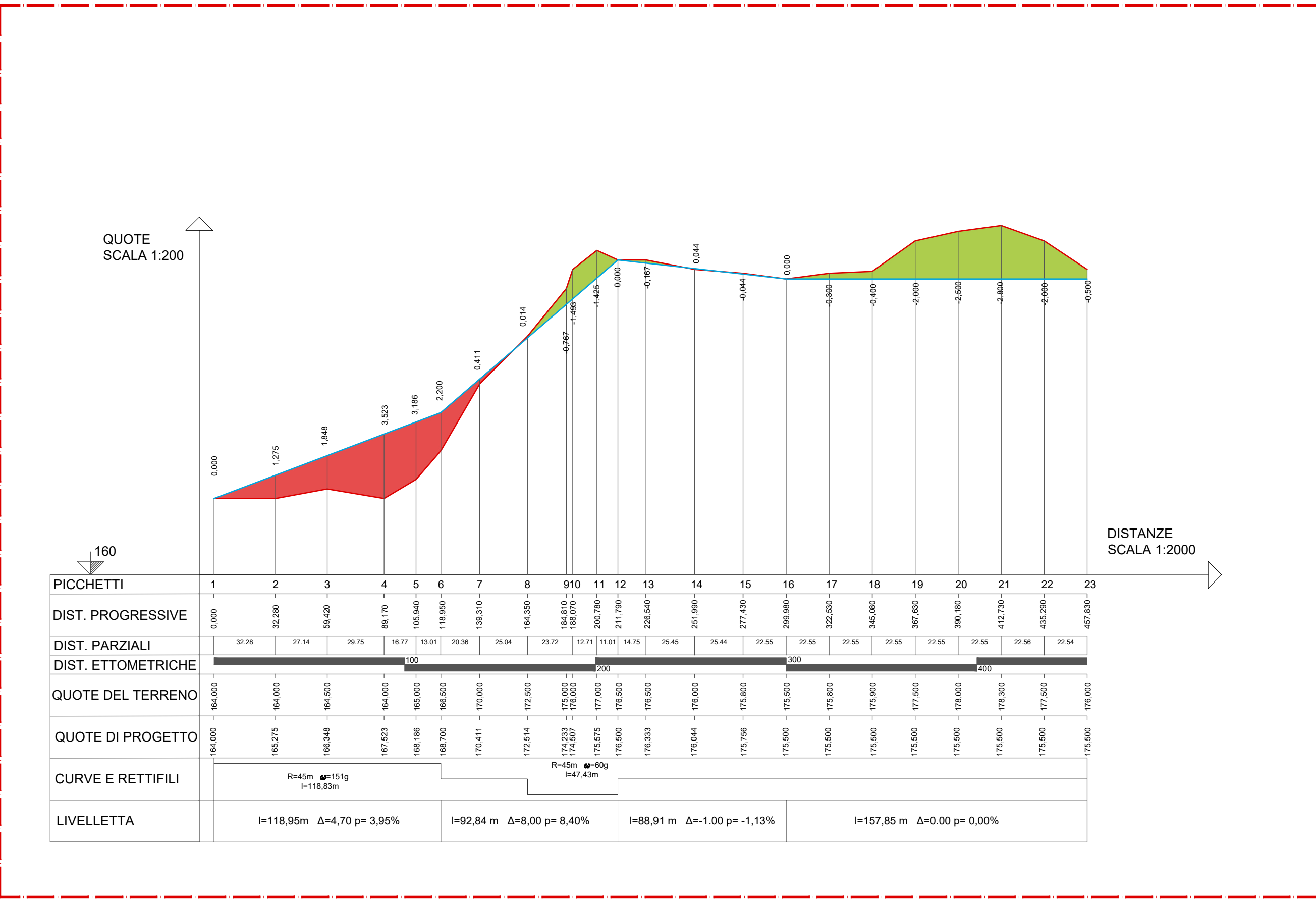
Profilo altimetrico WTG-B Scala 1:2.000
