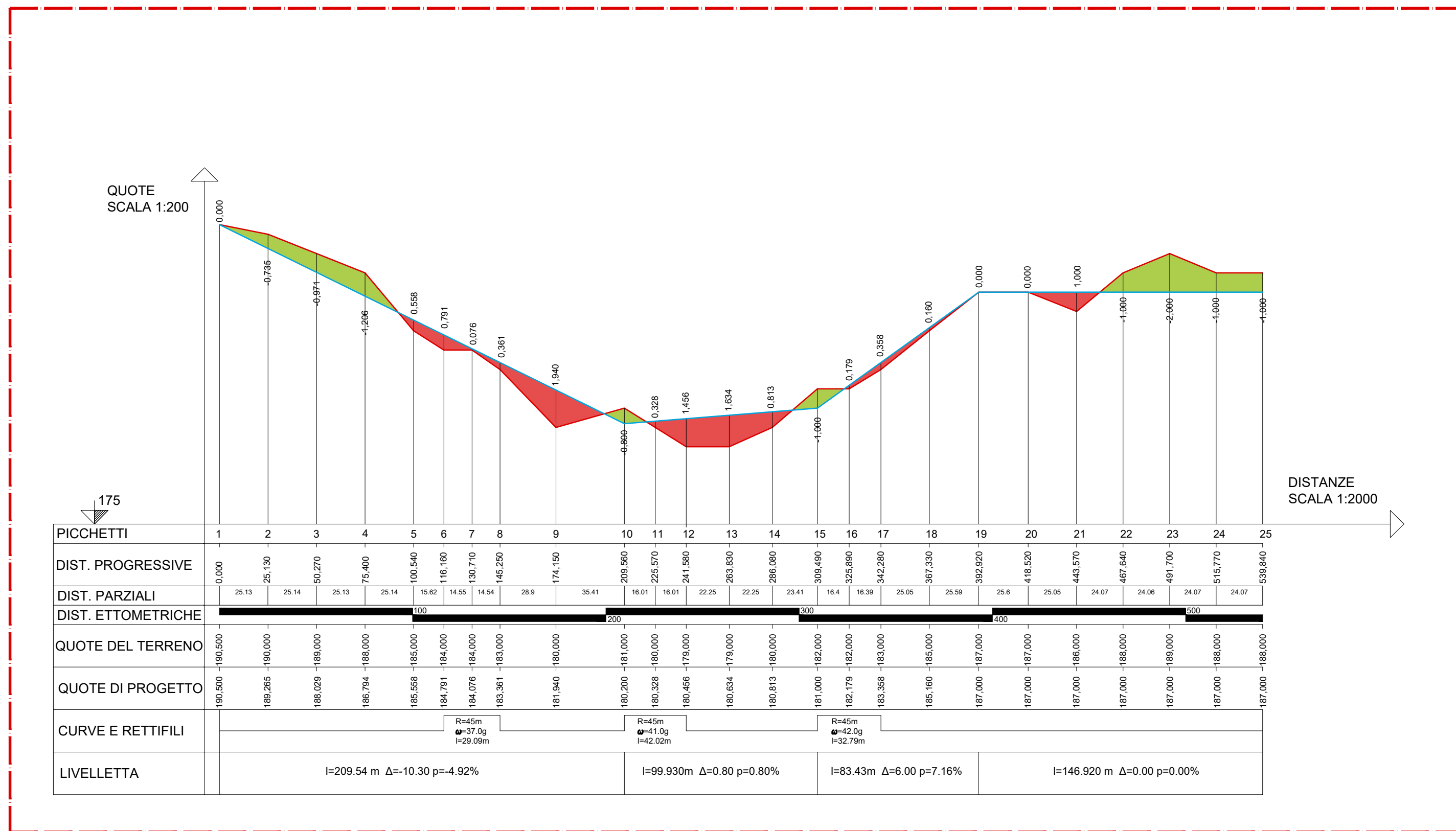
Profilo altimetrico WTG-0 Scala 1:2.000
