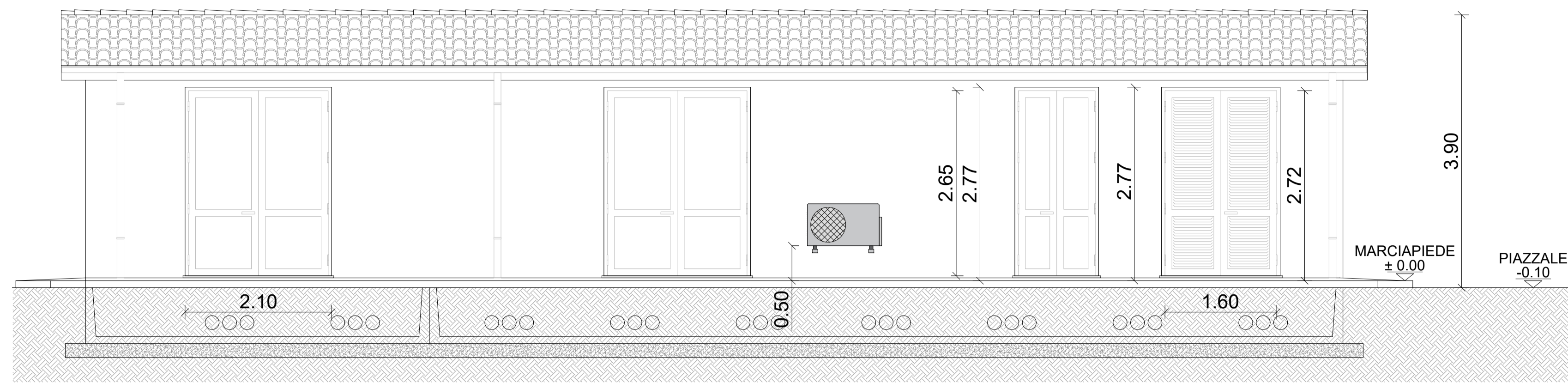
PROSPETTO A
