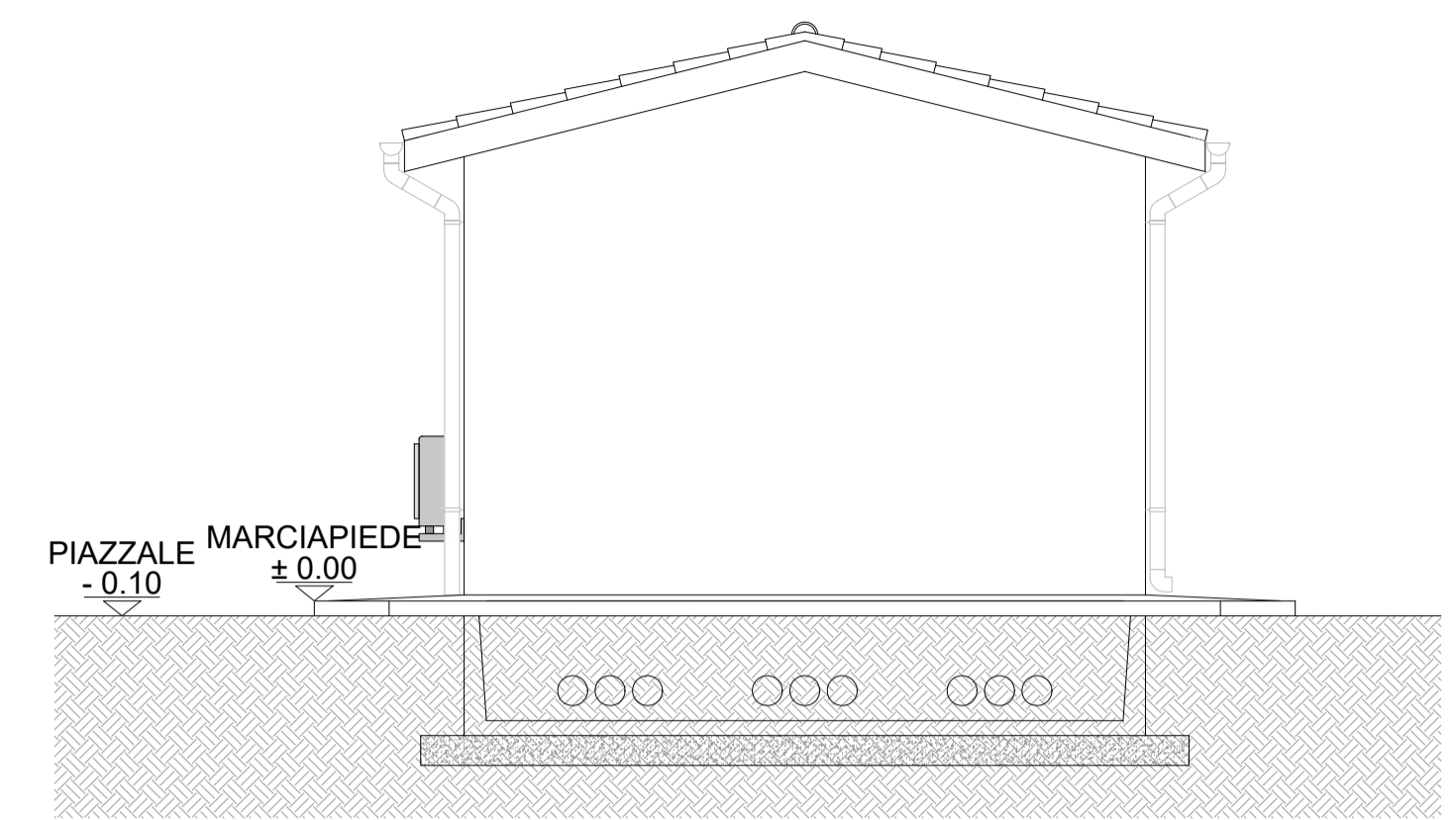
PROSPETTO D
