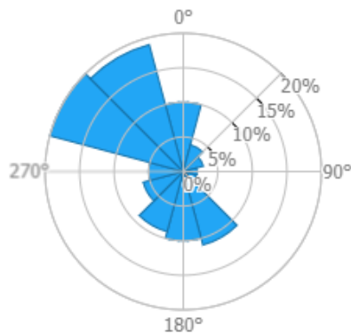
Figura 3: Frequenza del vento per direzione
