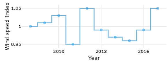
Figura 6– Varianza annua della ventosità media
