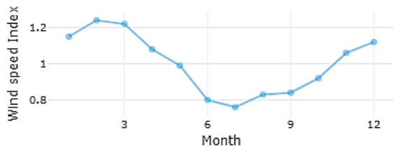
Figura 5 Stagionalità della ventosità media
