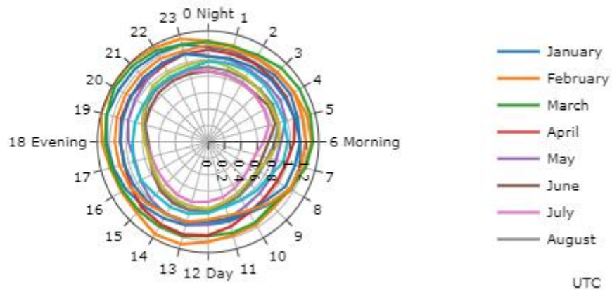
Figura 7 Scostamenti orari e stagionali dalla ventosità media
