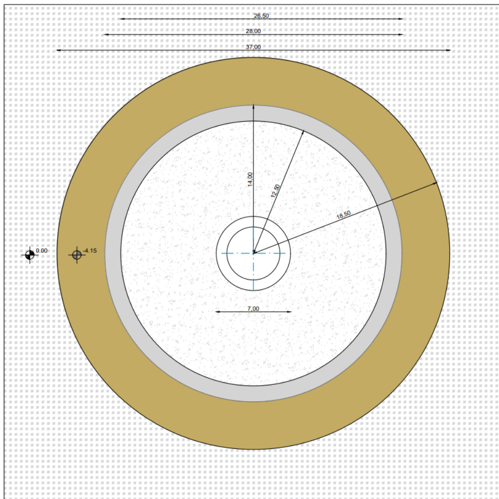
Figura 10 – Schemi plinto
