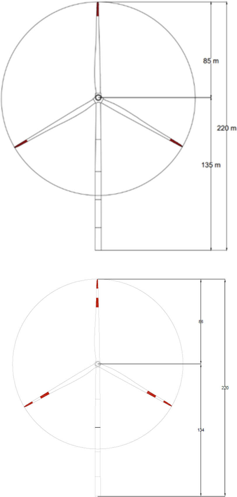
Figura 6 – Prospetti dell’aerogeneratore
