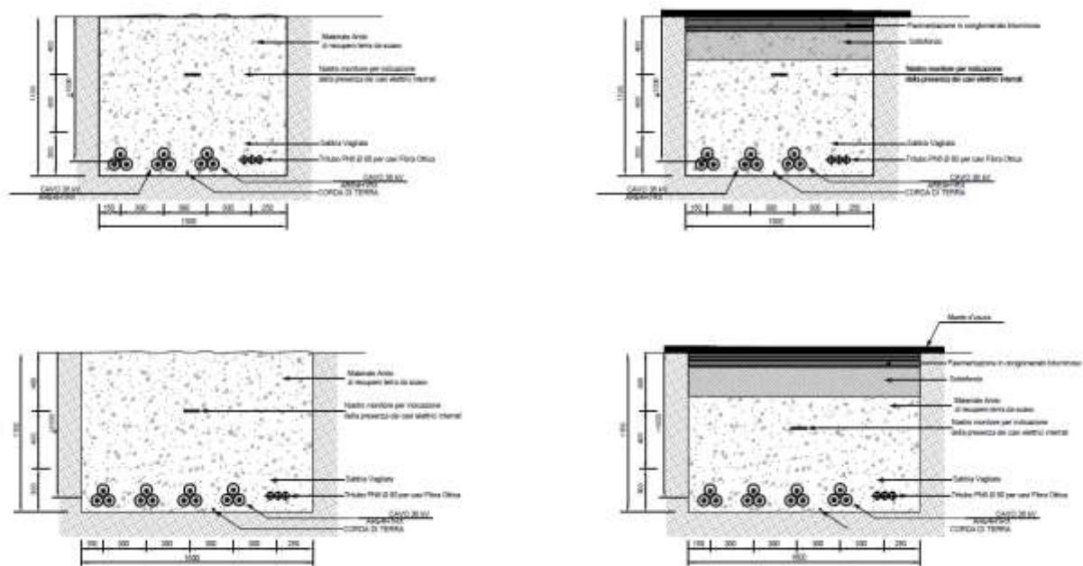
Figura 4-3: Cavidotti in progetto 36 kV con sezioni variabili da 50 a 300 mm 2
