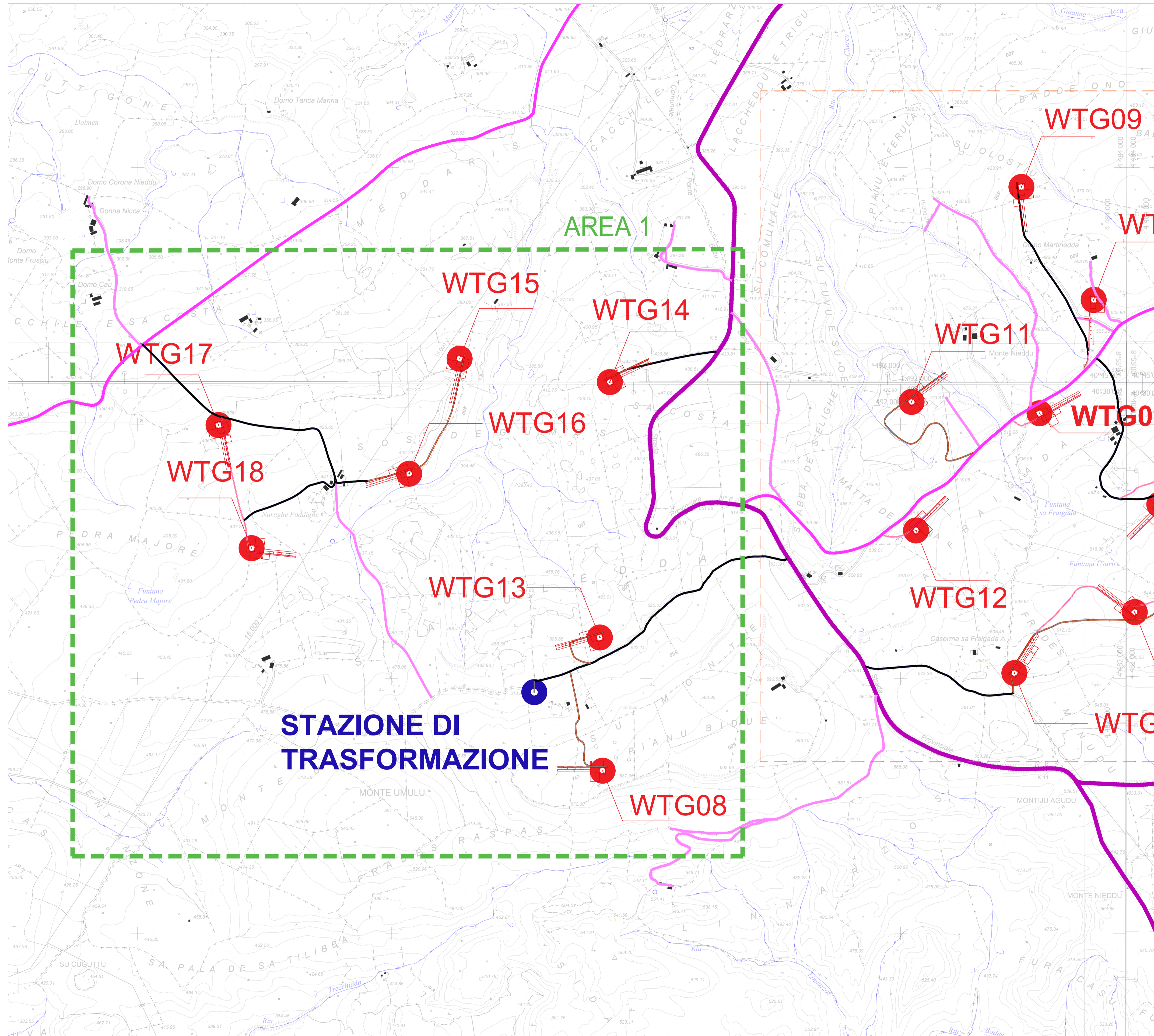
Planimetria generale
