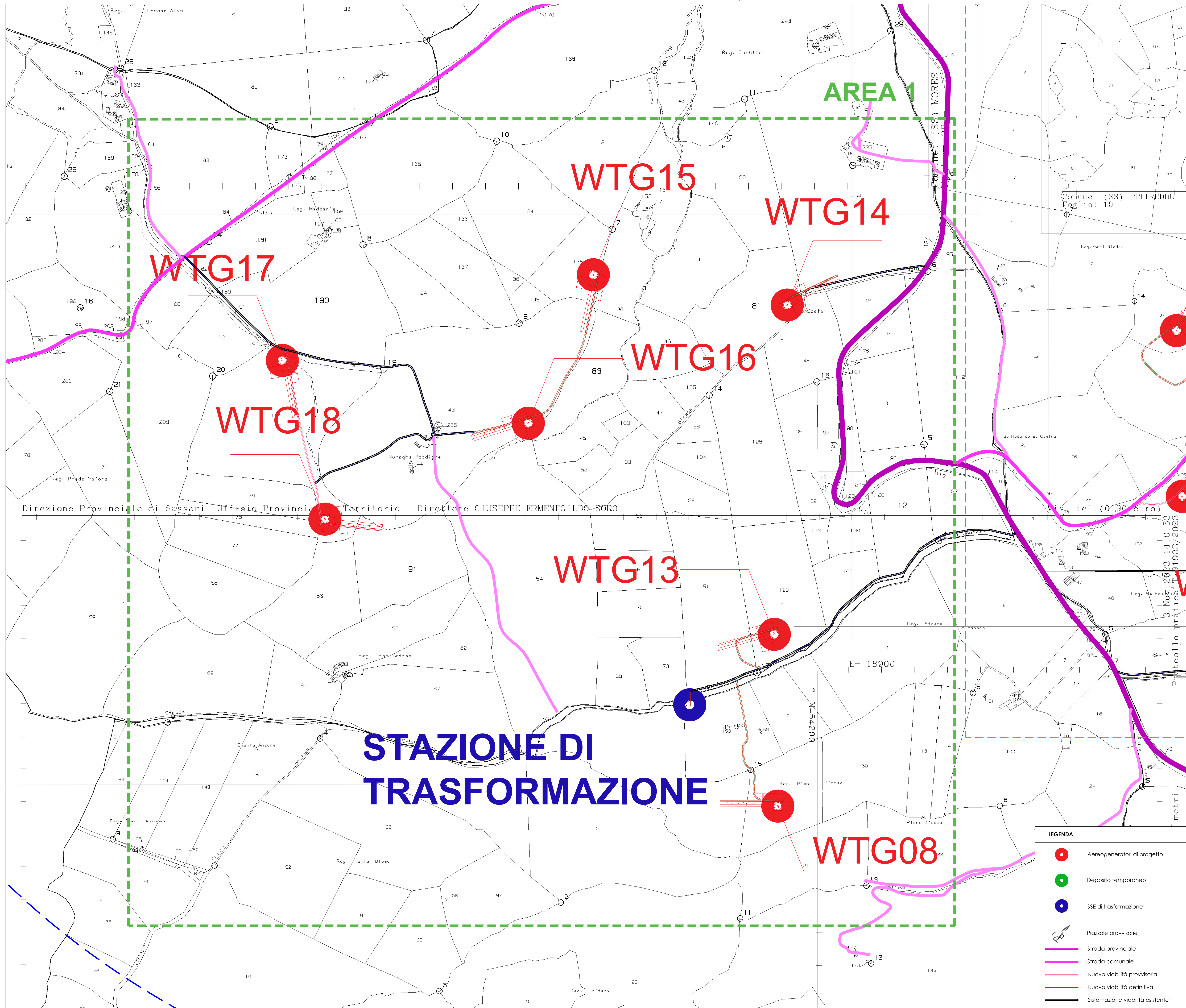
Planimetria con indicazione viabilità provvisoria e definitiva - Area 1
