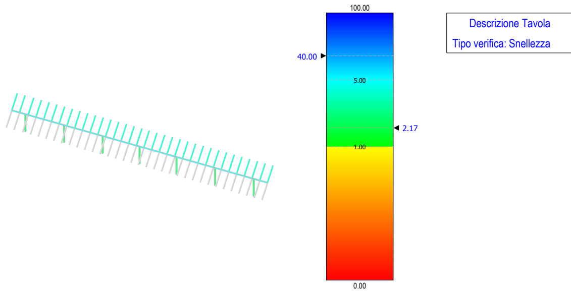
Figura 8: Verifica snellezza
