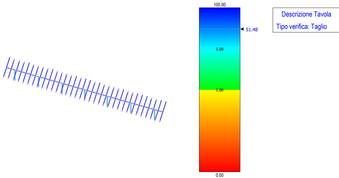
Figura 6: Verifica a taglio
