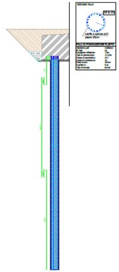
Pali di Fondazione - Lunghezza di infissione = 25m
