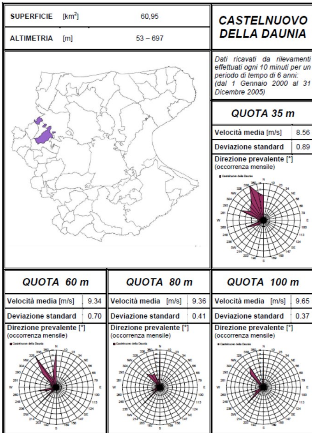
Figura21 Ventosità alle quote di 35-60-80-100 nel comune di Castelnuovo della Daunia (FG)-Università degli studi di Lecce-Progetto M.E.T.E.
