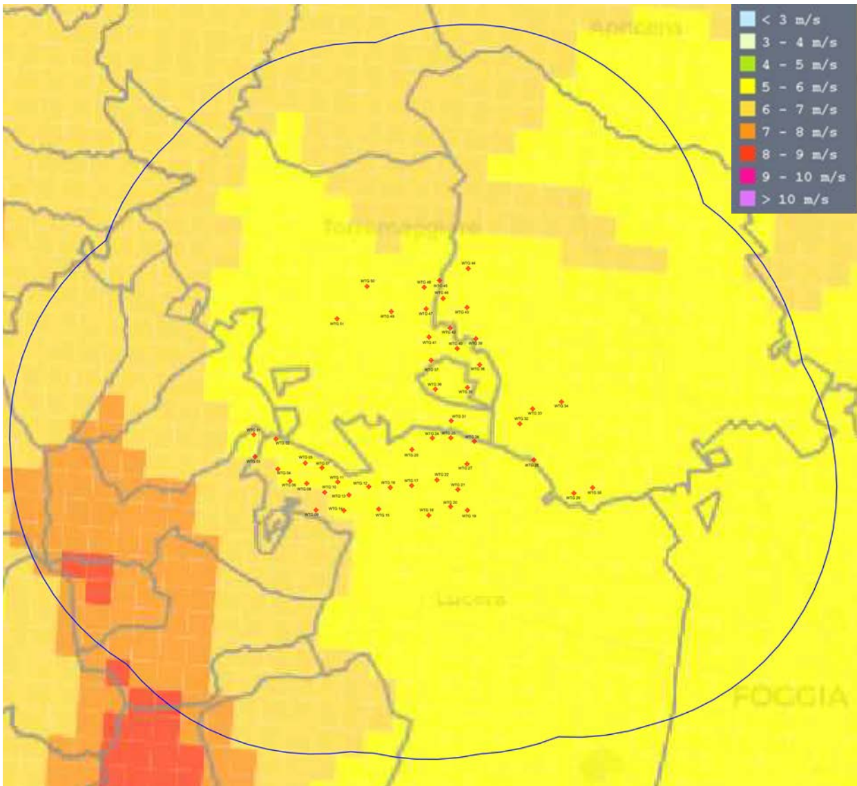
Impianto su Atlante eolico interattivo con velocità media annua del vento a 150 m s.l.m.
