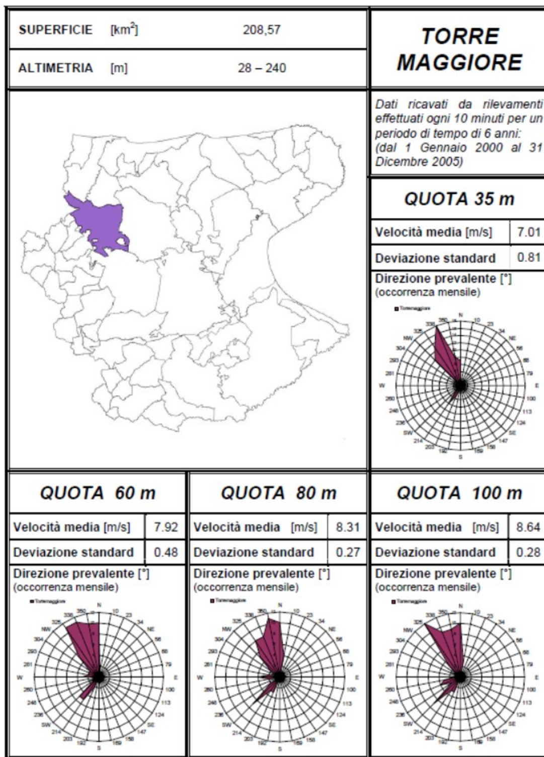
Figura 3 Ventosità alle quote di 35-60-80-100 nel comune di Torremaggiore (FG)-Università degli studi di Lecce-Progetto M.E.T.E.
