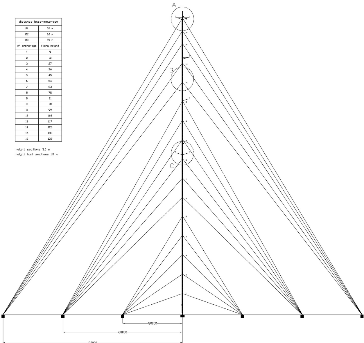
Torre anemometrica tipo
