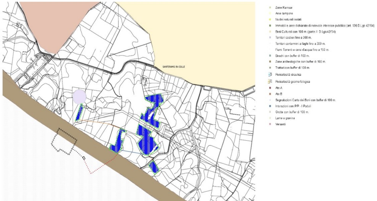
Figura 09: Area dell'impianto con segnalazione delle aree non idonee
