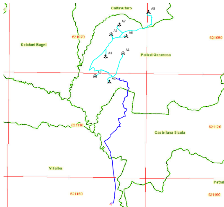
Figura 3 - Inquadramento area parco e sottostazione su CTR
