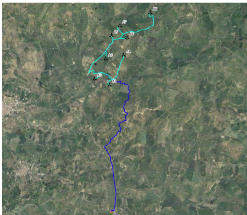
Figura 1 - Inquadramento area parco eolico su base ortofoto
