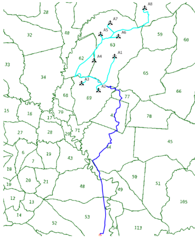
Figura 2 - Inquadramento area parco eolico su catastale
