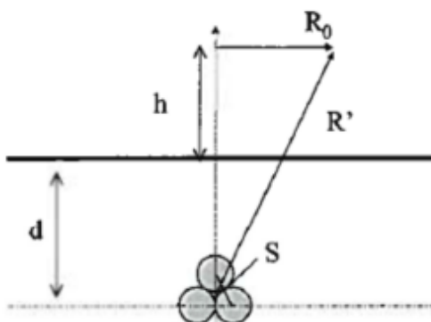
Figura 11 – Schema di principio per il calcolo delle distanze da terne di cavi interrati con posa a trifoglio oltre le quali l’induzione magnetica è inferiore all’obiettivo di qualità
