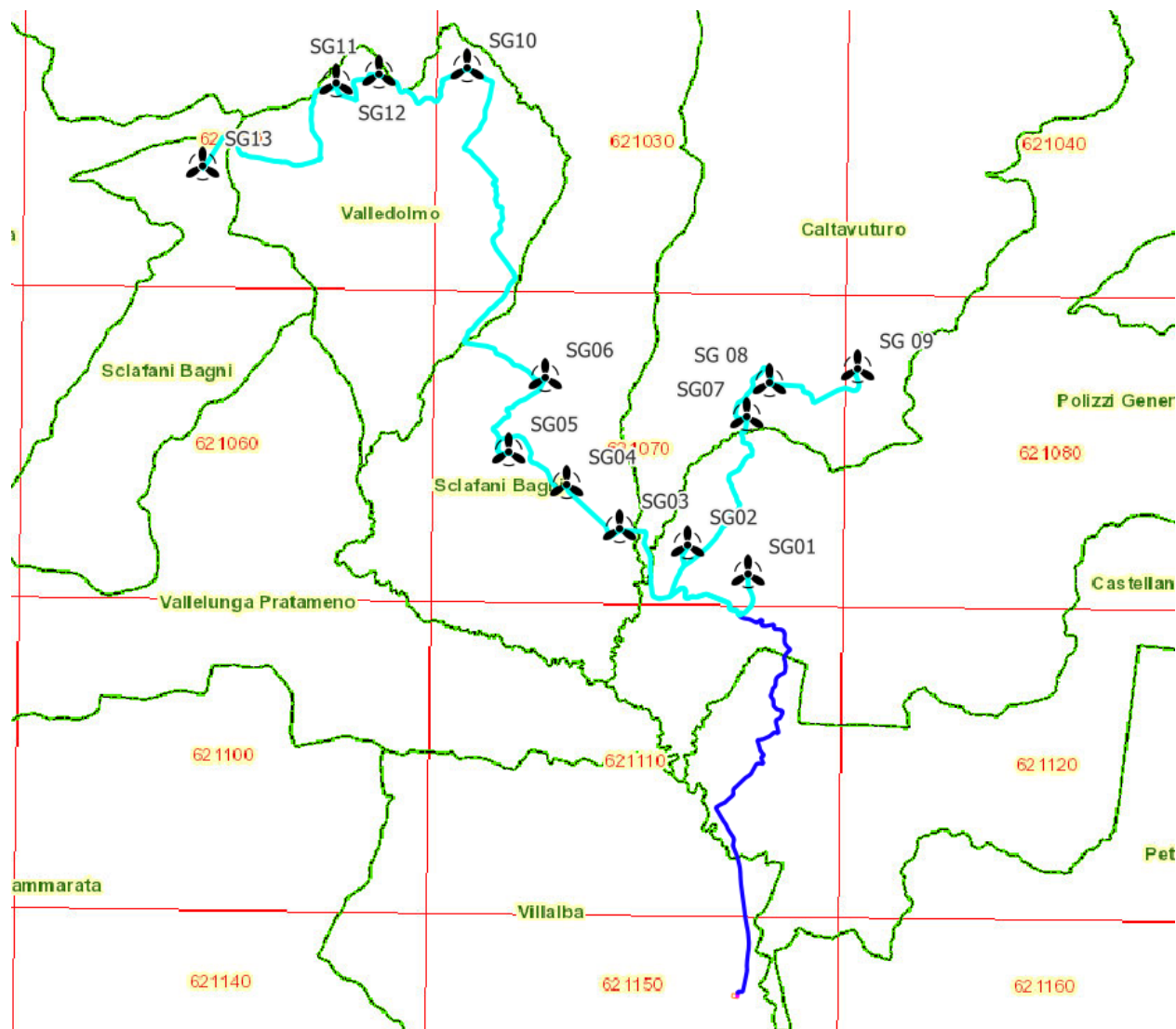
Figura 3 - Inquadramento area campo e sottostazione su CTR
