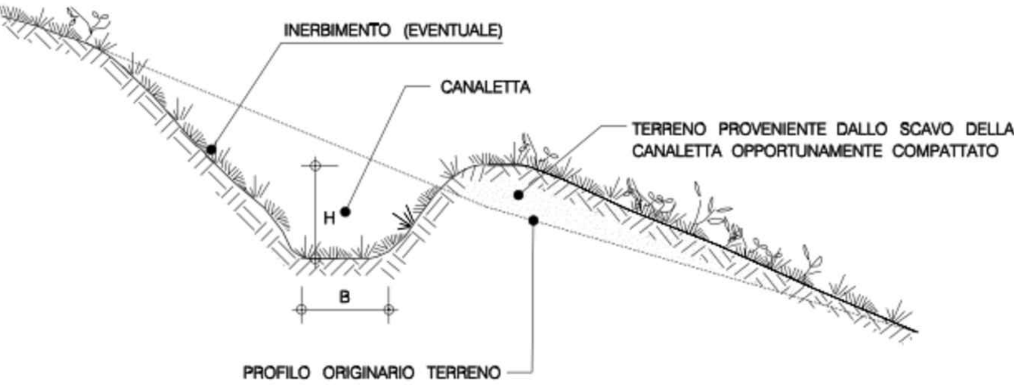
CANALET TA IN TERRA – TIPOLOGIA 1
