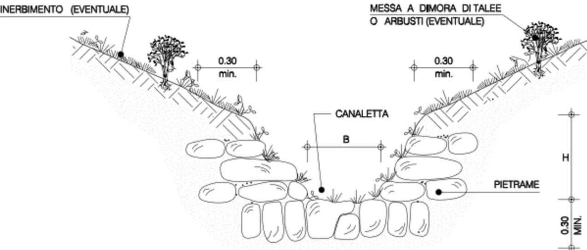
CANALET TA RIVESTITA CON PIETrame TIPOLOGIA 3
