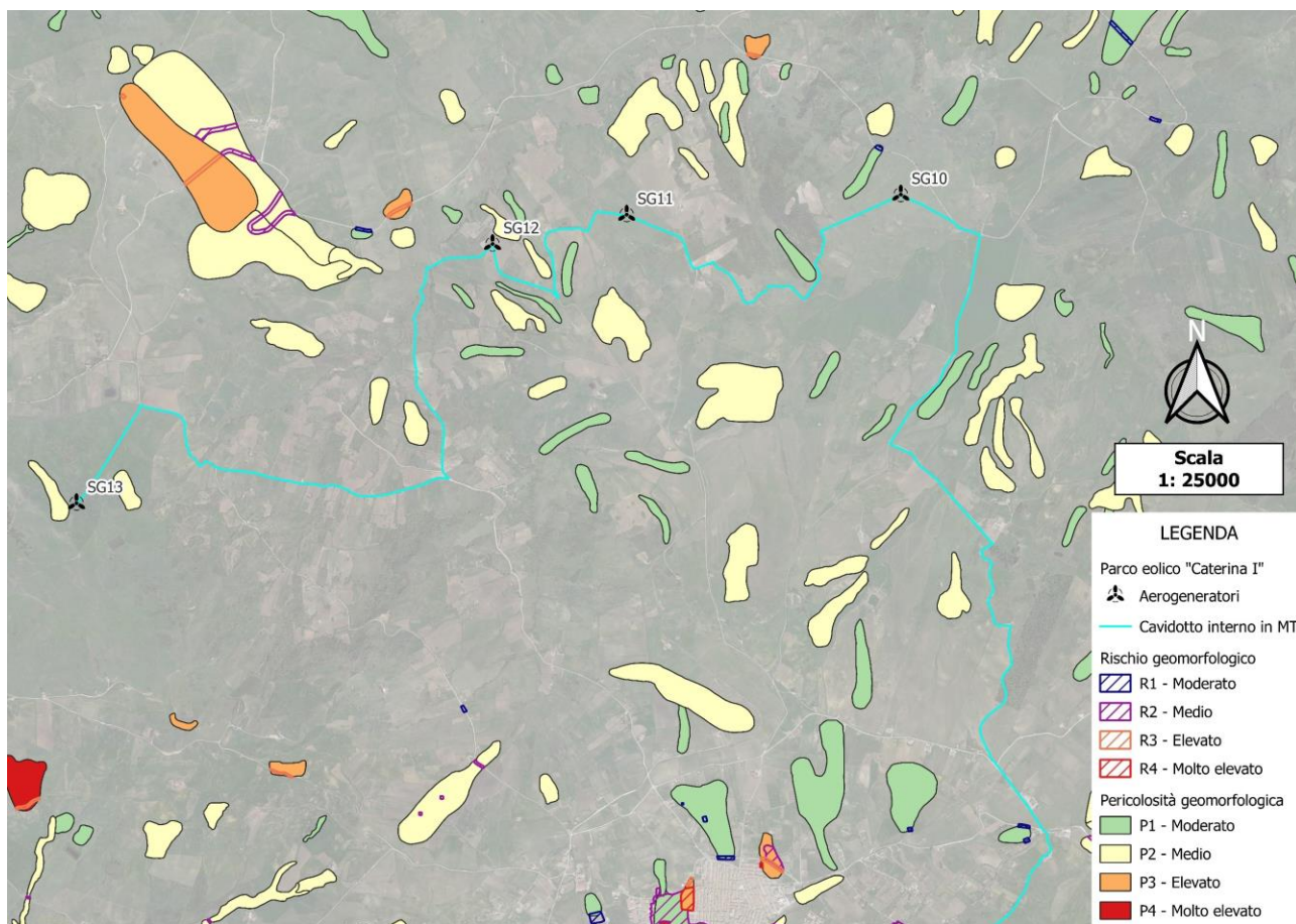
Figura 5: Stralcio della carta del rischio e della pericolosità Geomorfologica.
