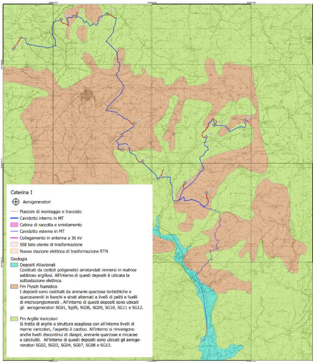
Figura 4: Stralcio della Carta Geologica.
