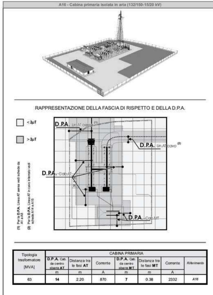
Figura 18 - Scheda A16 - Dpa per cabina primaria
