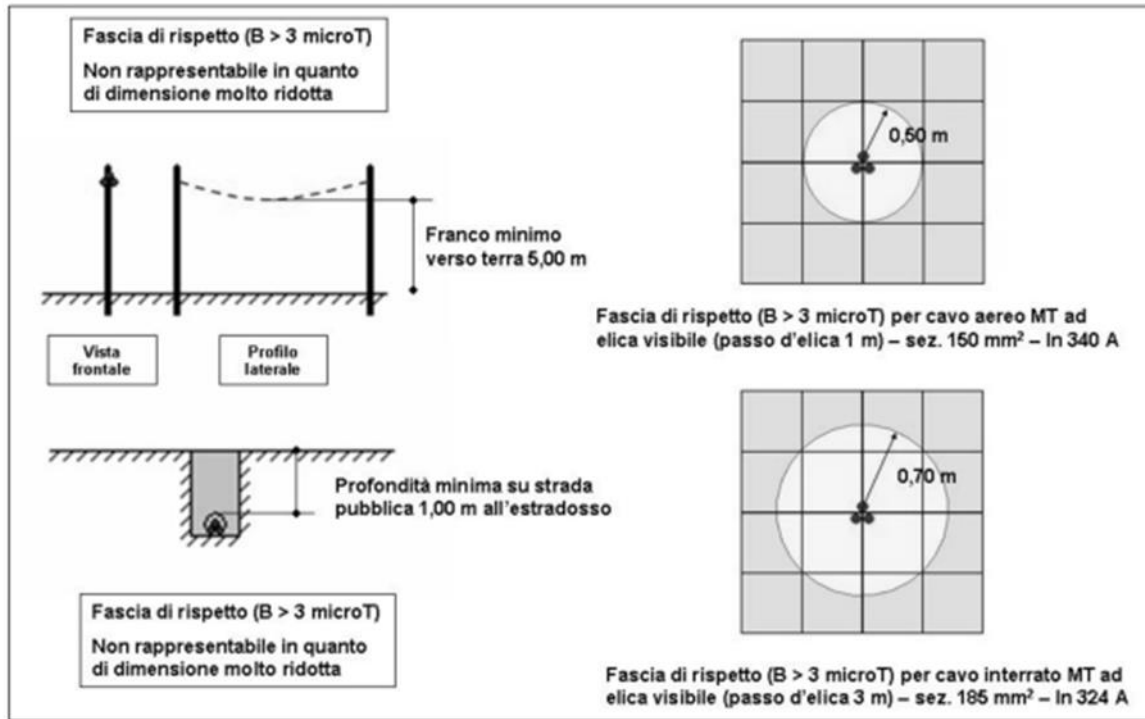
Figura 14 – Curve di livello dell'induzione magnetica generata da cavi cordati ad elica
