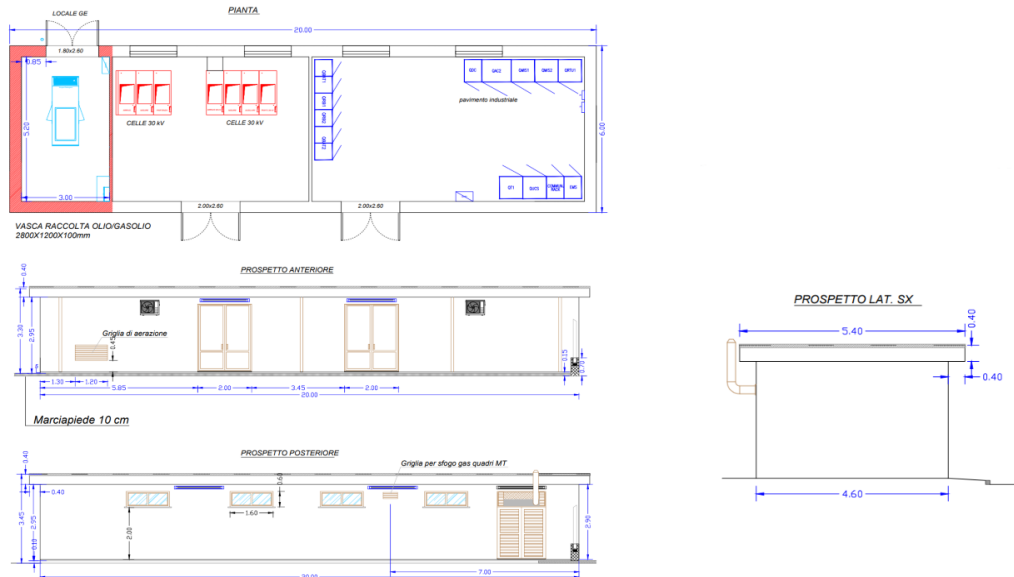
Figura 7 - Tipico Cabina di Raccolta e Smistamento
