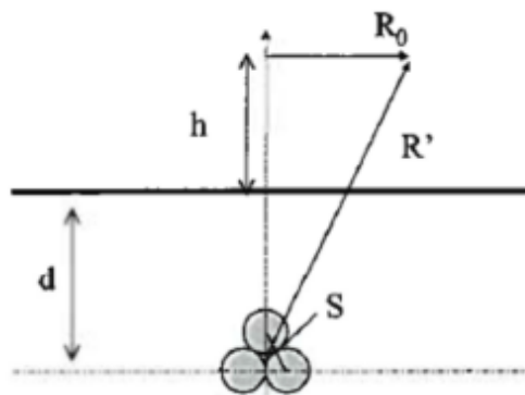
Figura 16 – Schema di principio per il calcolo delle distanze da terne di cavi interrati con posa a trifoglio oltre le quali l’induzione magnetica è inferiore all’obiettivo di qualità
