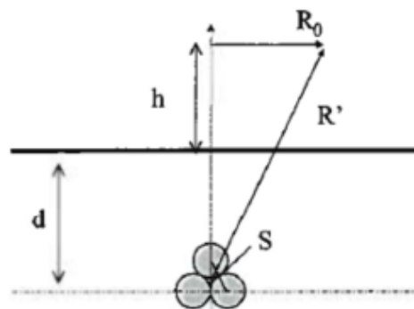
Figura 17 – Schema di principio per il calcolo delle distanze da terne di cavi interrati con posa a trifoglio oltre le quali l’induzione magnetica è inferiore all’obiettivo di qualità
