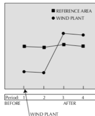
Figura 11 - Stime puntuali di un indicatore di impatto in un disegno idealizzato di BACI su quattro periodi di tempo con una leggera indicazione di recupero dopo l'impatto.
