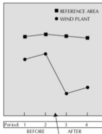
Figura 11 - Stime puntuali di un indicatore di impatto in un disegno idealizzato di BACI su quattro periodi di tempo con una leggera indicazione di recupero dopo l'impatto.
