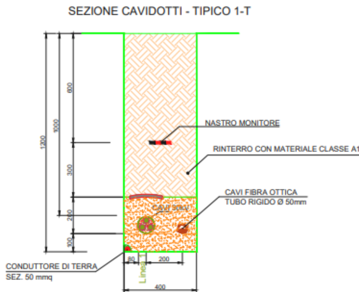
Figura 12- Sezione di scavo elettrodotto su terreno
