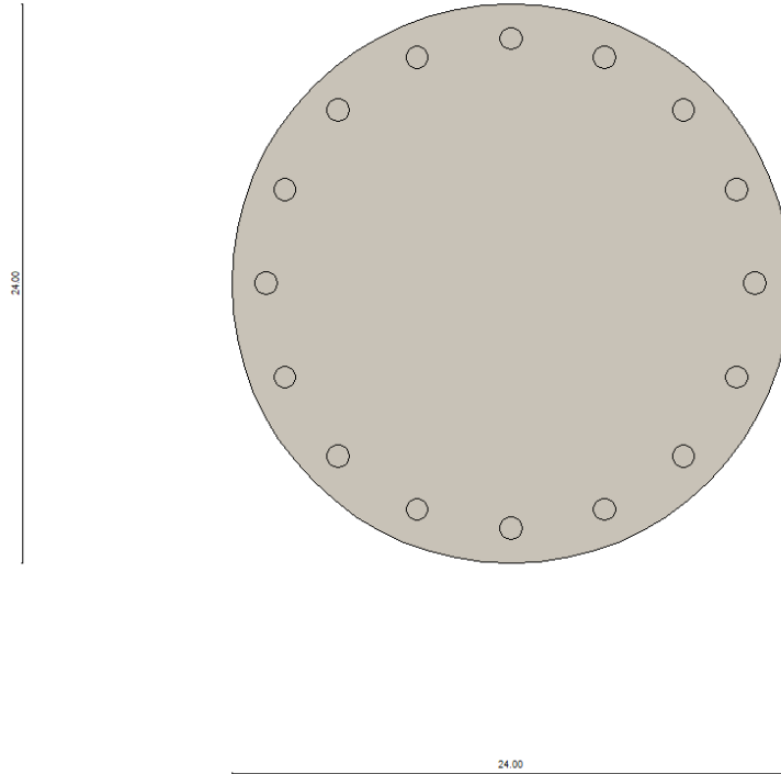
Figura 8- Pianta fondazione
