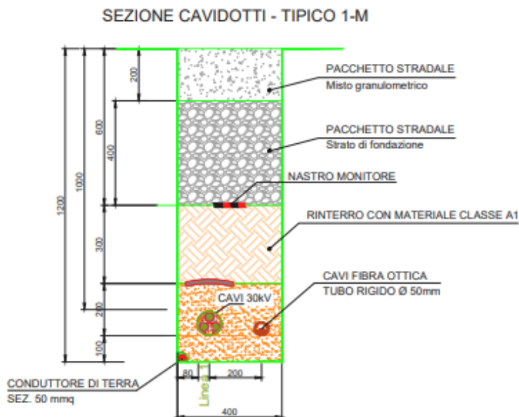
Figura 11- Sezione di scavo elettrodotta su strada sterrata
