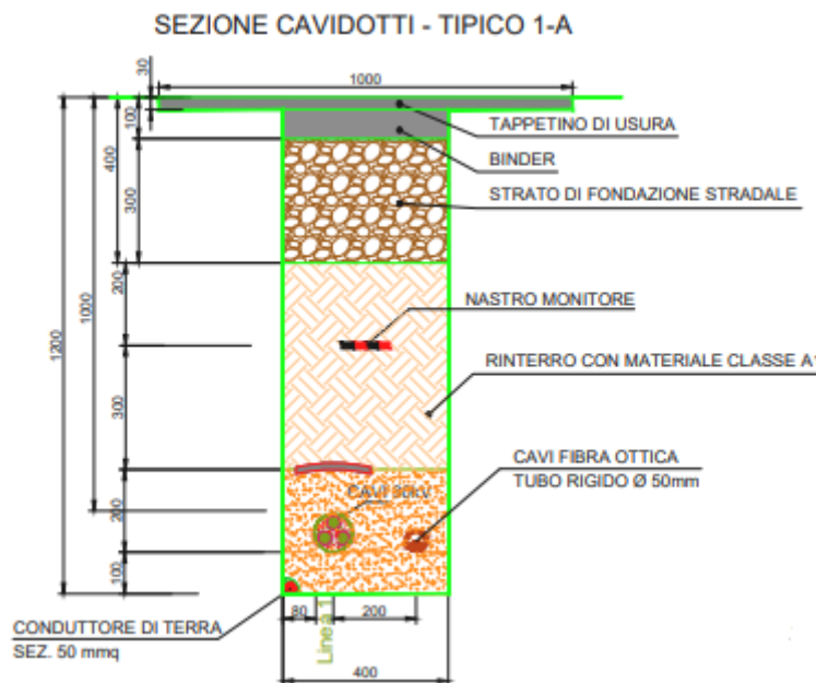
Figura 10- Sezione di scavo elettrodotta su strada asfaltata
