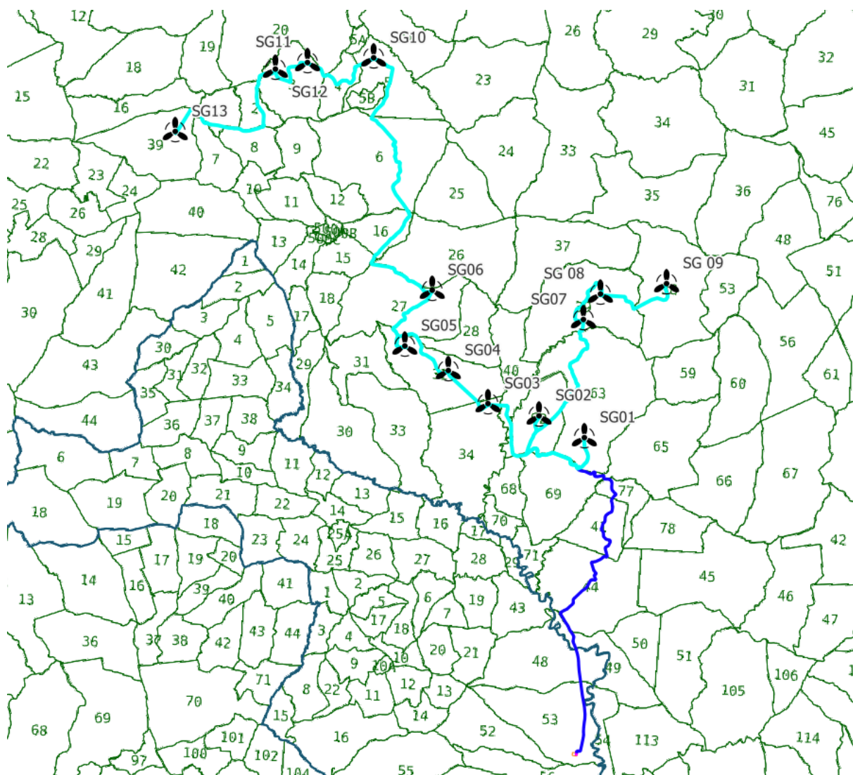
Figura 4: Layout di impianto (catastale)
