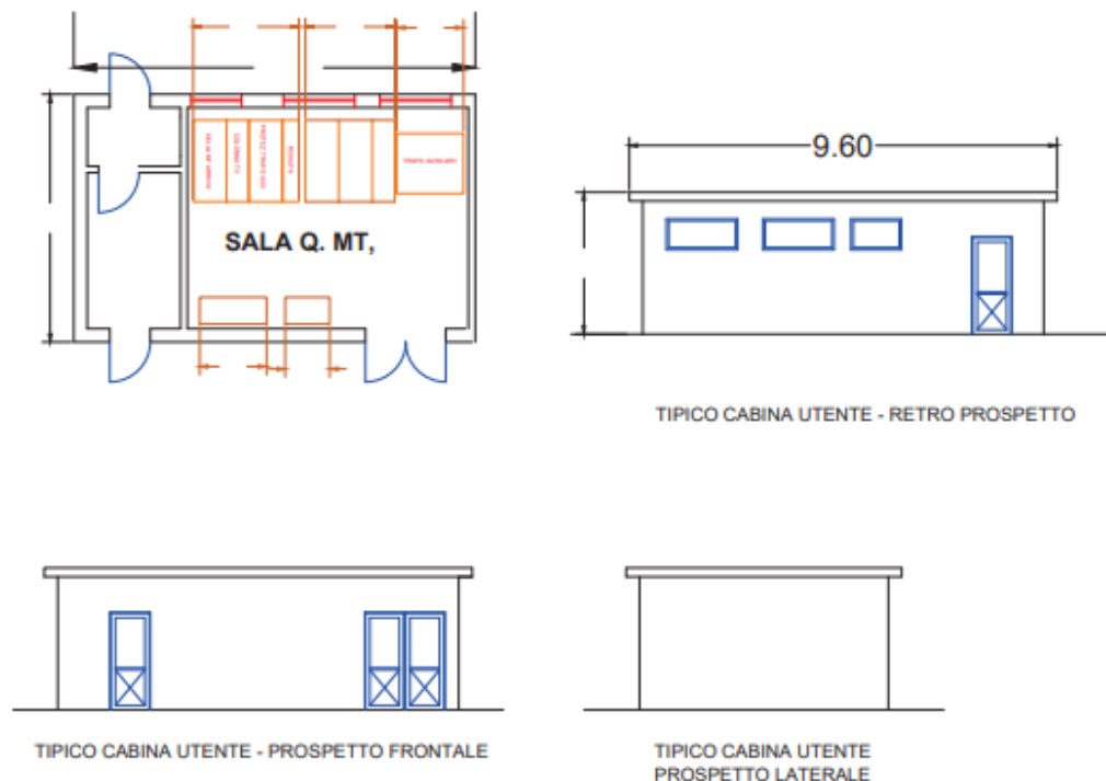
Figura 14- Particolare SSE Lato Utente Genzano
