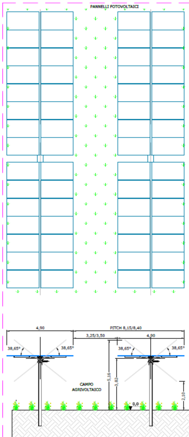
Fig. 2 – Piantumazione tra le file di tracker
