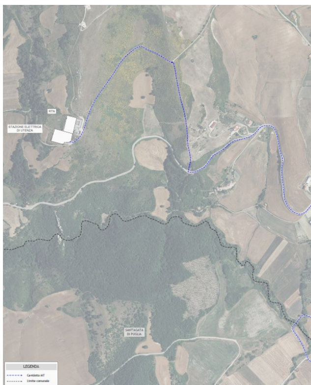
Figura 2 – Stralcio della planimetria con individuazione dell'impianto eolico esistente "Impianto Piano d'Olivola" su ortofoto
