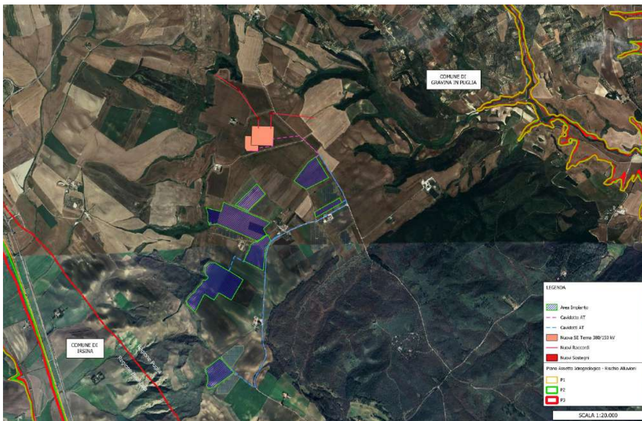
Figura 2-2: (Tav ALL_08.2) Estratto del Piano stralcio per la difesa dal rischio idrogeologico - Rischio alluvioni nell'area di intervento e layout di progetto
