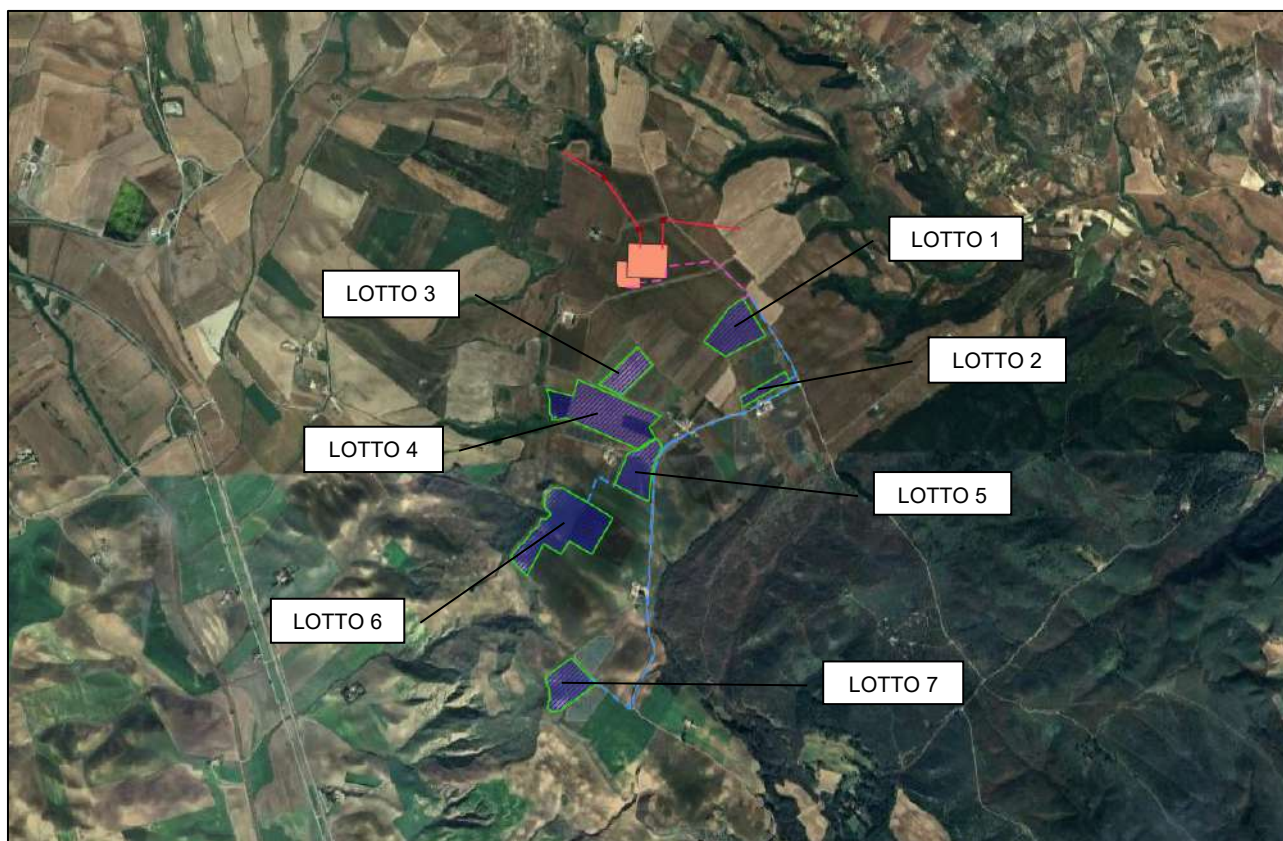
Figura 3-1: Inquadramento dei lotti di impianto
