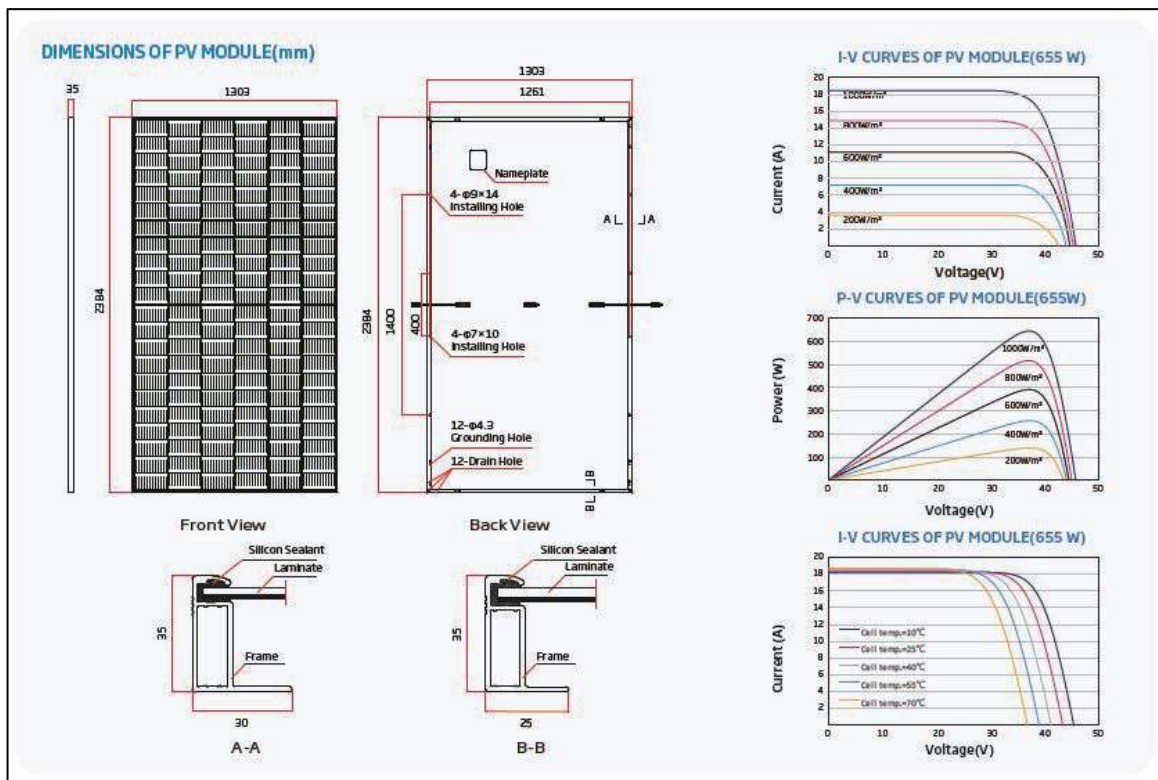
Figura 3-5: Scheda tecnica moduli
