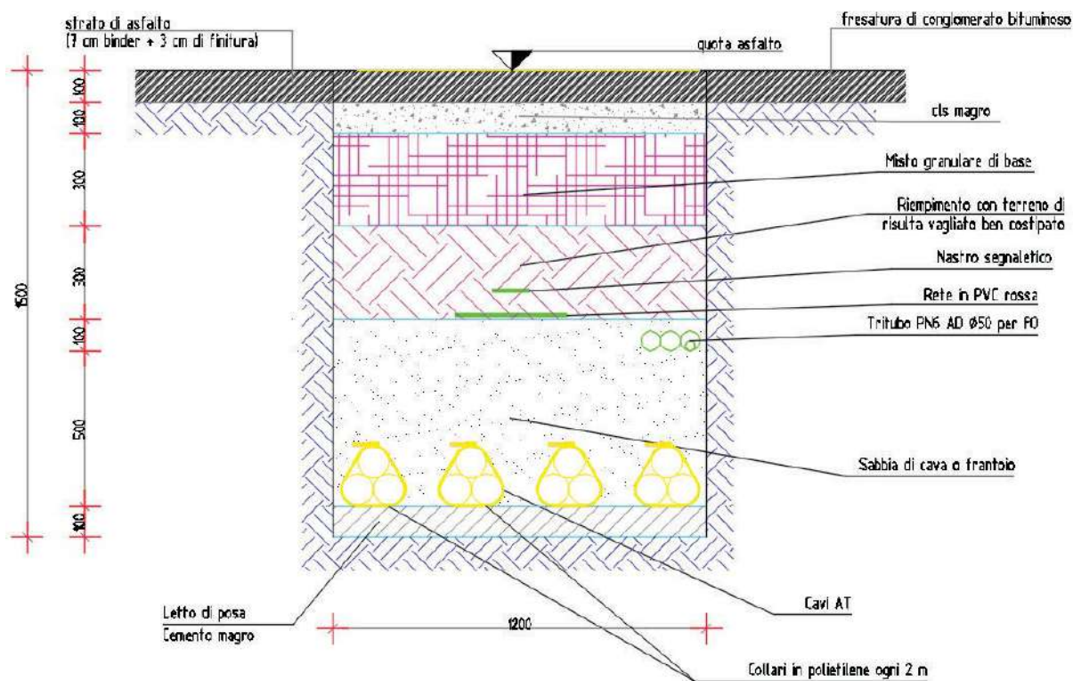
Figura 3-10: Sezione tipica di posa della linea in cavo su strade asfaltate
