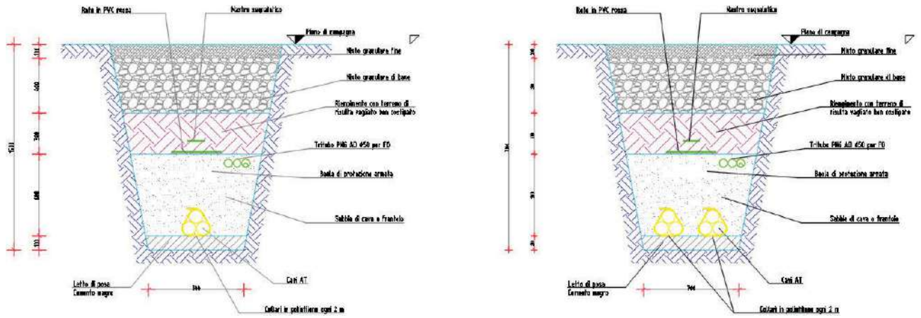
Figura 3-8: Sezione tipica di posa della linea in cavo su strade sterrate (1 e 2 terne)
