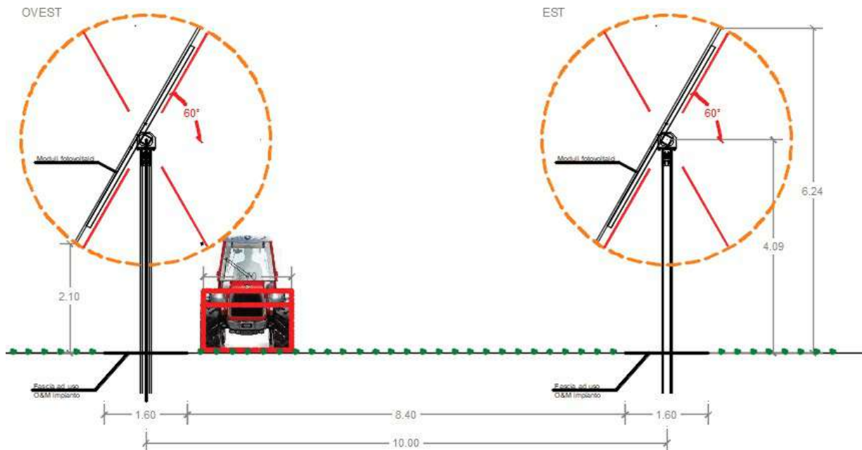
Figura 3-3: Sistema agri-voltaico – Verifica della compatibilità del sistema in fase di semina
