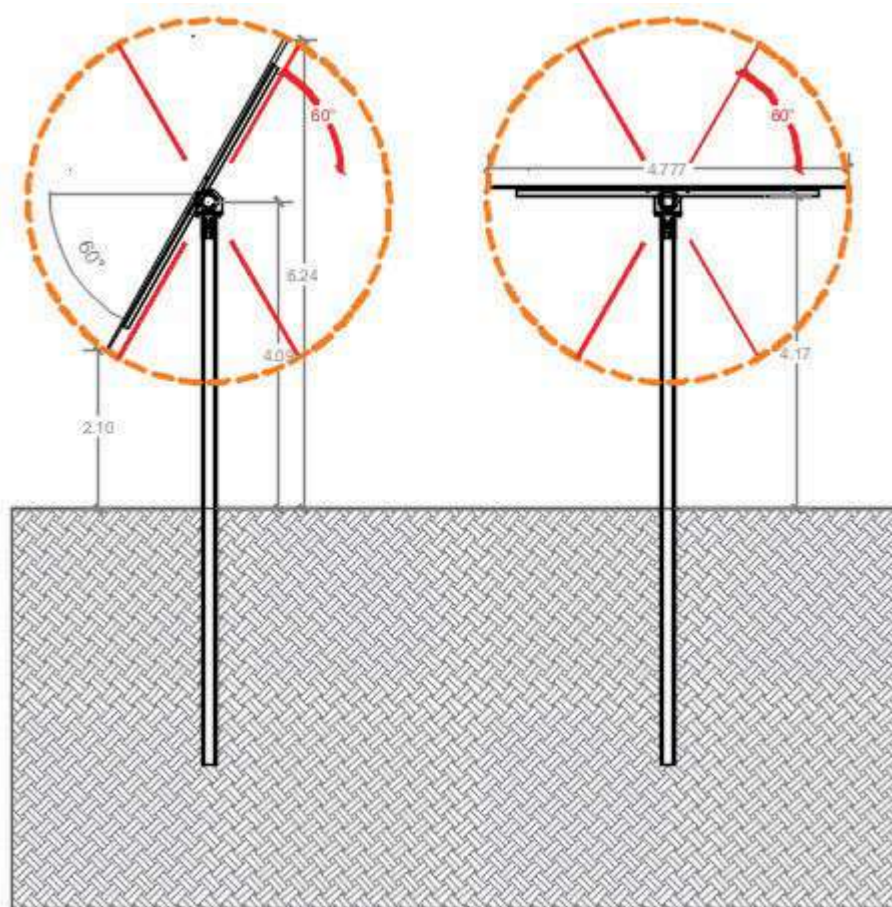
Figura 3-8: Sezione tipo struttura porta pannelli
