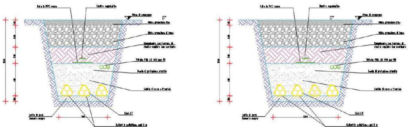
Figura 3-9: Sezione tipica di posa della linea in cavo su strade sterrate (3 e 4 terne)
