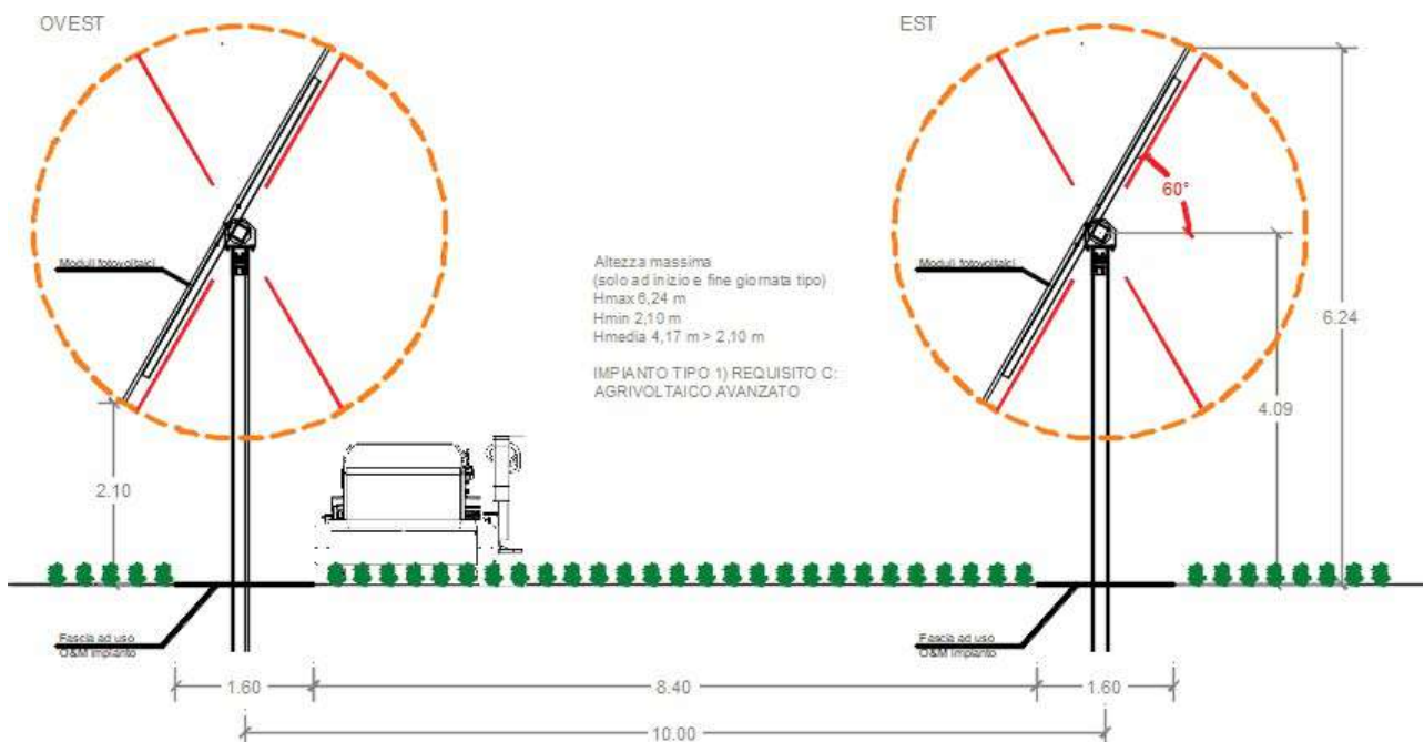
Figura 3-4: Sistema agri-voltaico – Verifica della compatibilità del sistema in fase di raccolta
