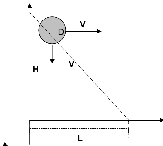
Figura 4-9: Schema di caduta della particella solida
