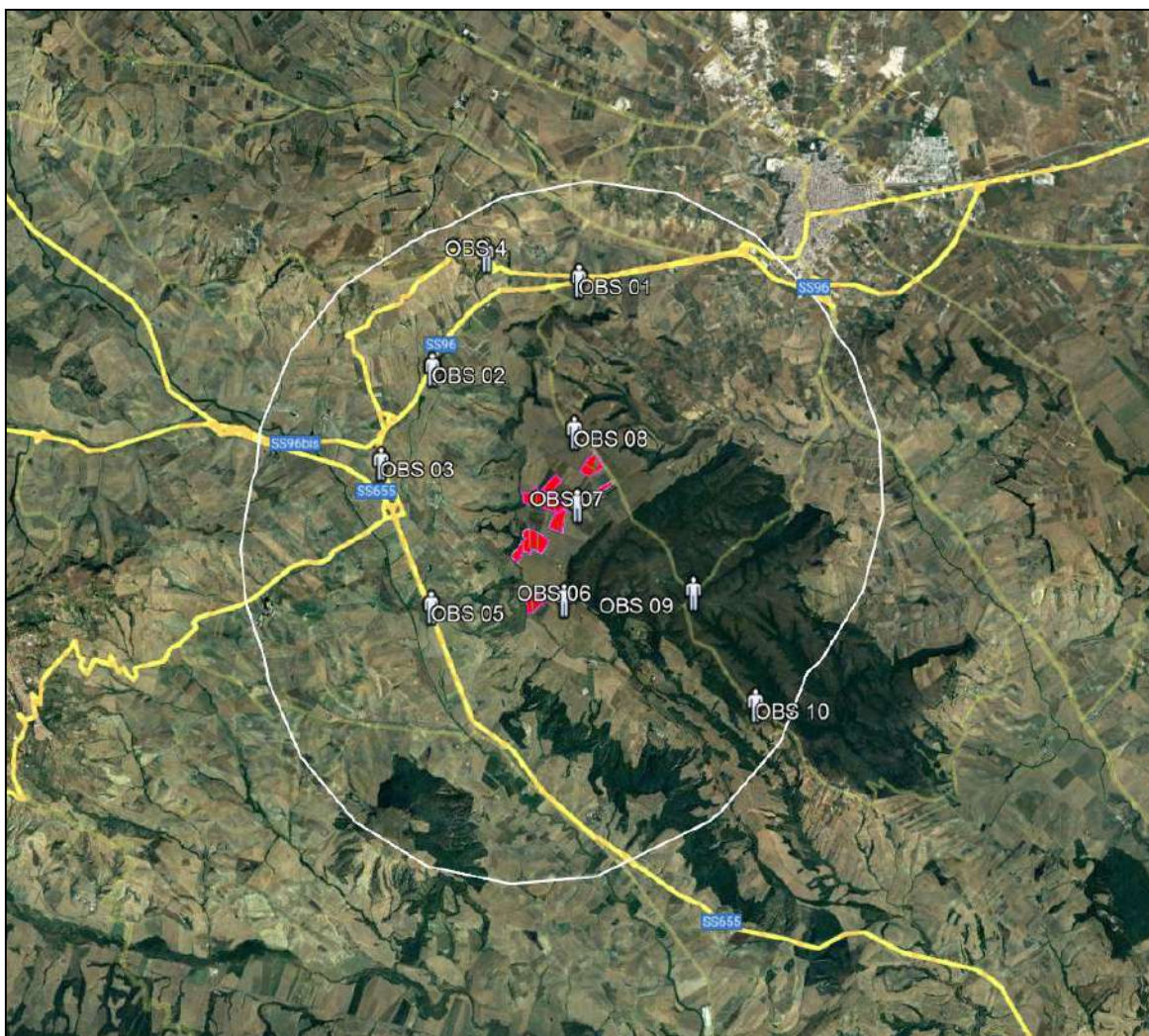
Figura 6-4: Ubicazione Osservatori
