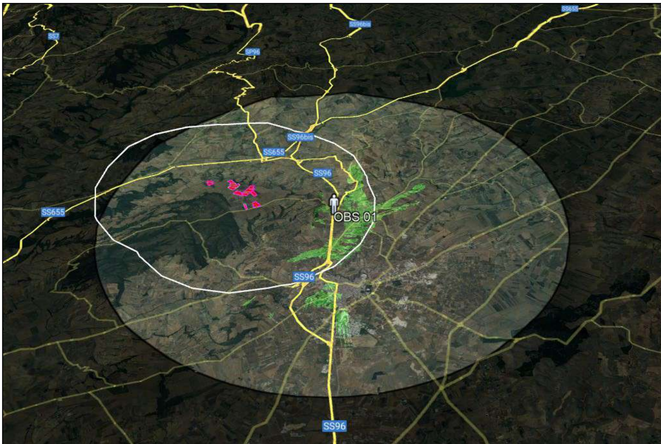
Figura 6-5: OSSERVATORE 1: Area di visibilità teorica
