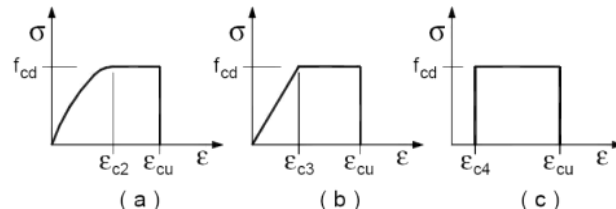
Diagrammi di progetto tensione – deformazione del calcestruzzo.
