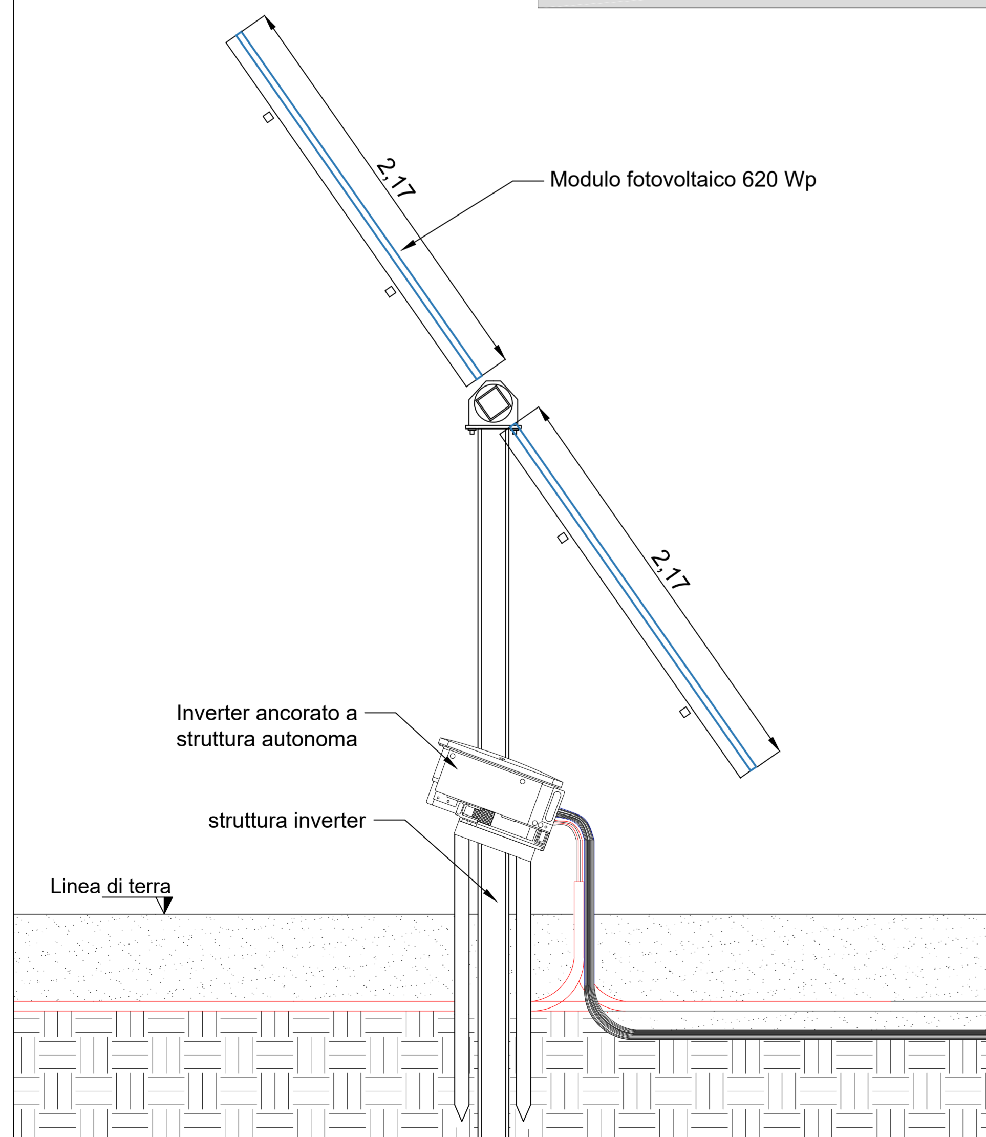
Particolare struttura inverter - Scala 1:20
