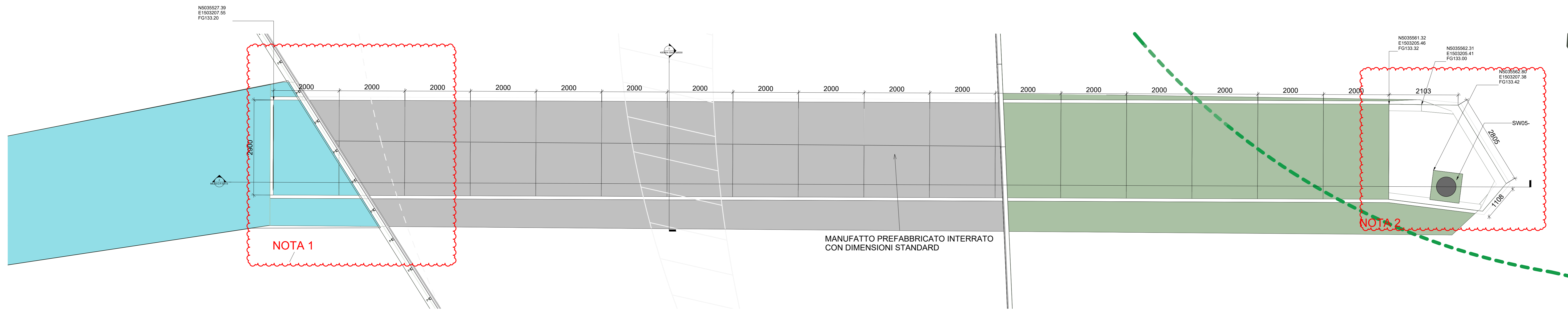
1 PIANTE CAMERETTA E BOX PREFABBRICATI INTERRATI 1 : 50
