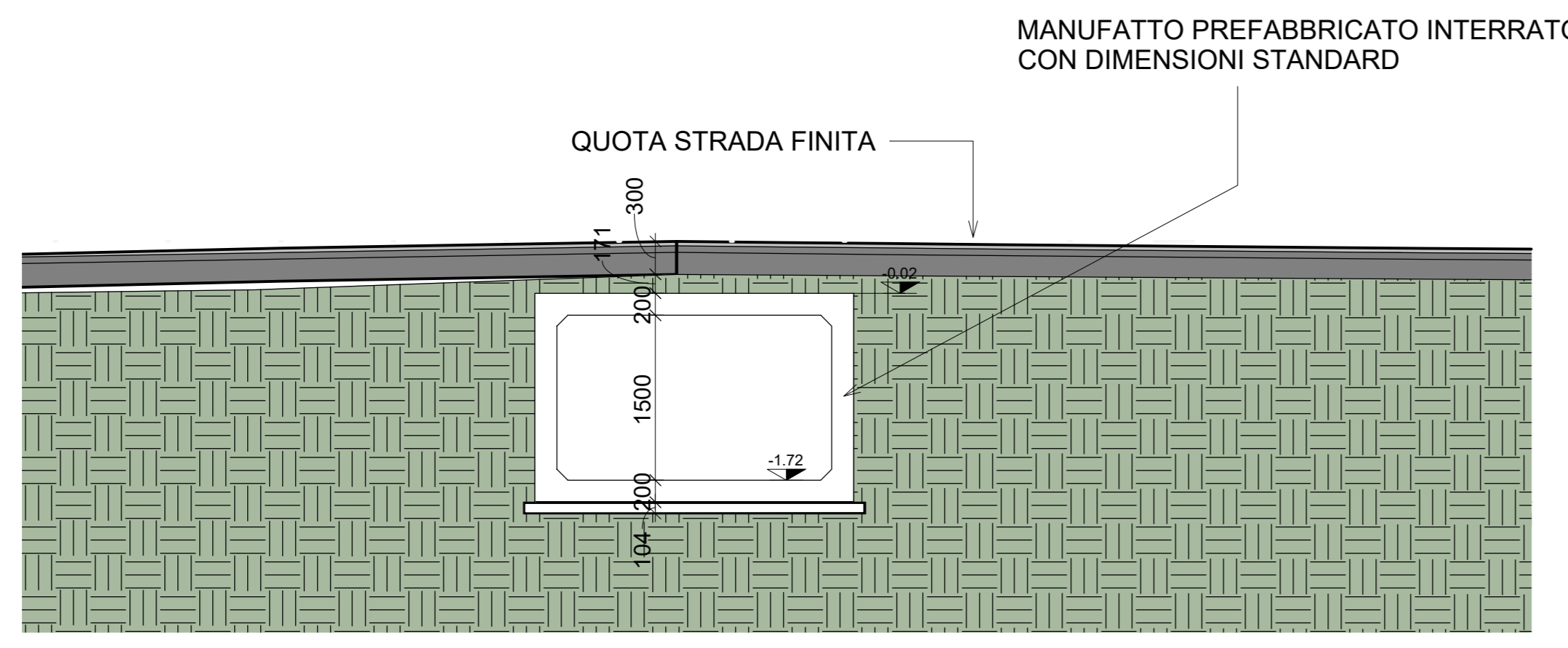
3 Sezione 3 1 : 50
