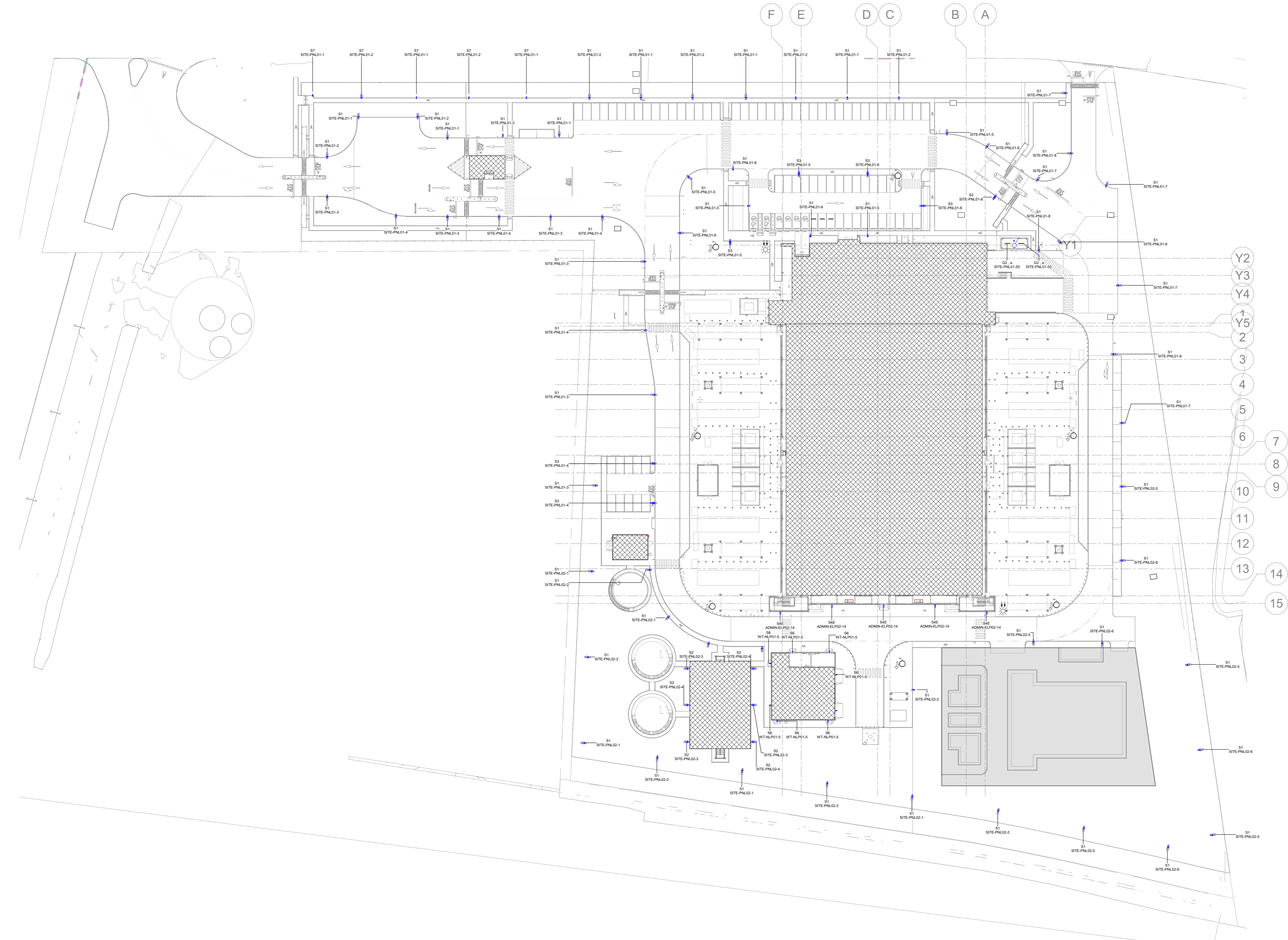
1 PLANIMETRIA AREE ESTERNE - IMPIANTO DI ILLUMINAZIONE 1 : 500
