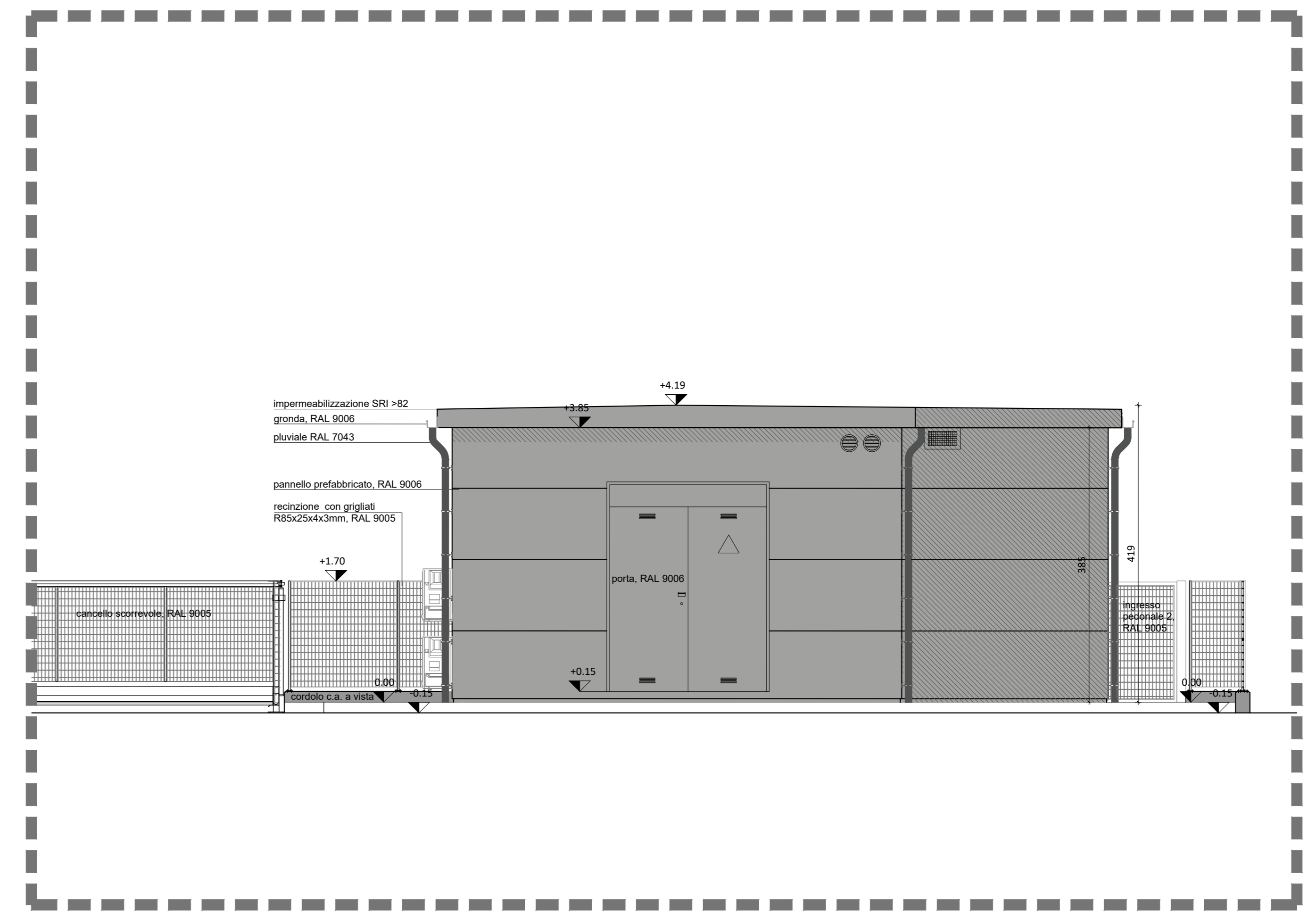
Prospetto nord
