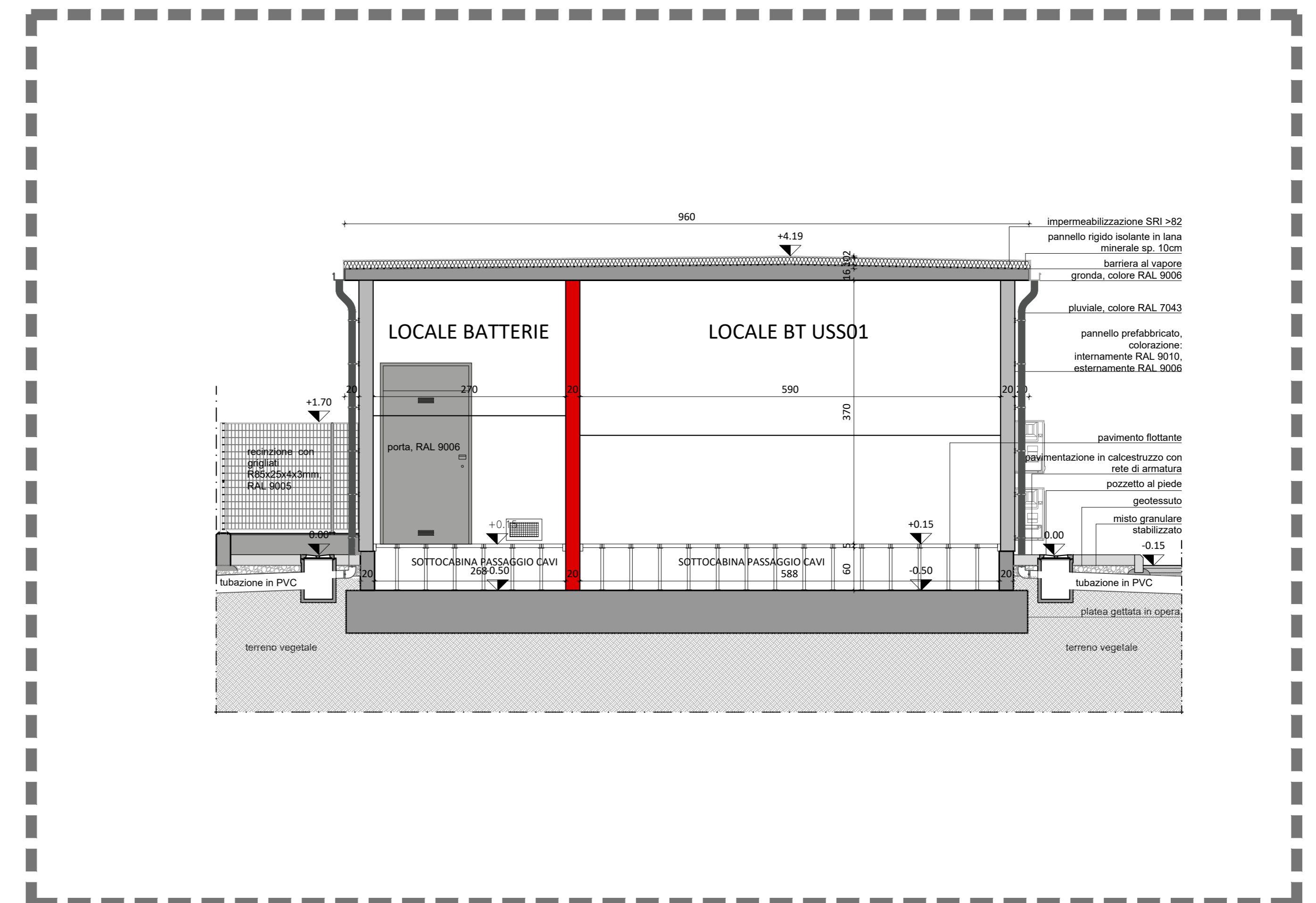
Sezione B - B
