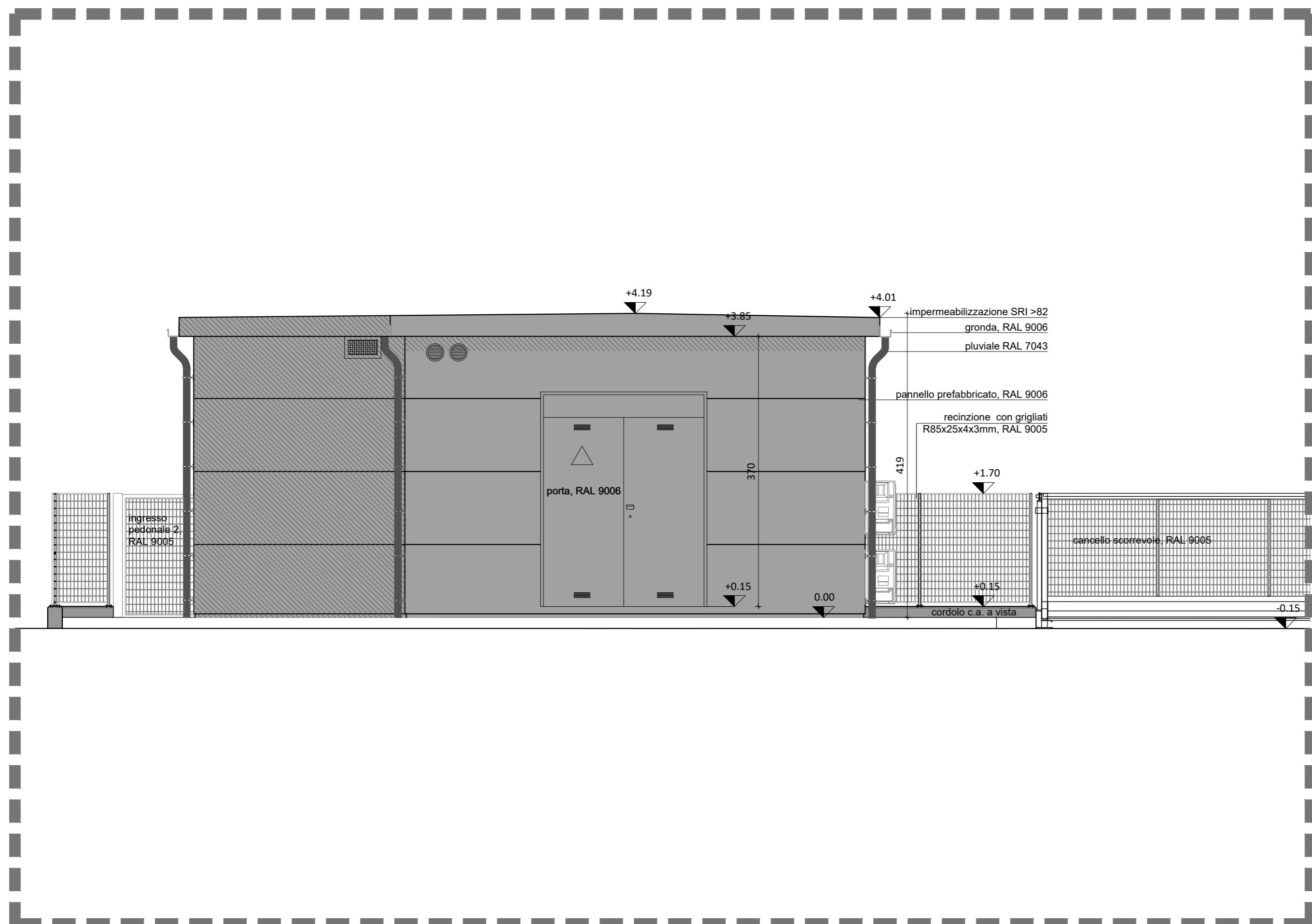
Prospetto sud
