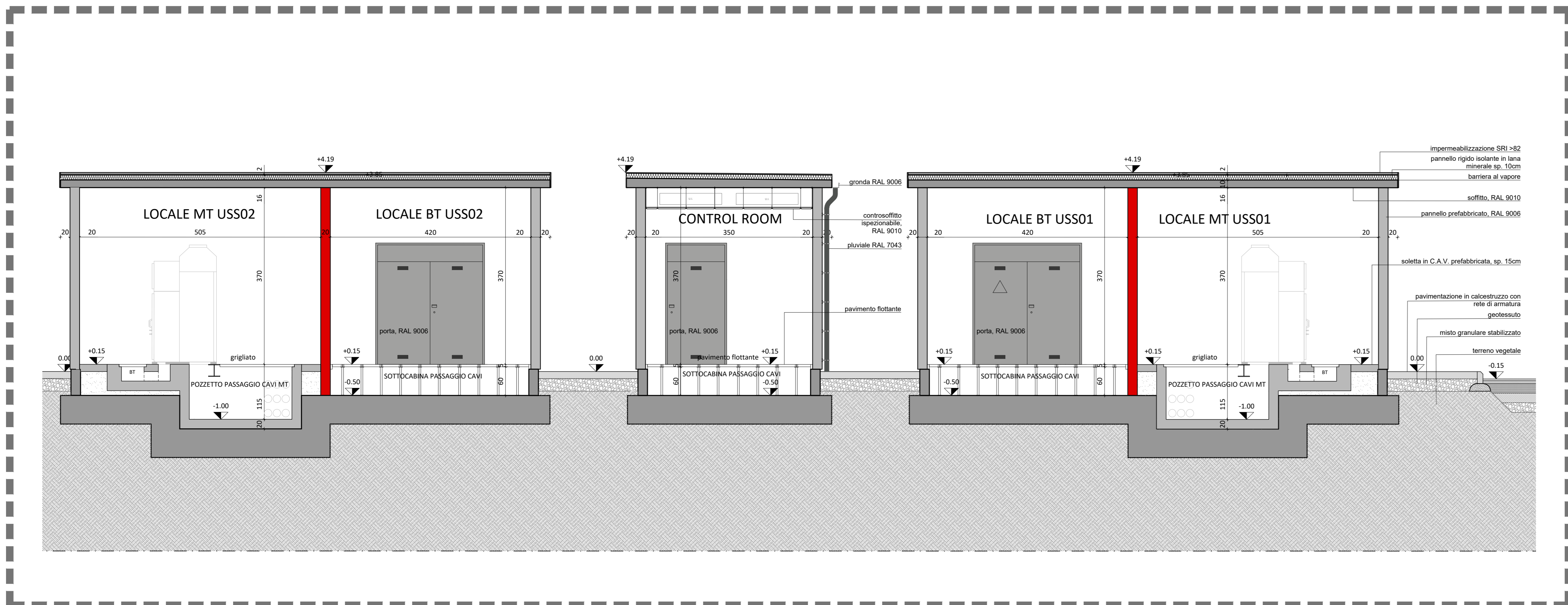
Sezione A - A
