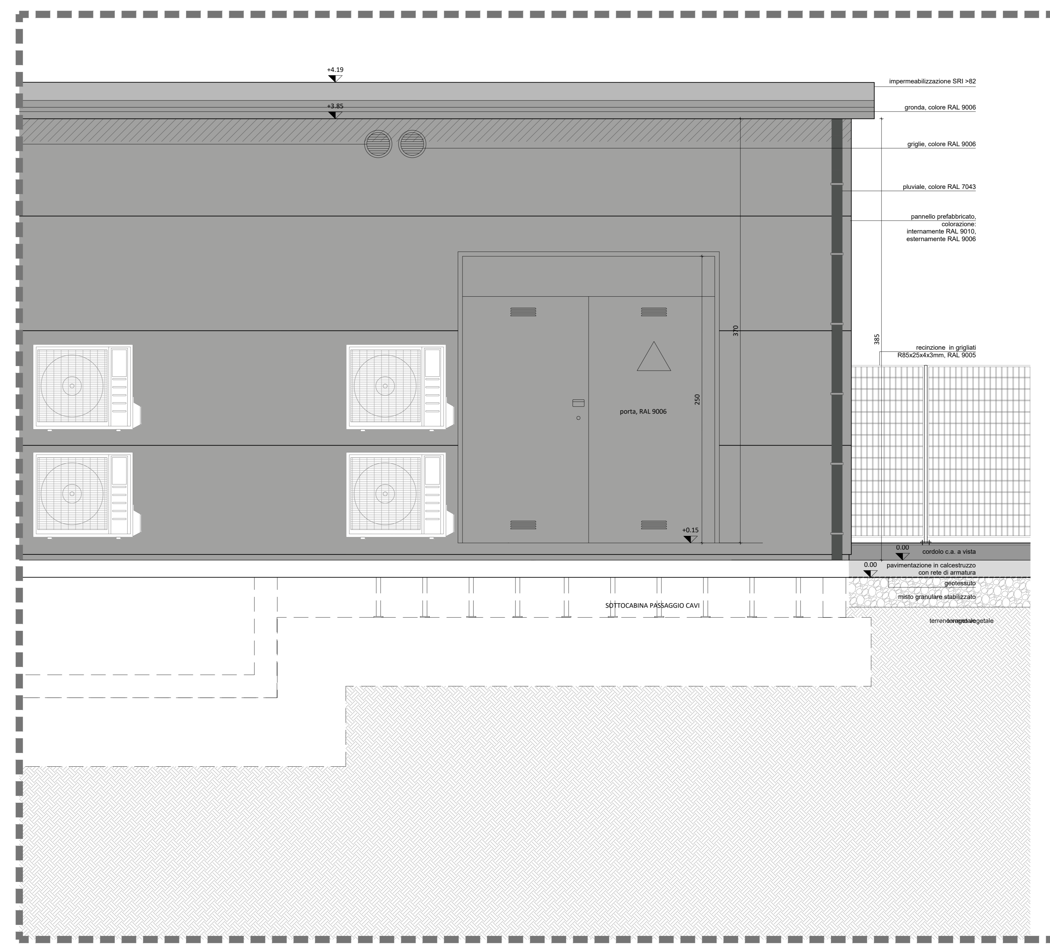
Particolare di facciata LOCALE BT USS 01 scala 1:20
