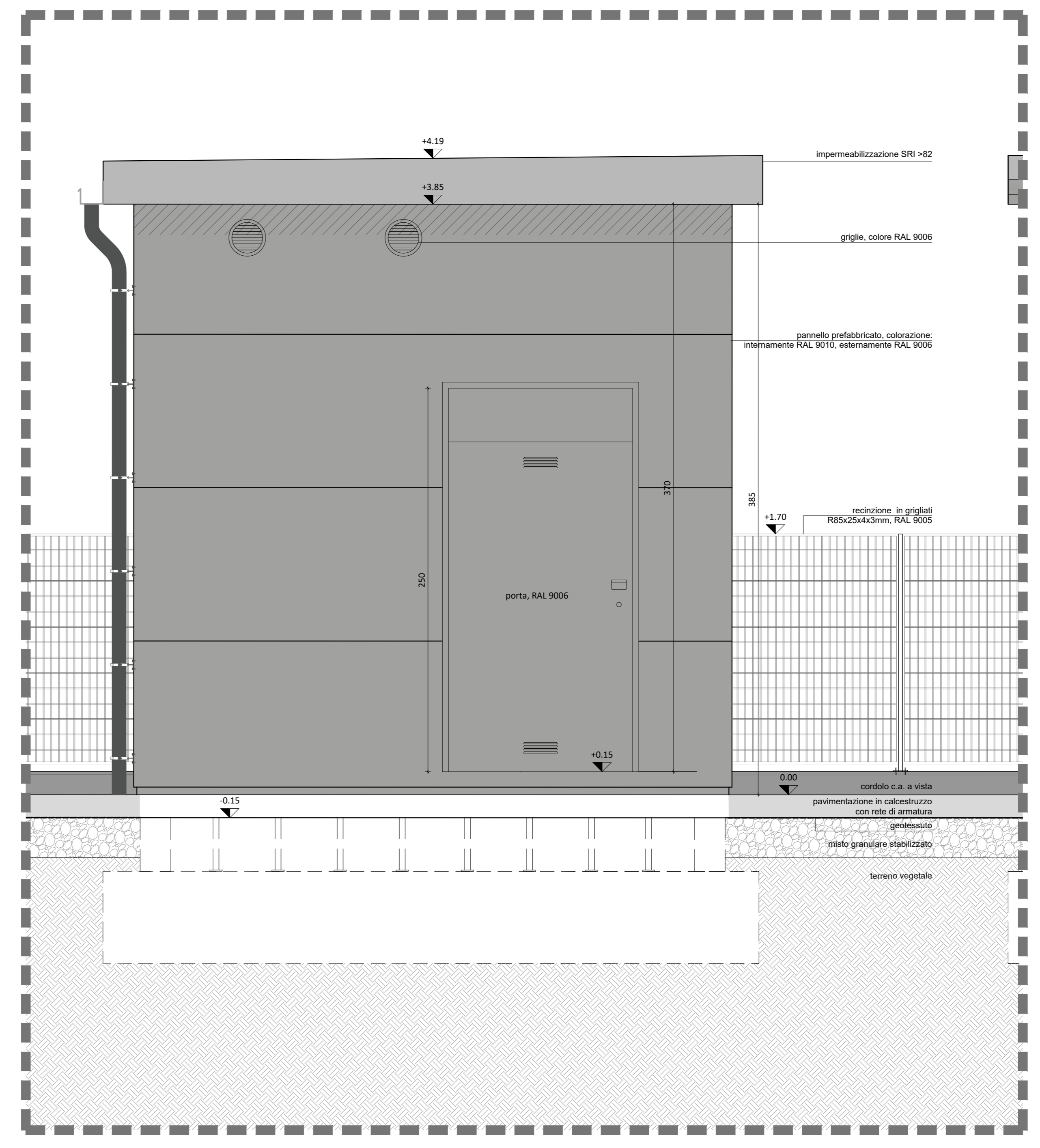
Particolare di facciata Control Room scala 1:20
