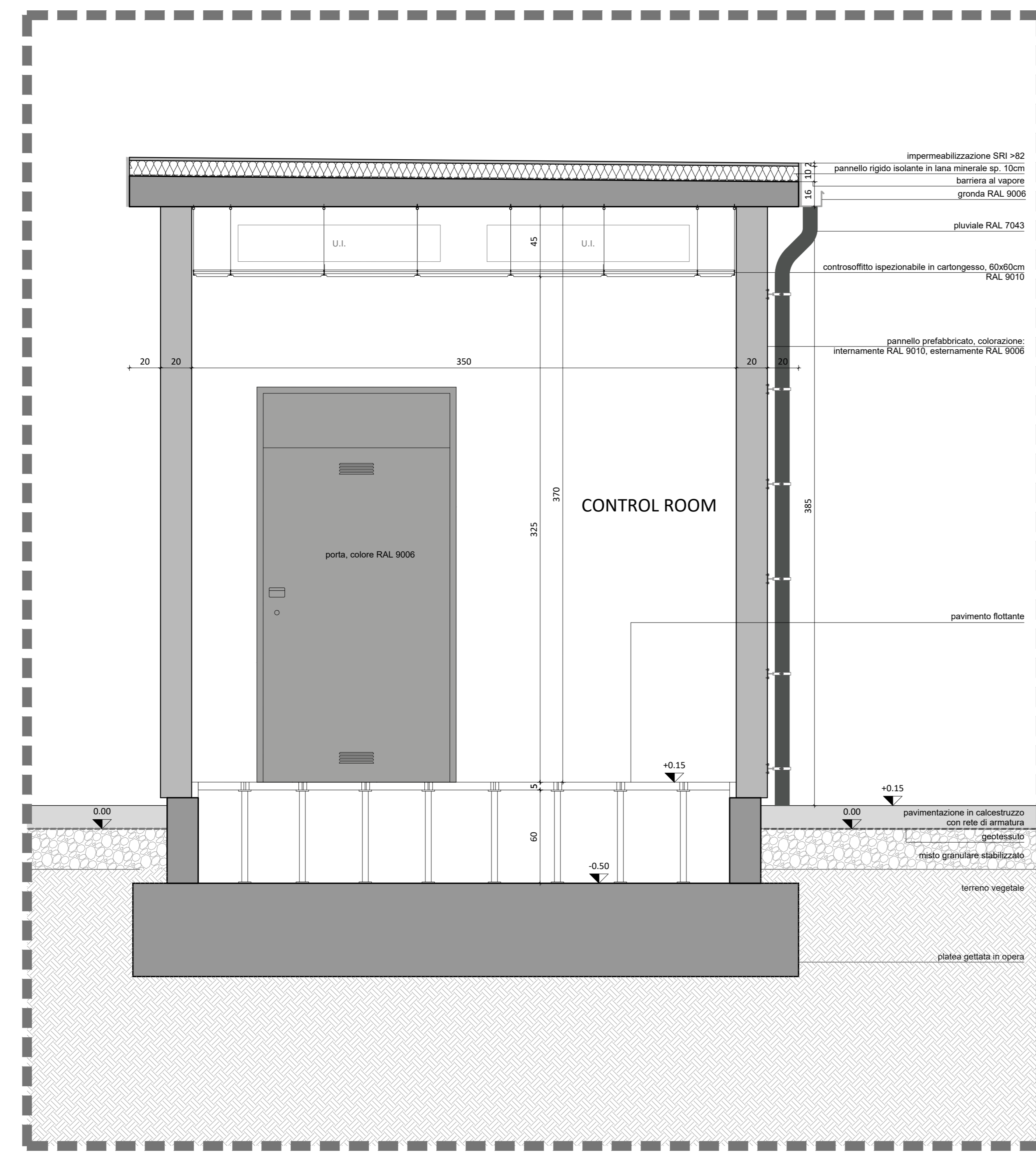
Sezione Control Room scala 1:20
