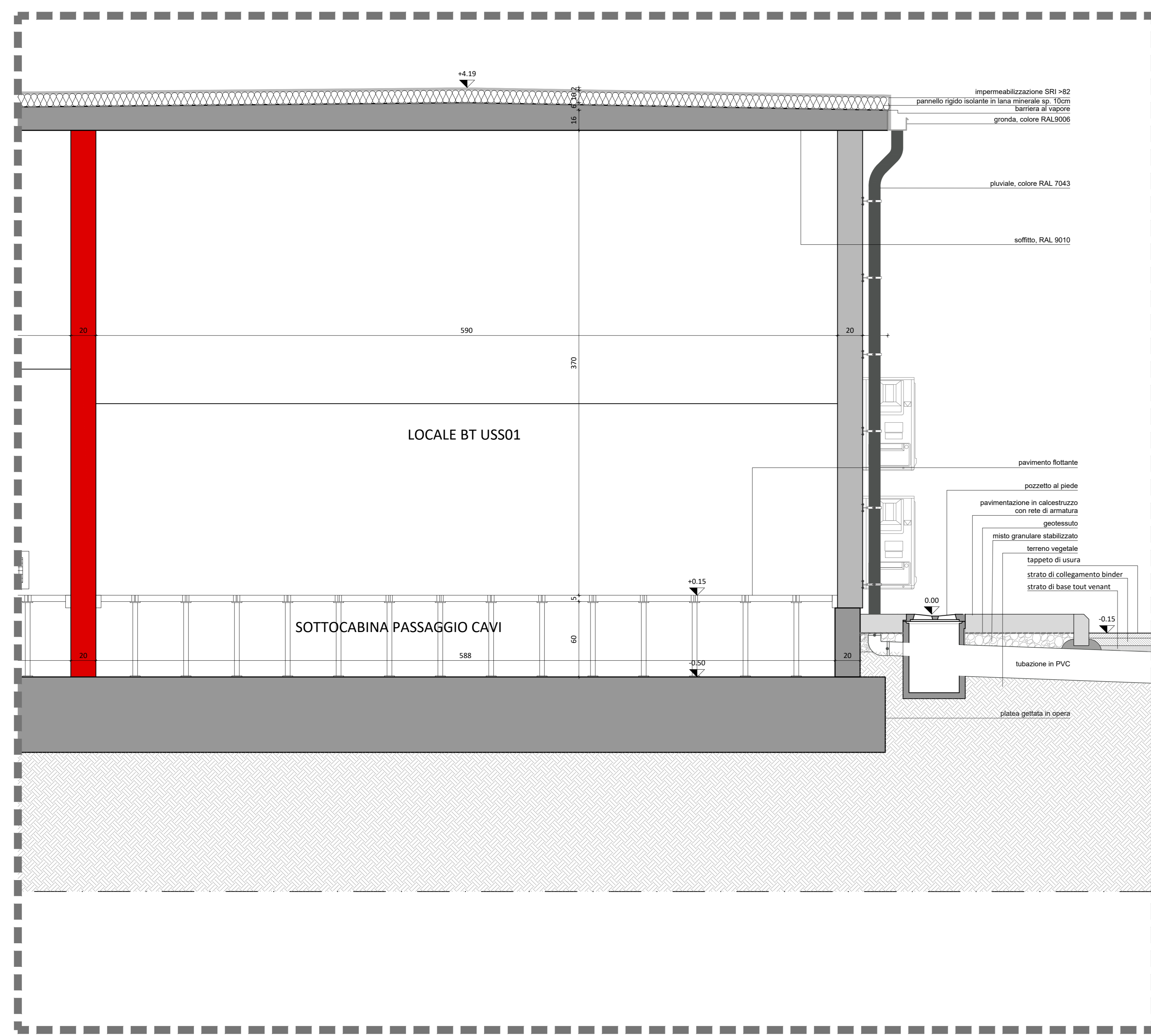
Sezione LOCALE BT USS 01 scala 1:20
