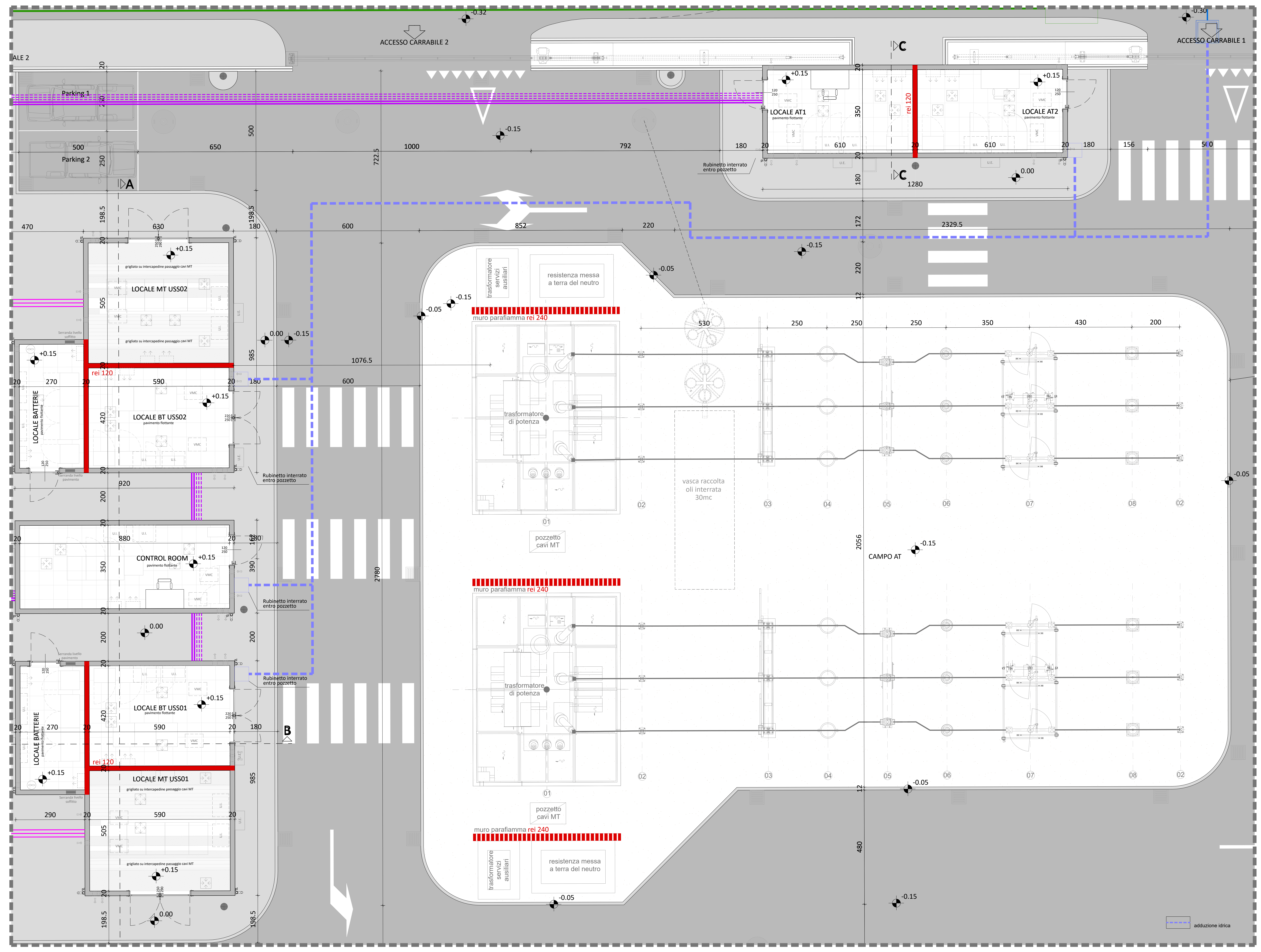
Planimetria impianto acqua potabile
